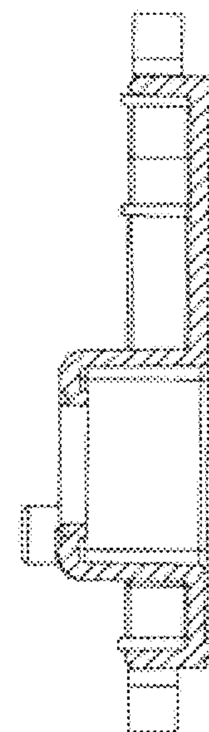
SECTION A-A
