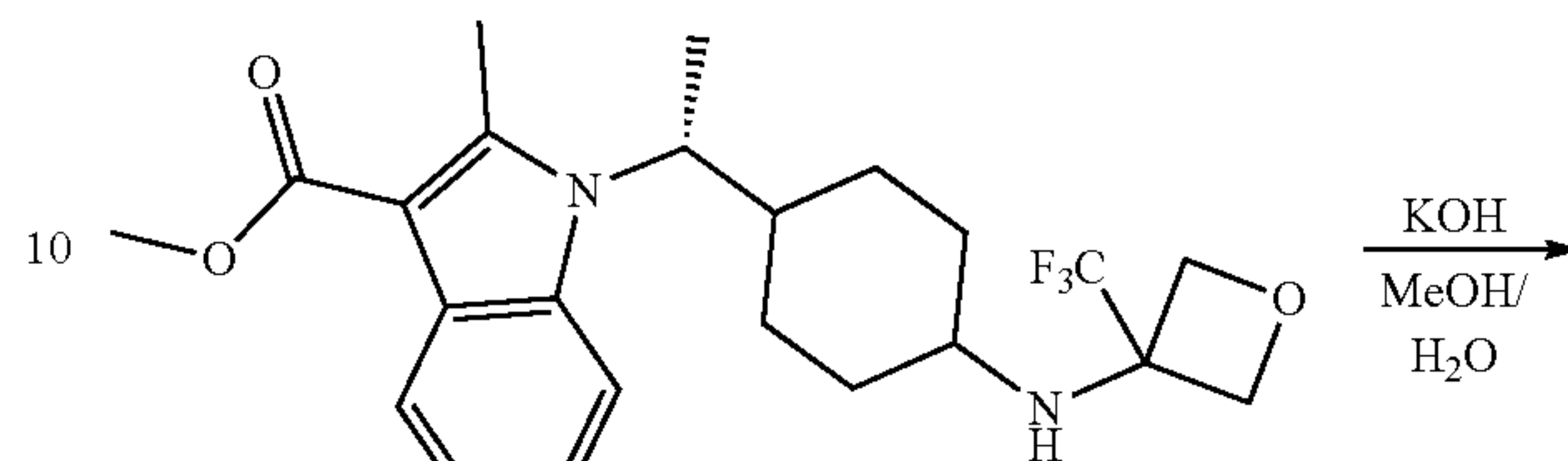
M3
