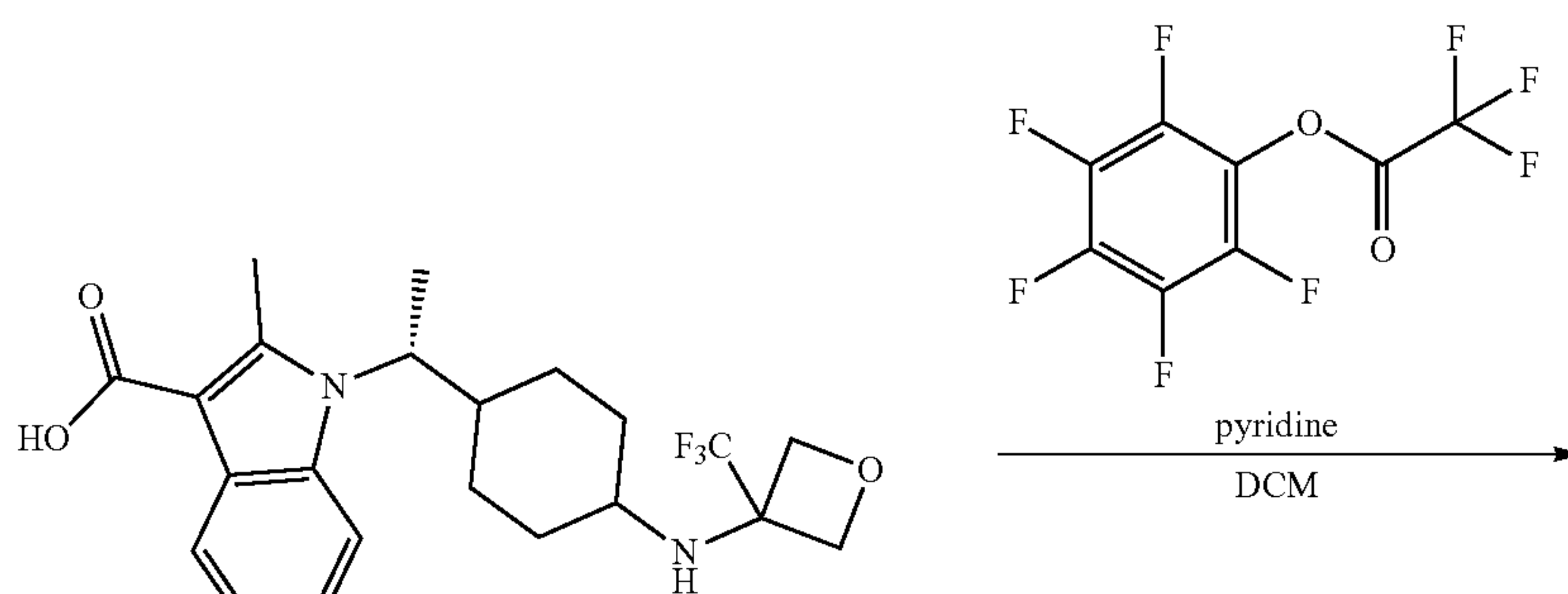
M4
