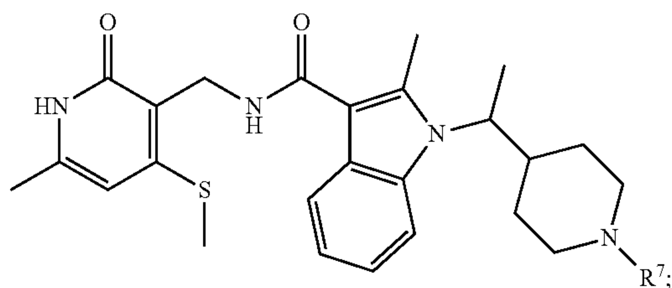
(XXII)
