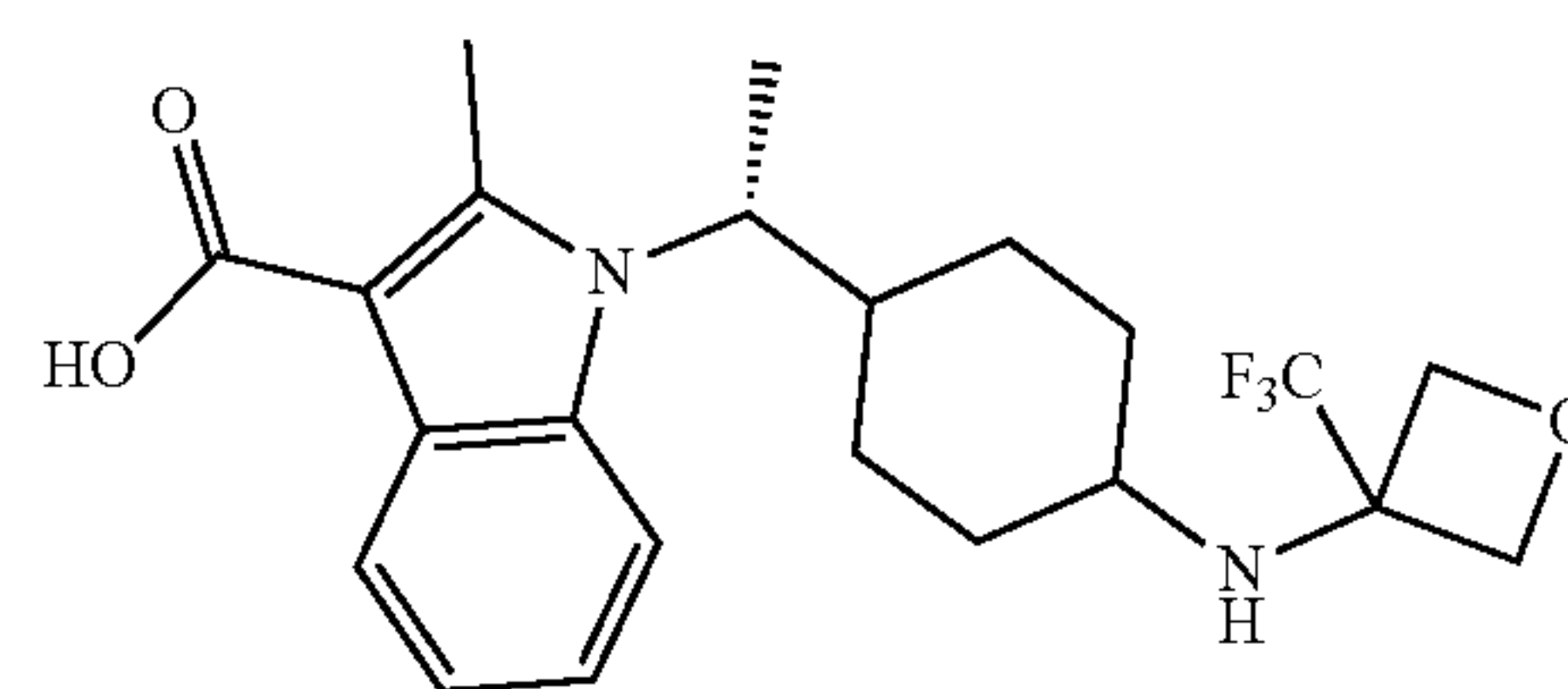
M4
