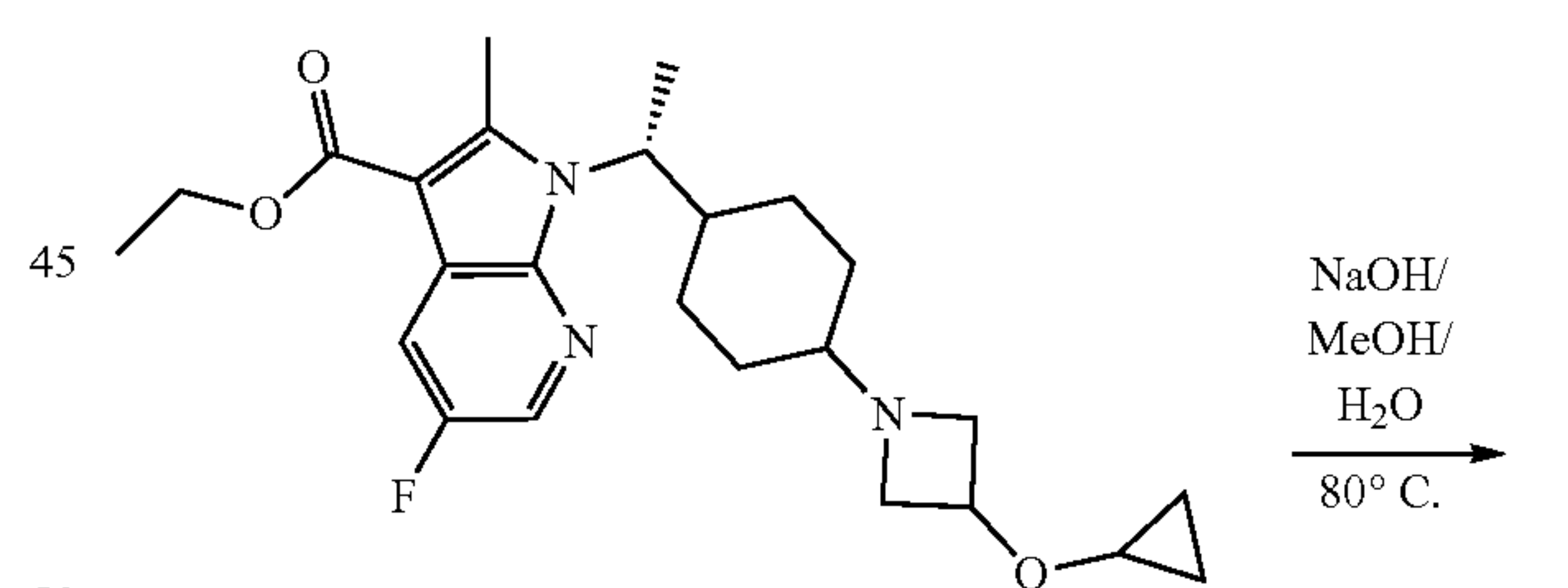
J8 isomer 2
