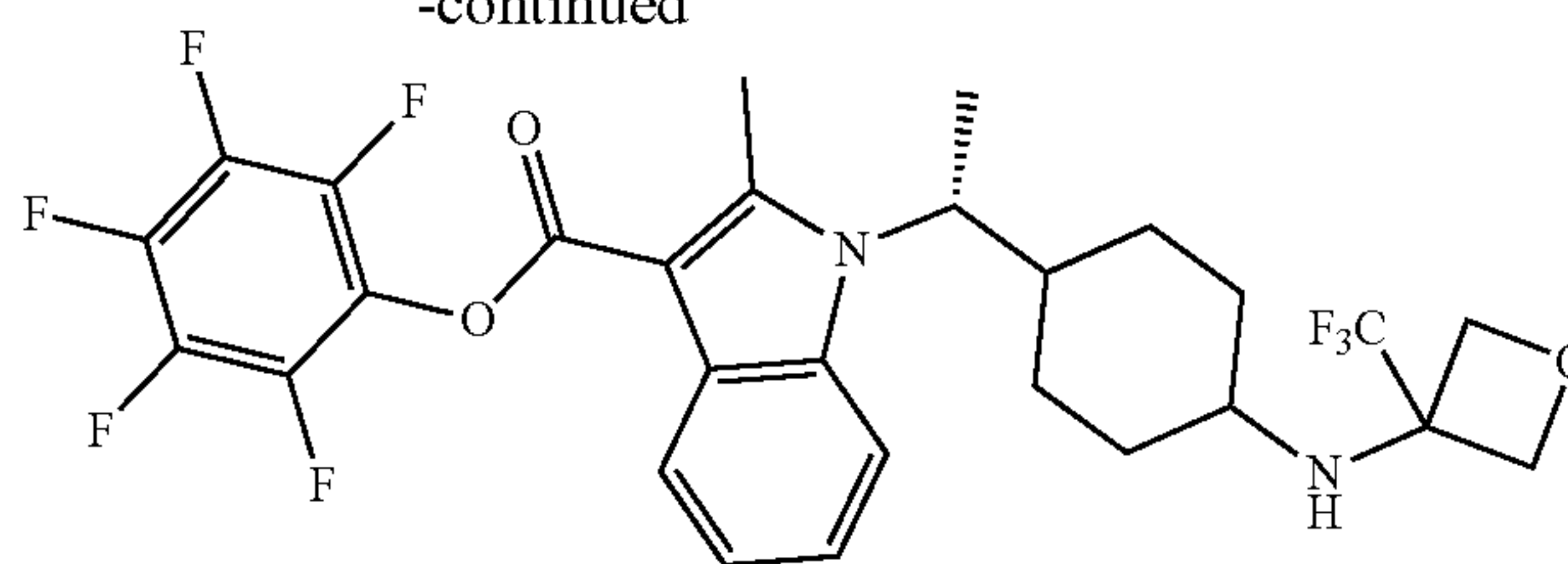
M5
