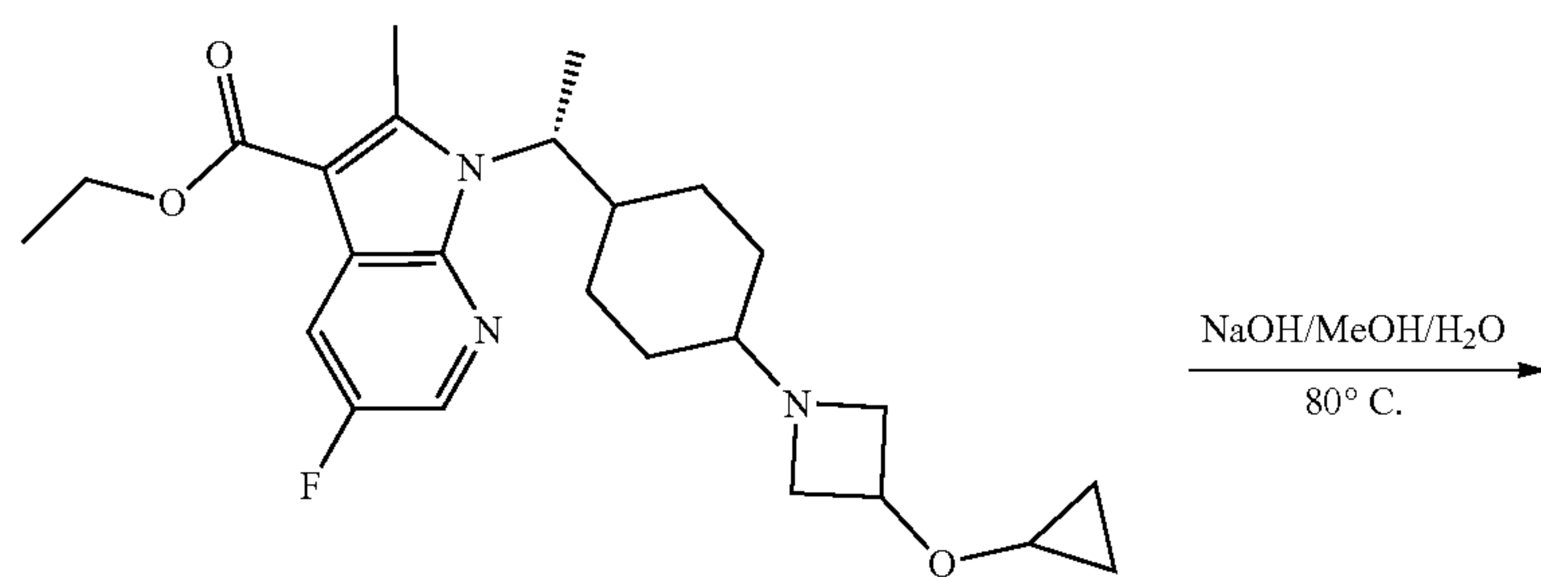
J8 isomer 2
