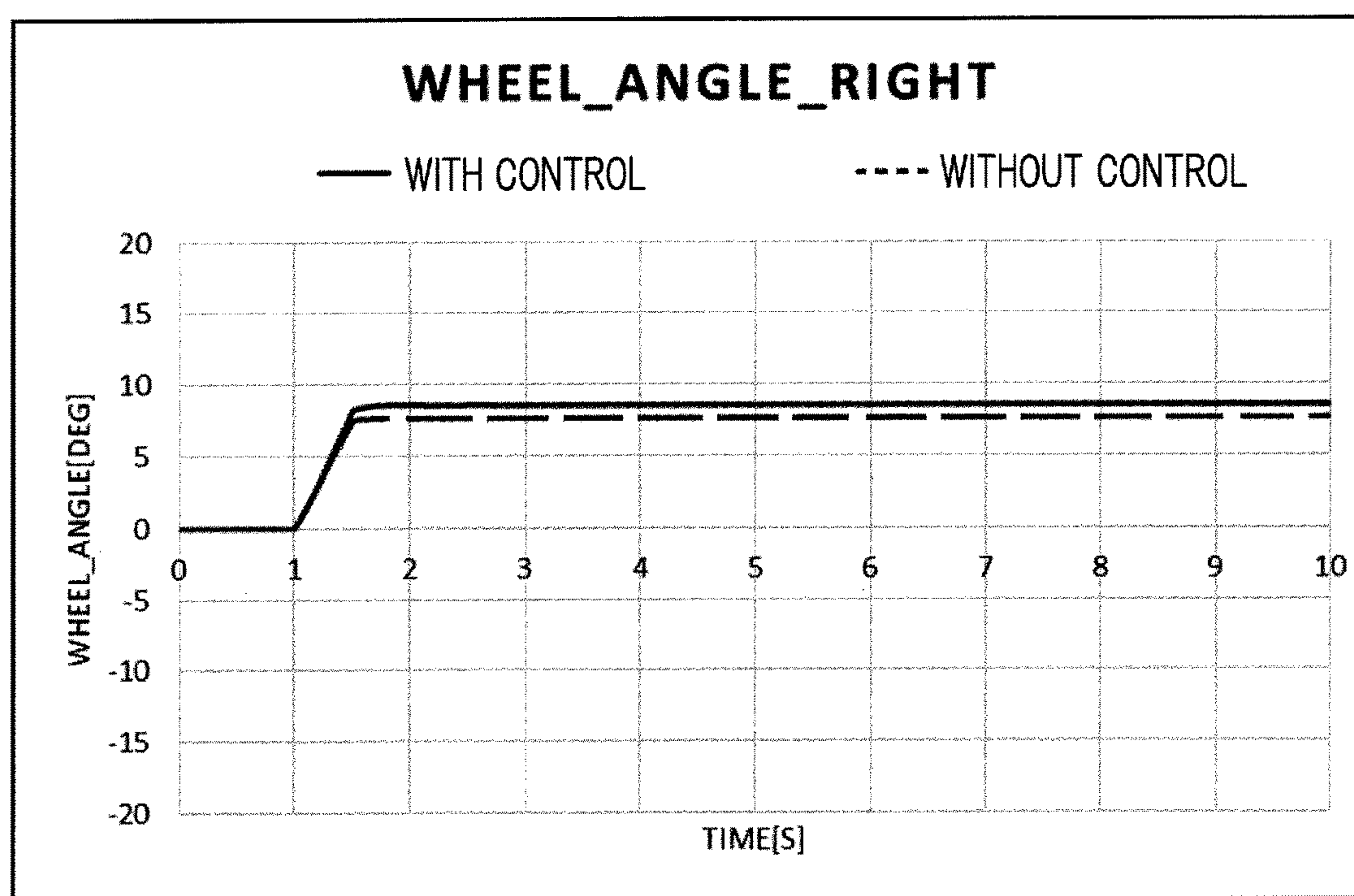
(d) RIGHT WHEEL ANGLE
