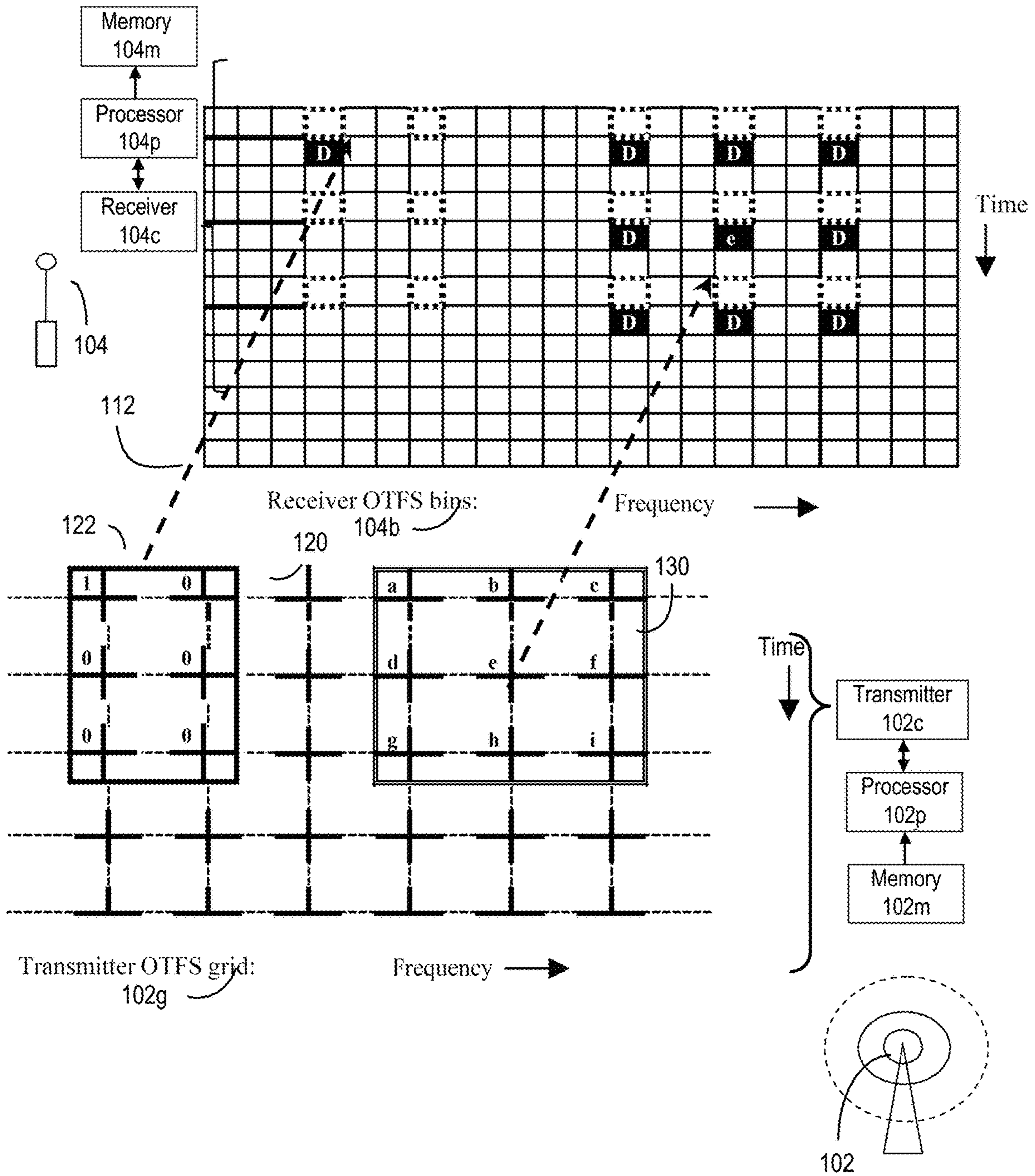
FIG. 17B
