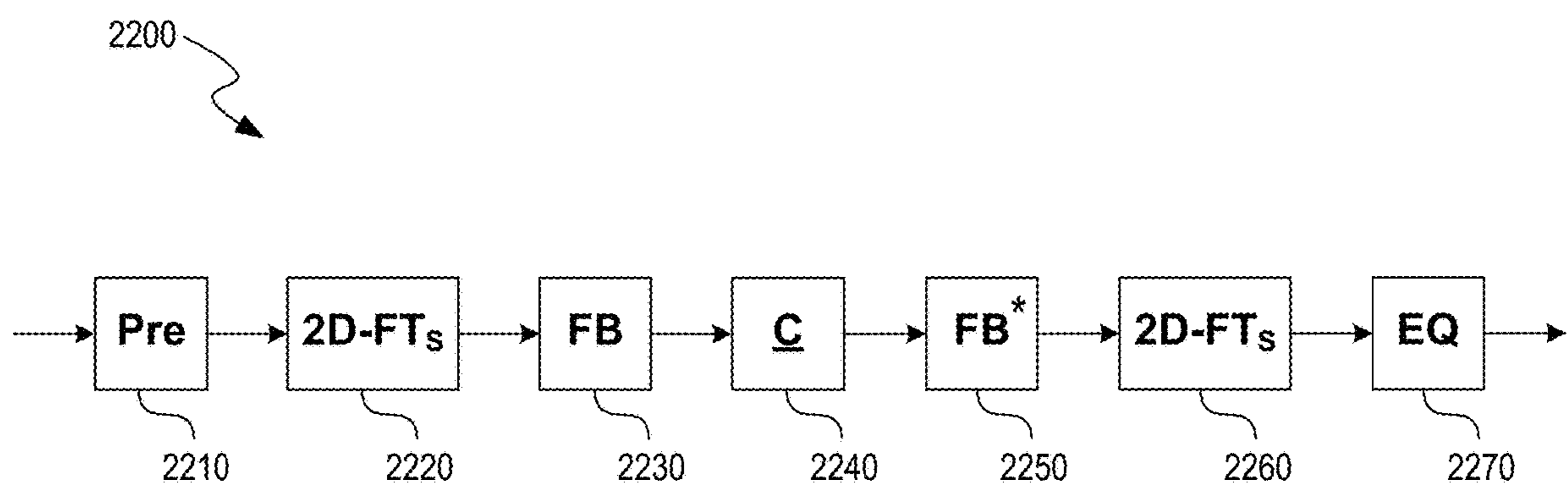
FIG. 22
