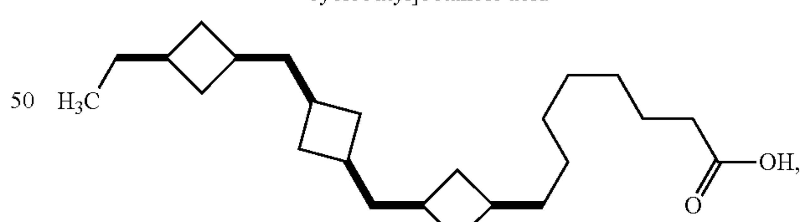
8-[3-(3-Pentyl)-cyclobutylmethyl]-cyclobutyl]octanoic acid
