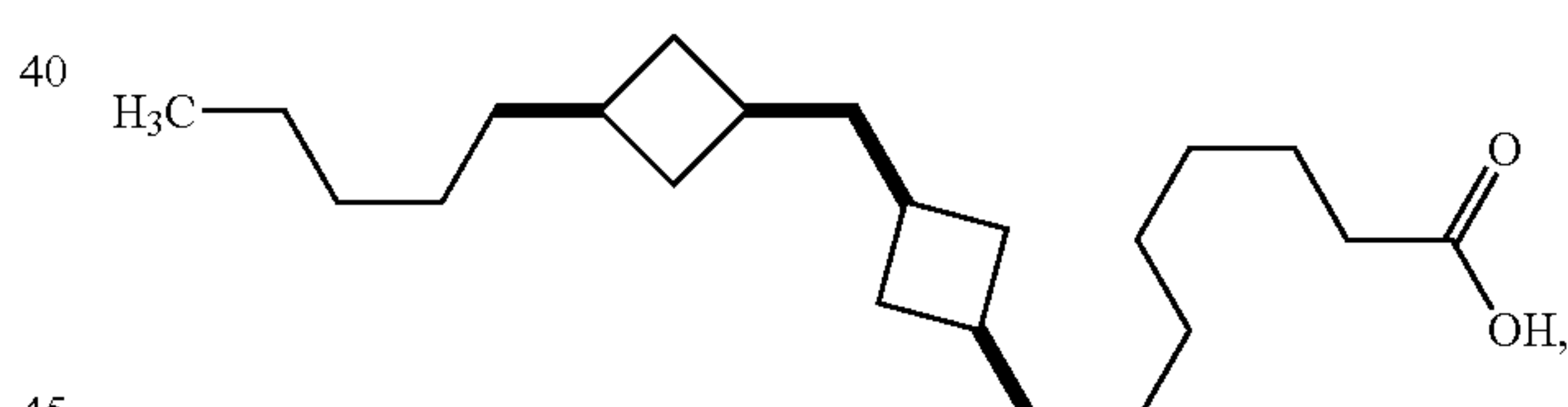
8-[3-(3-Pentyl)-cyclobutylmethyl]-cyclobutyl]octanoic acid
