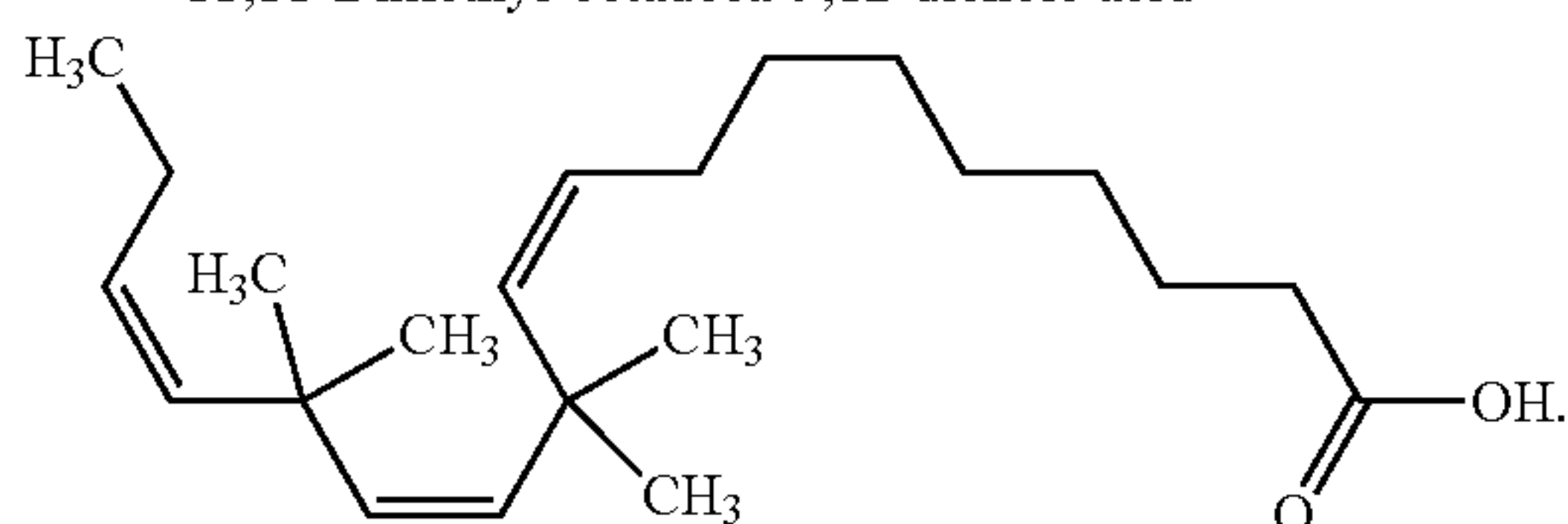
11,11,14,14-Tetramethyl-octadeca-9,12,15-trienoic acid
