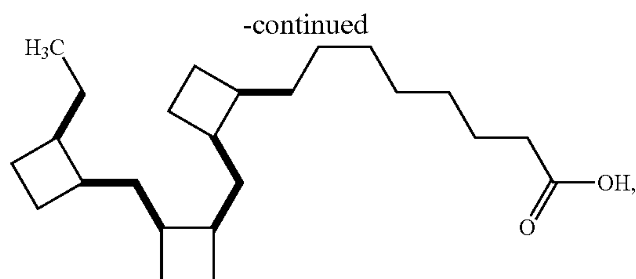
8-{2-[2-(2-Ethyl-cyclobutylmethyl)-cyclobutyl]-cyclobutyl}-octanoic acid
