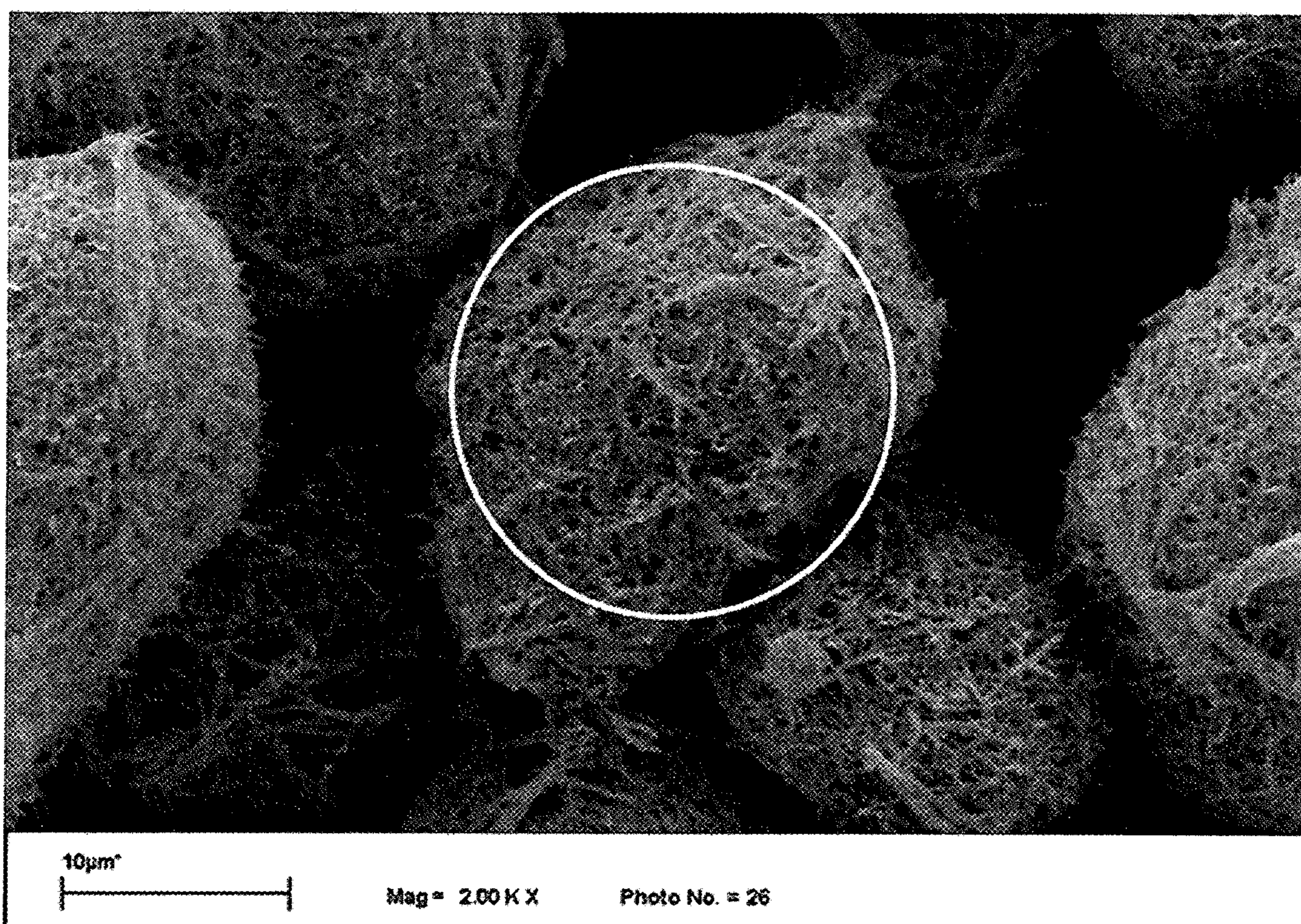
SEM of Crystalline Xonotlite (CSH)
