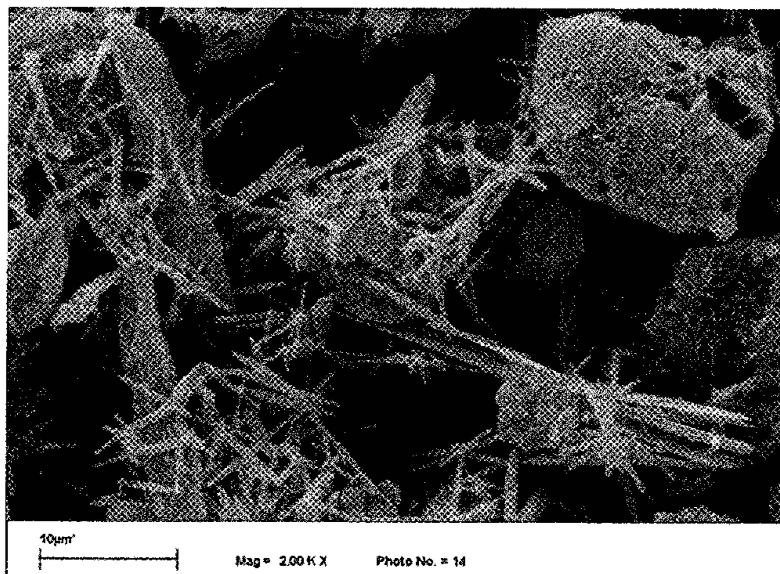
SEM of Nano-Composite (SAS & FCA)
