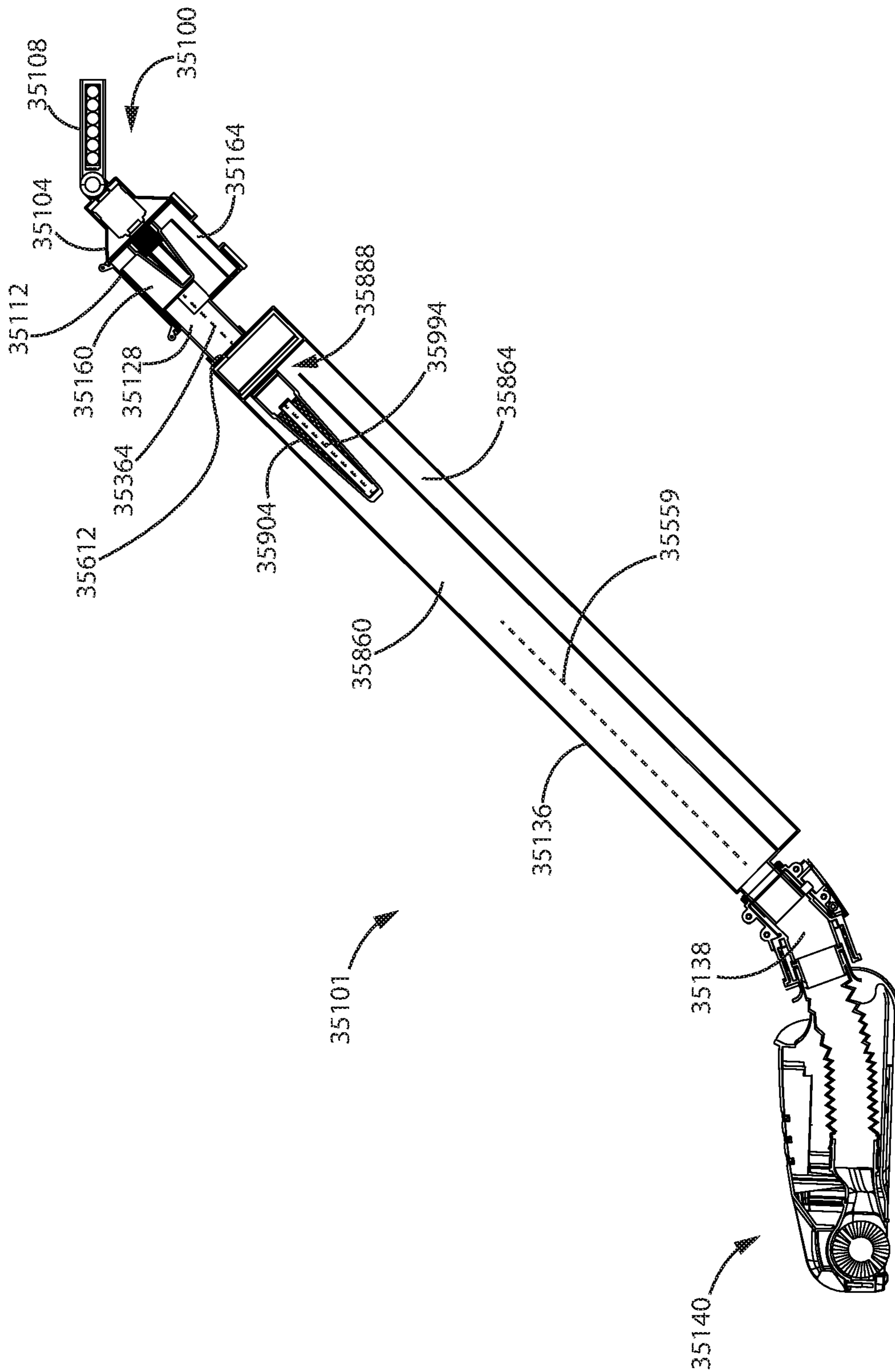
FIG. 81
