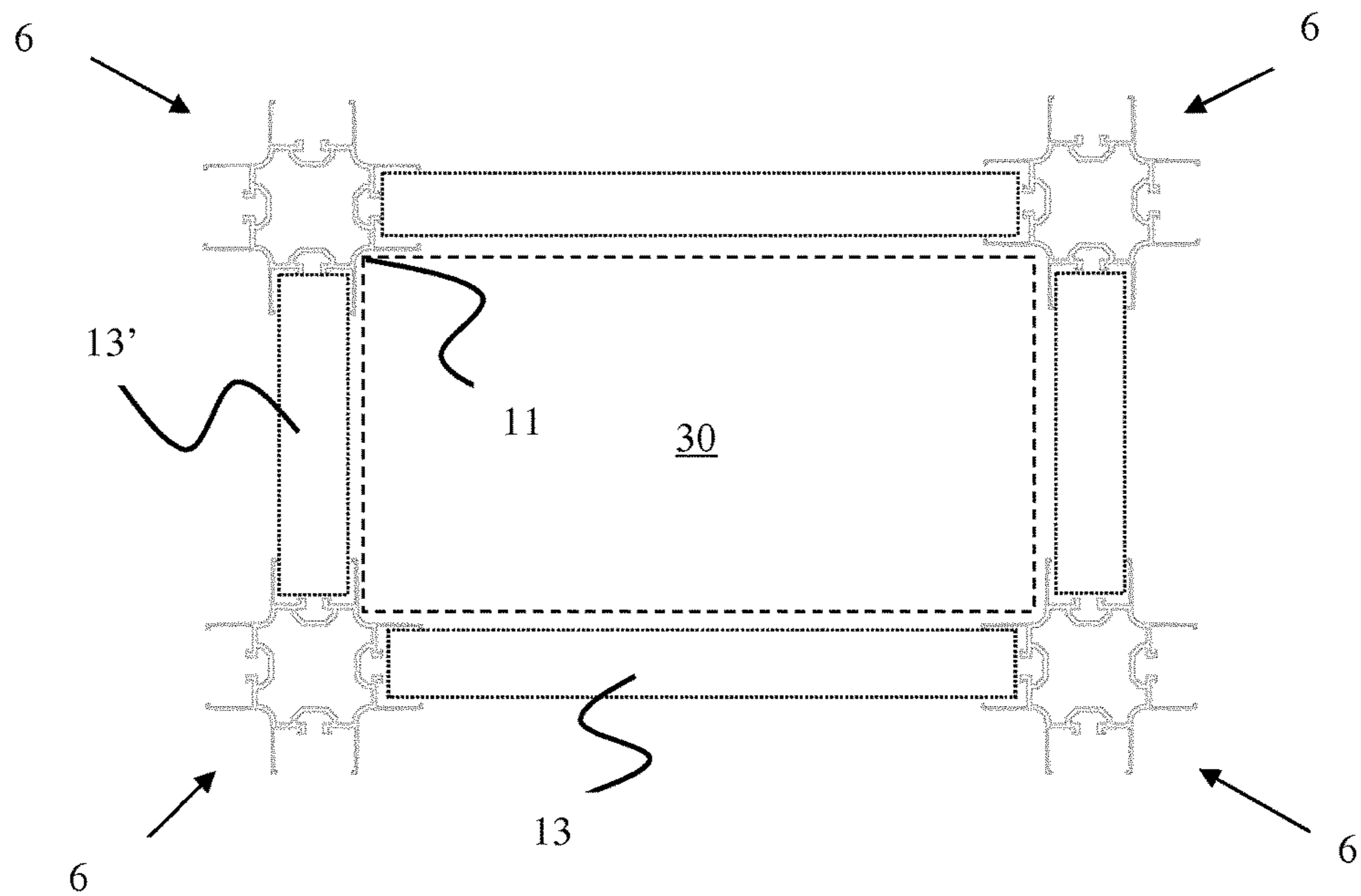
Fig. 14 (C-C)
