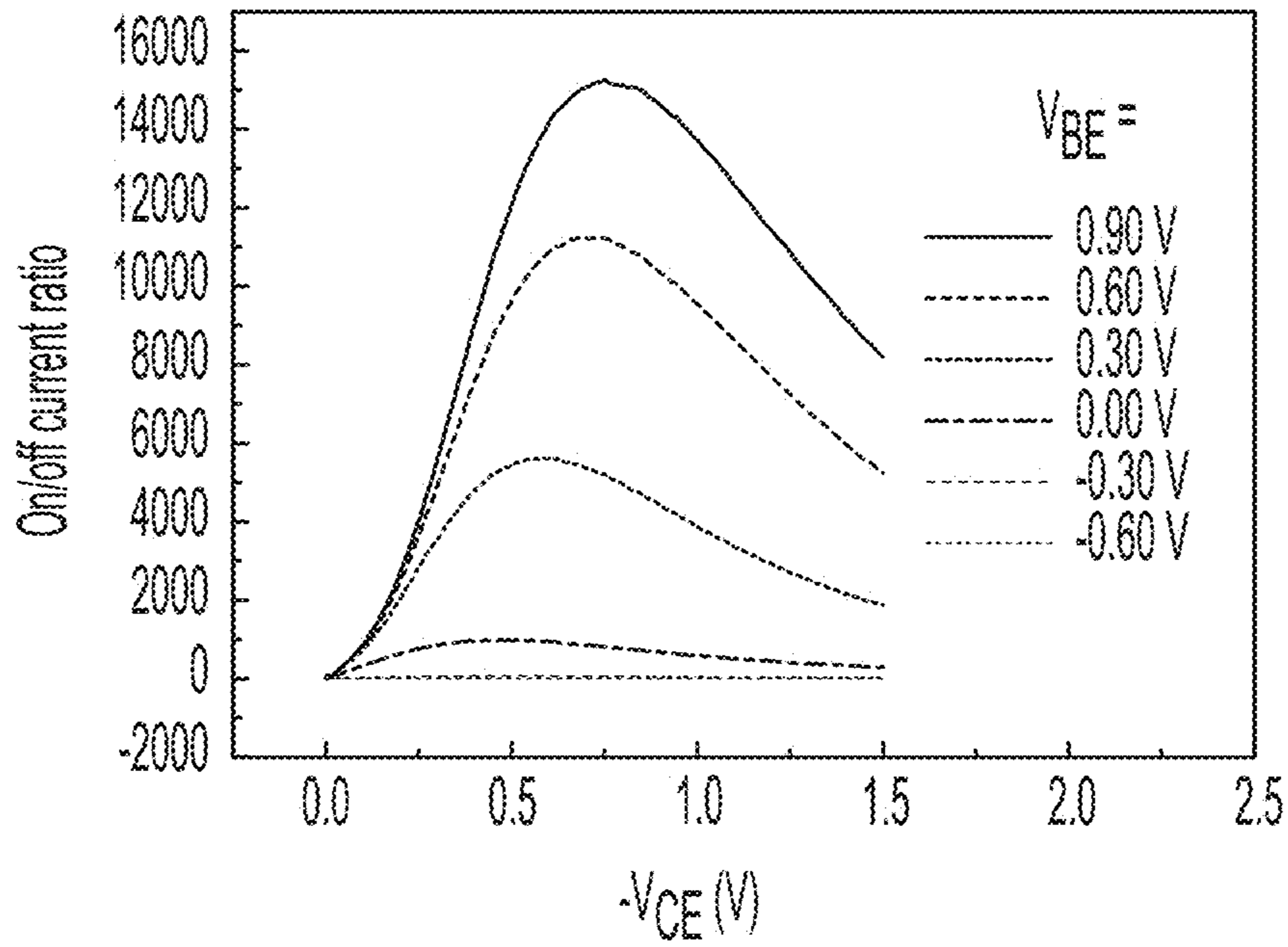
FIG. 5B
