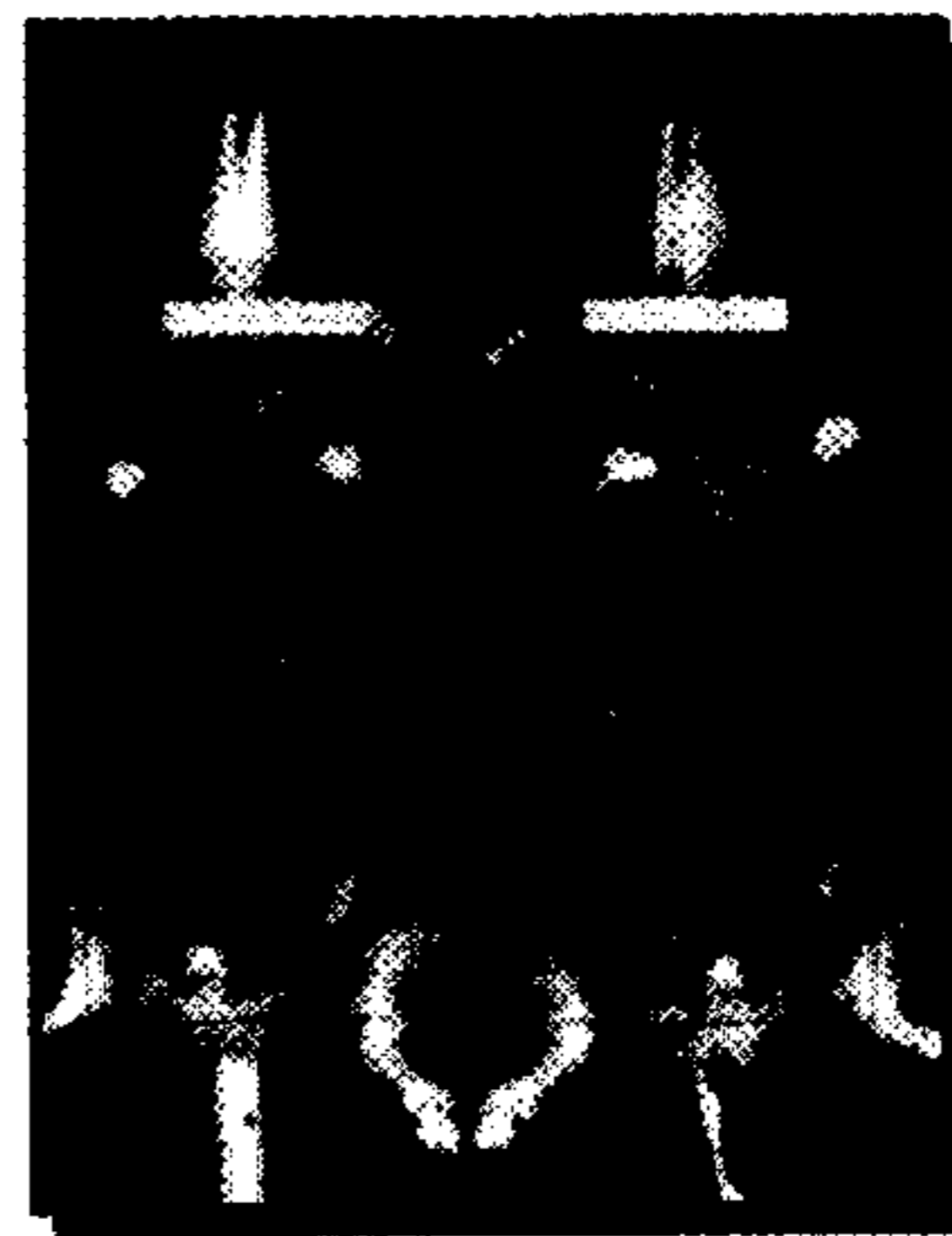
WT-AAV2
