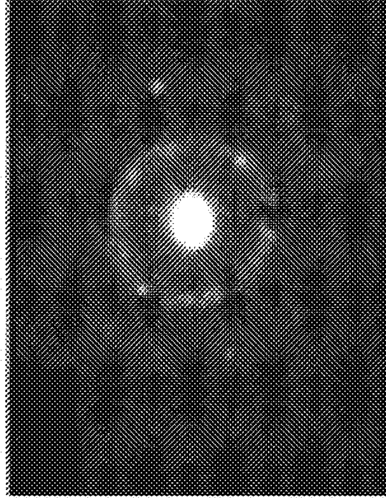
nc-OS
