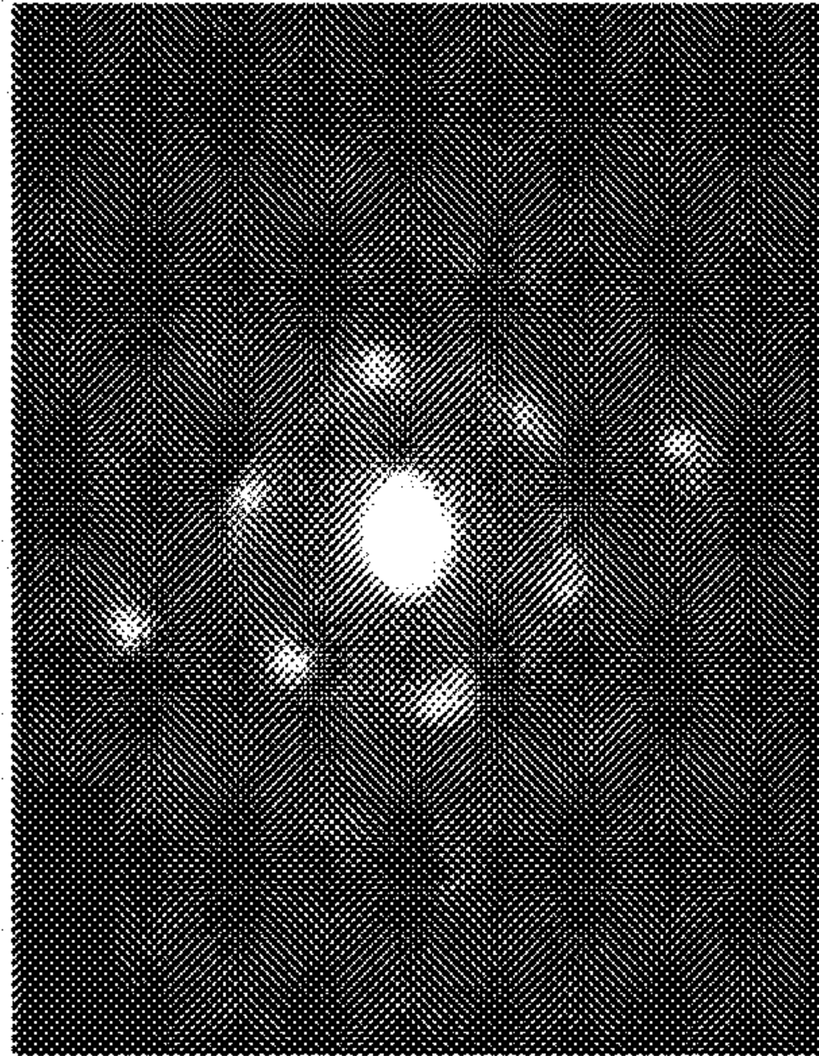
CAAC-OS
