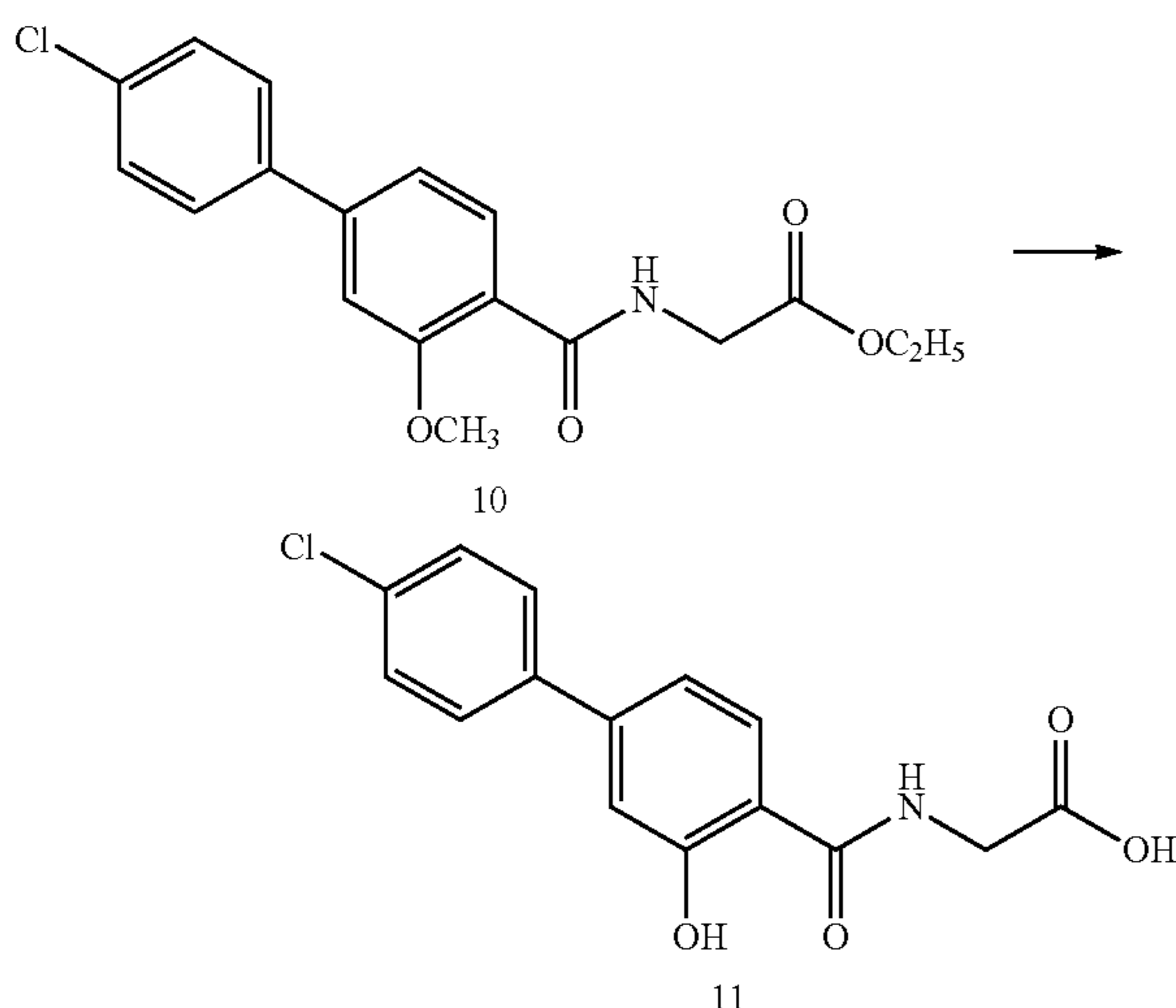
Scheme VI
