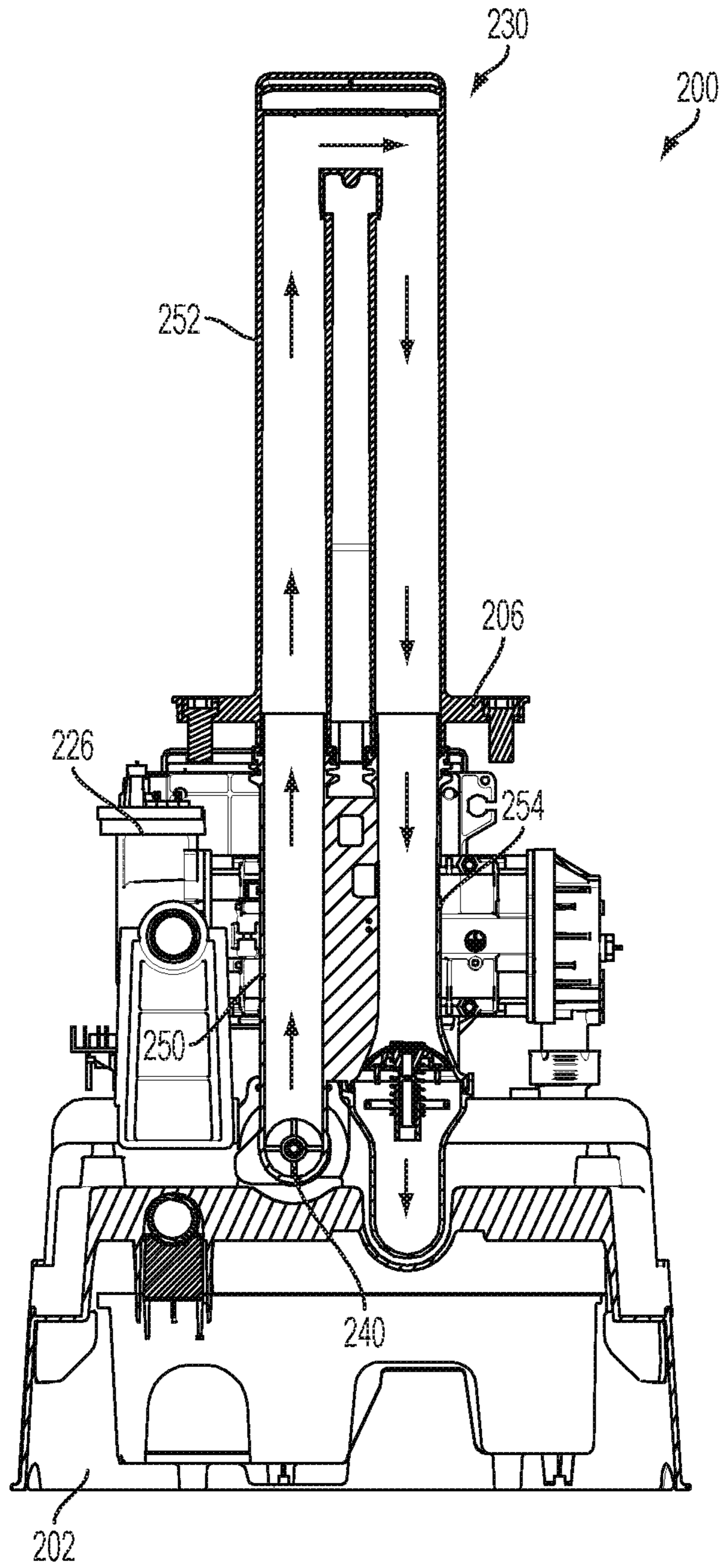
FIG. 14
