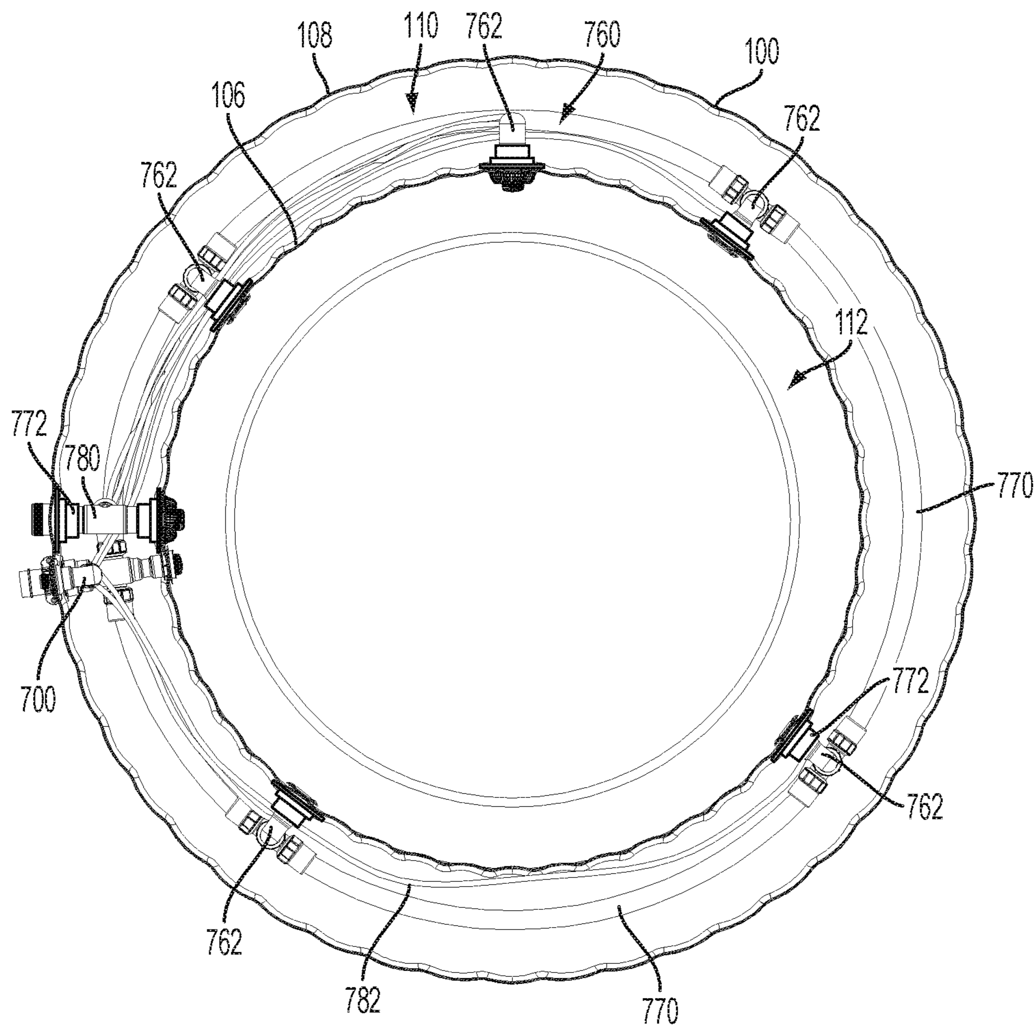
FIG. 41
