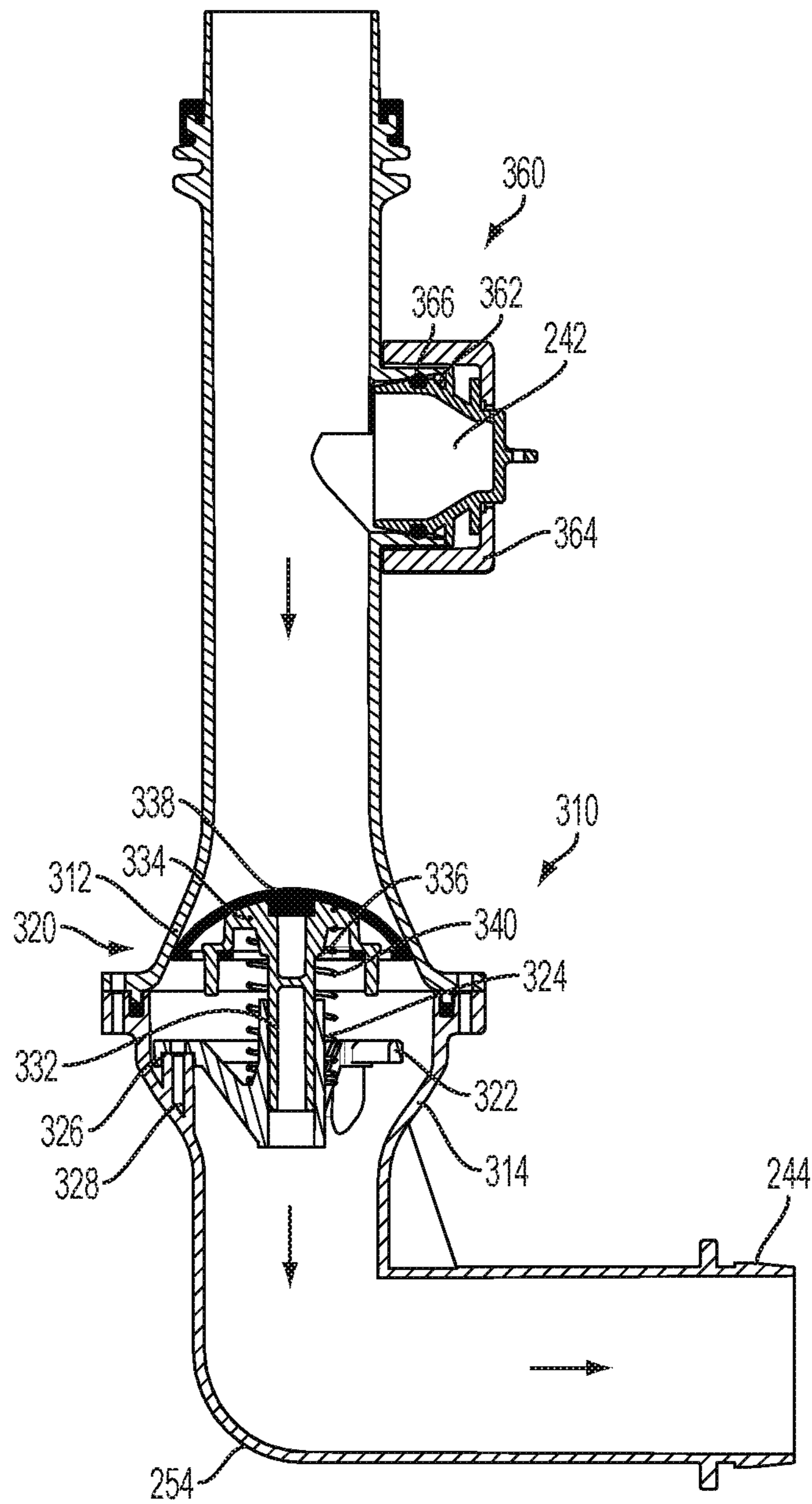
FIG. 20
