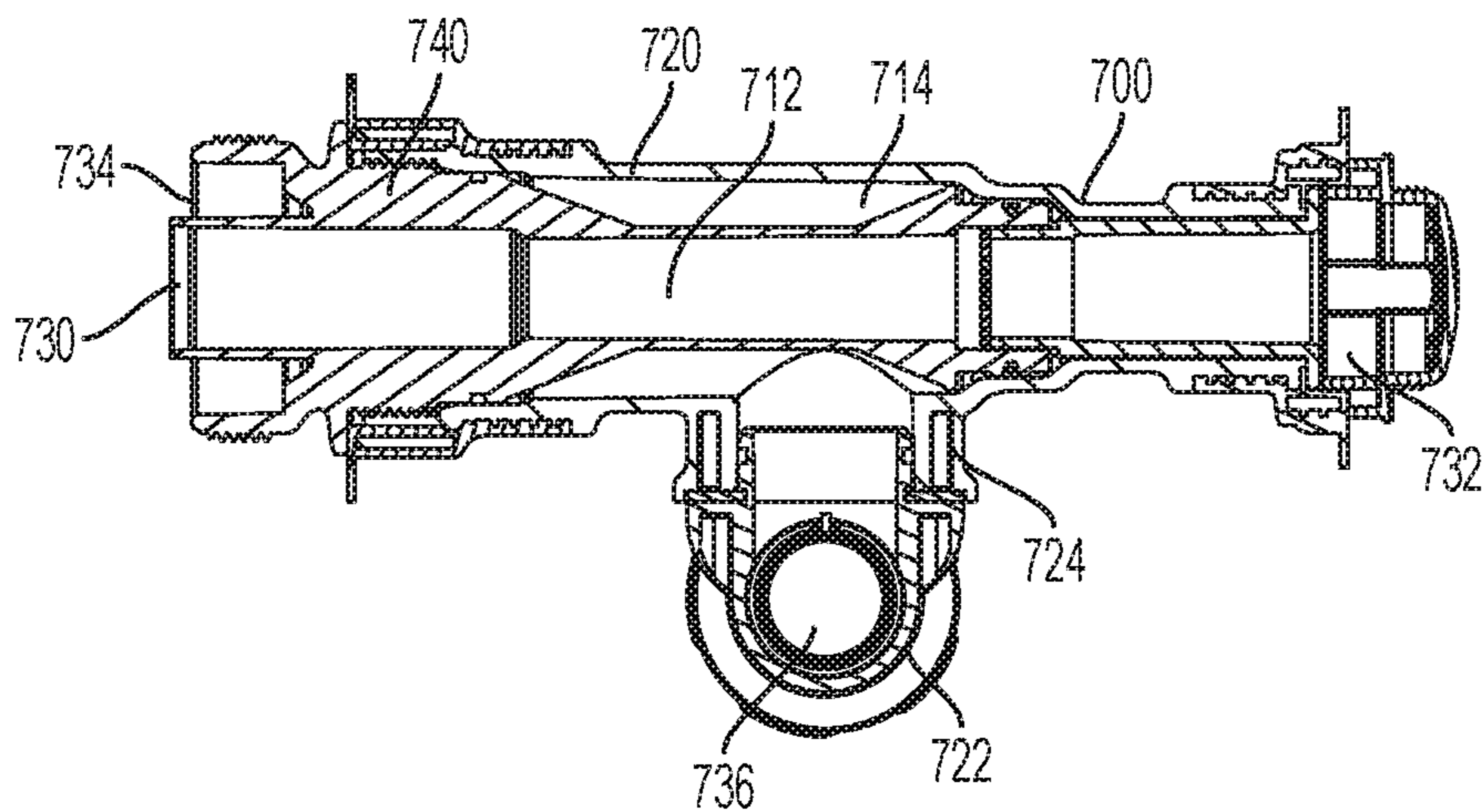
FIG. 38
