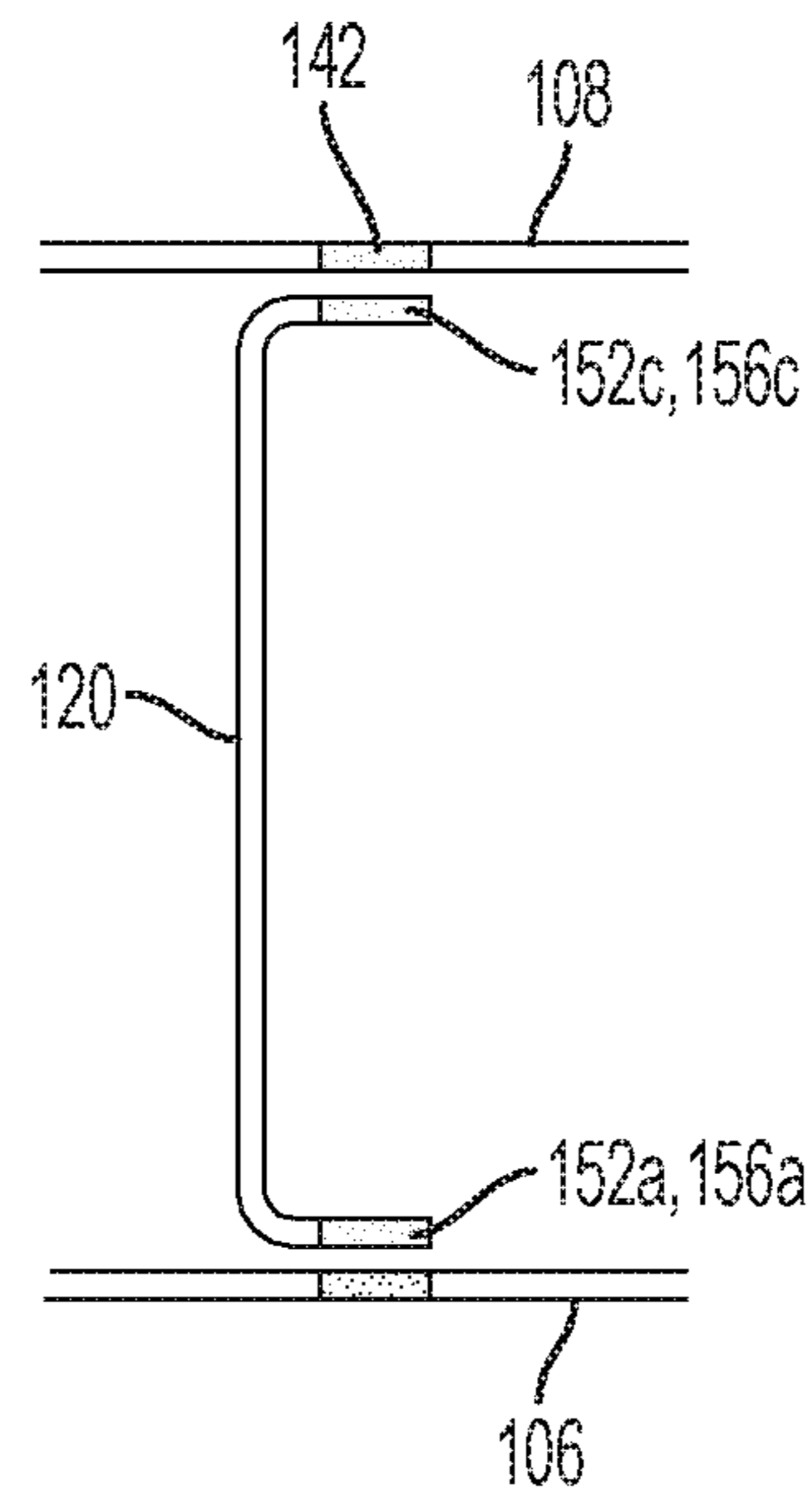
FIG. 7
