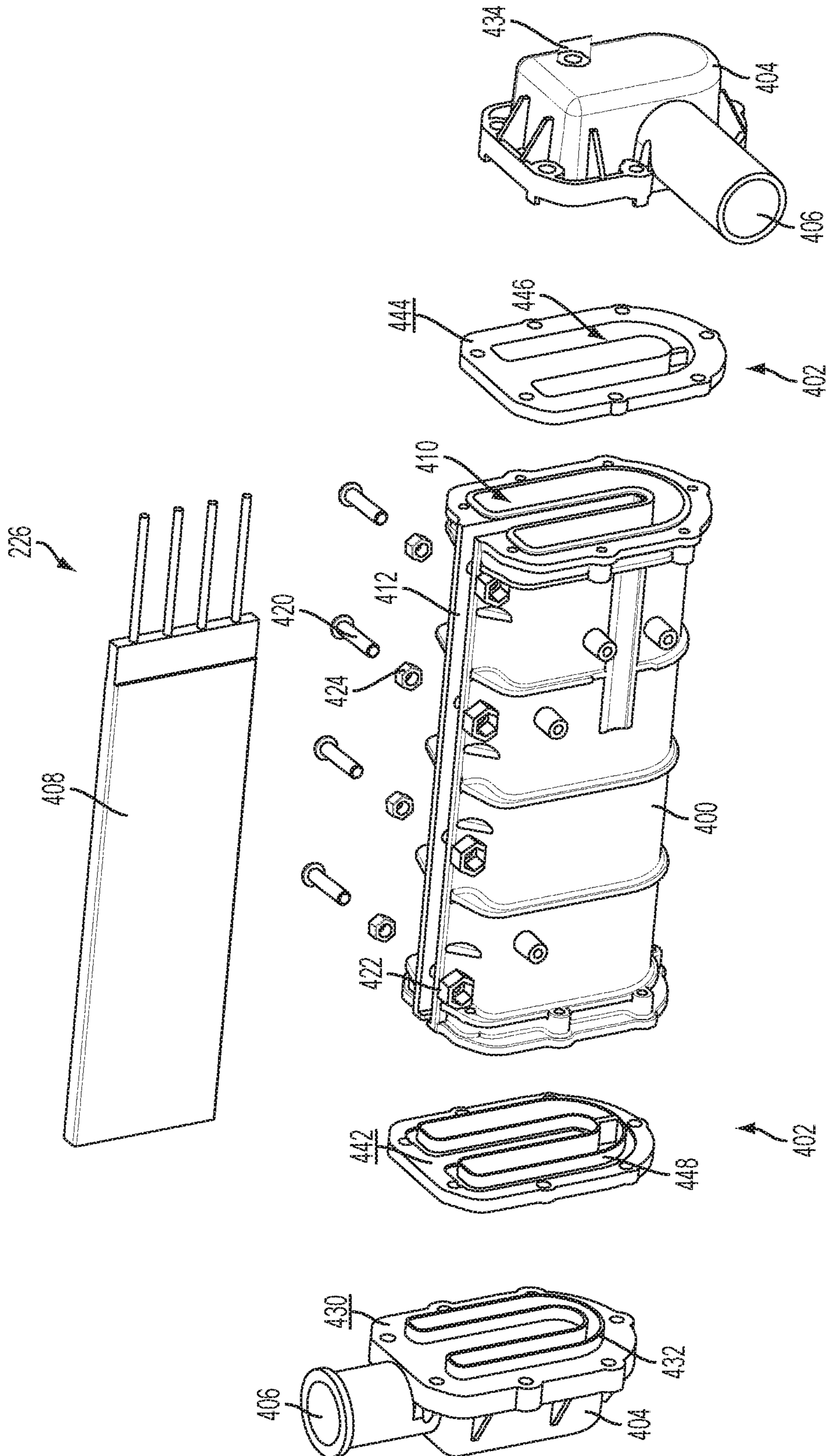
FIG. 25
