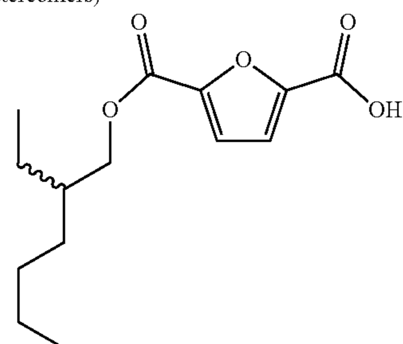
FDM(2EH) (Enantiomers)
