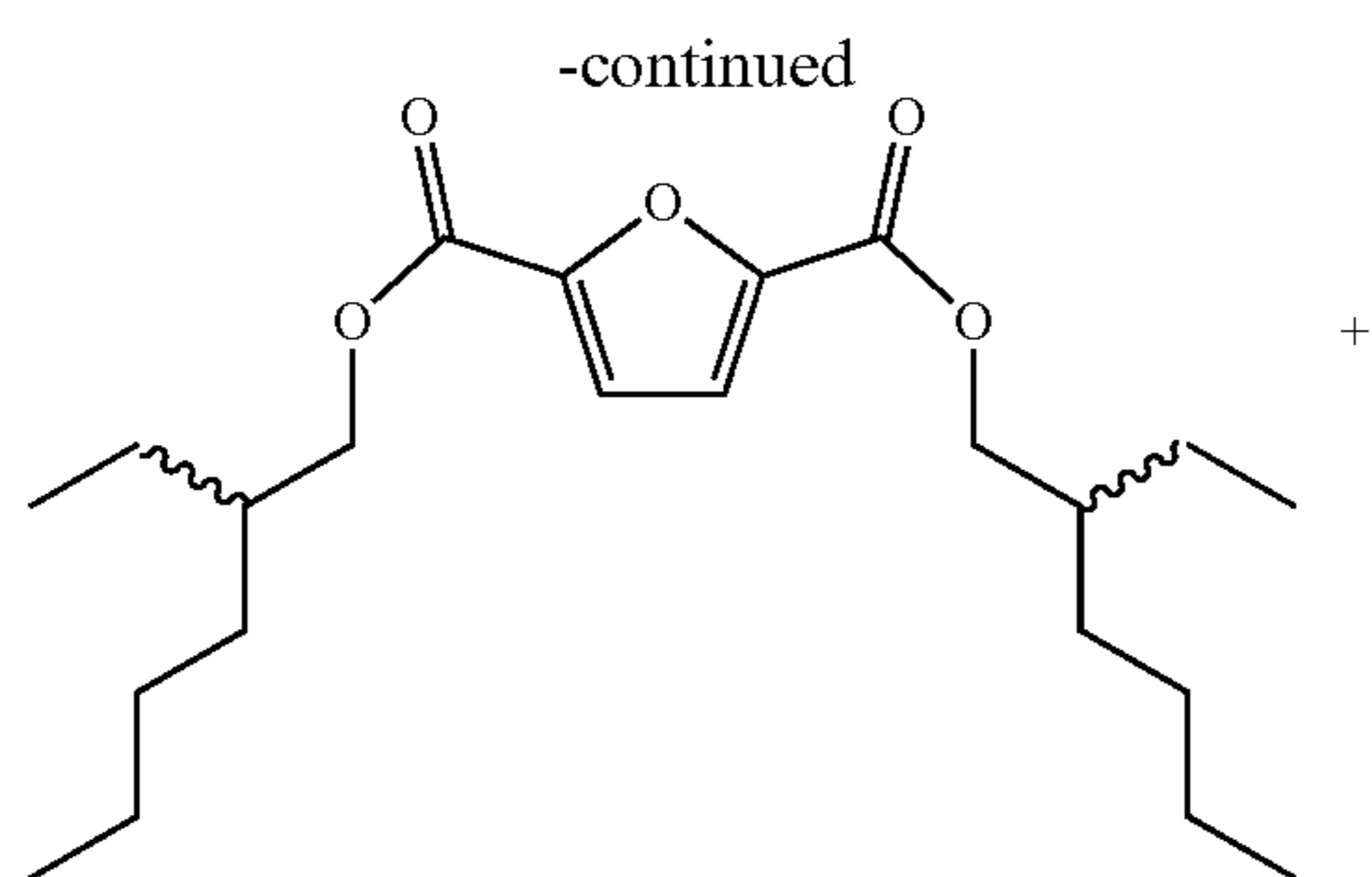
FD(2EH) Diastereomers)
