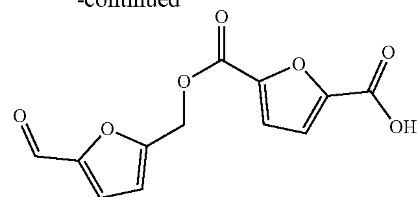
FDCA-HMF monoester
