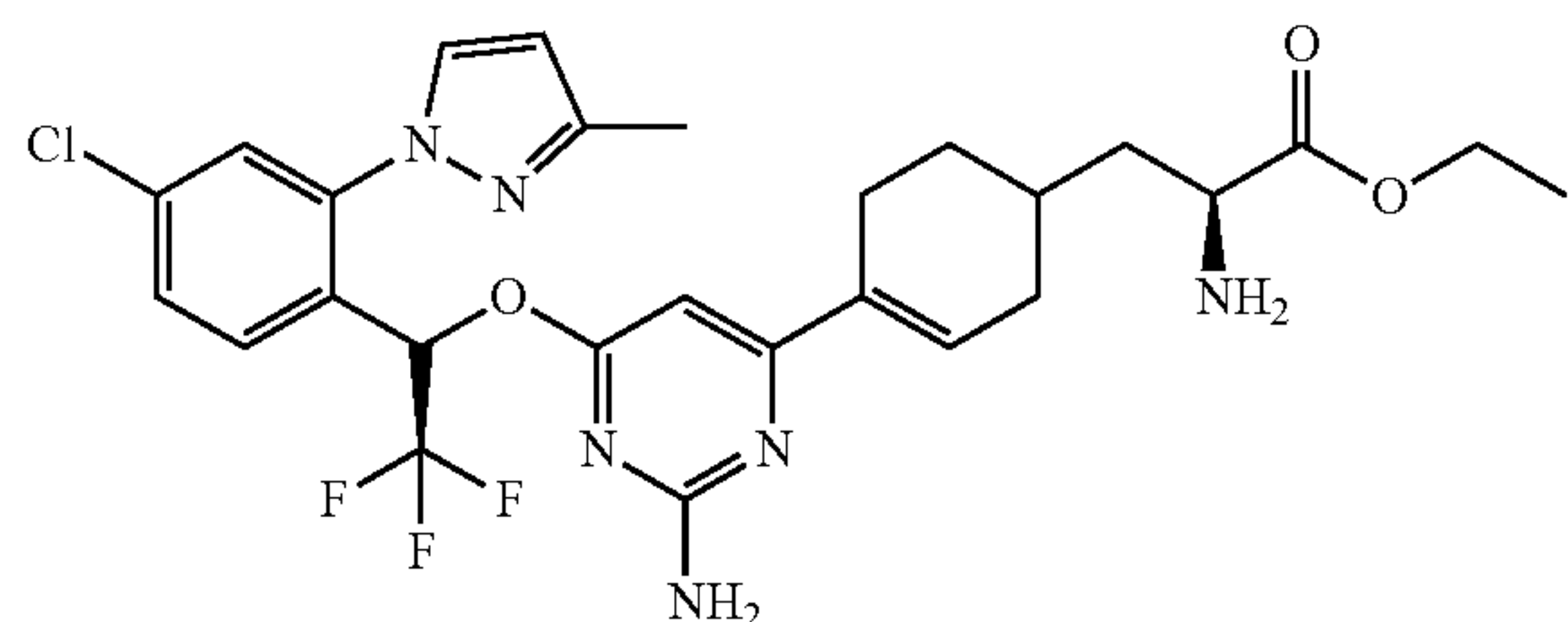
[Formula 36]
