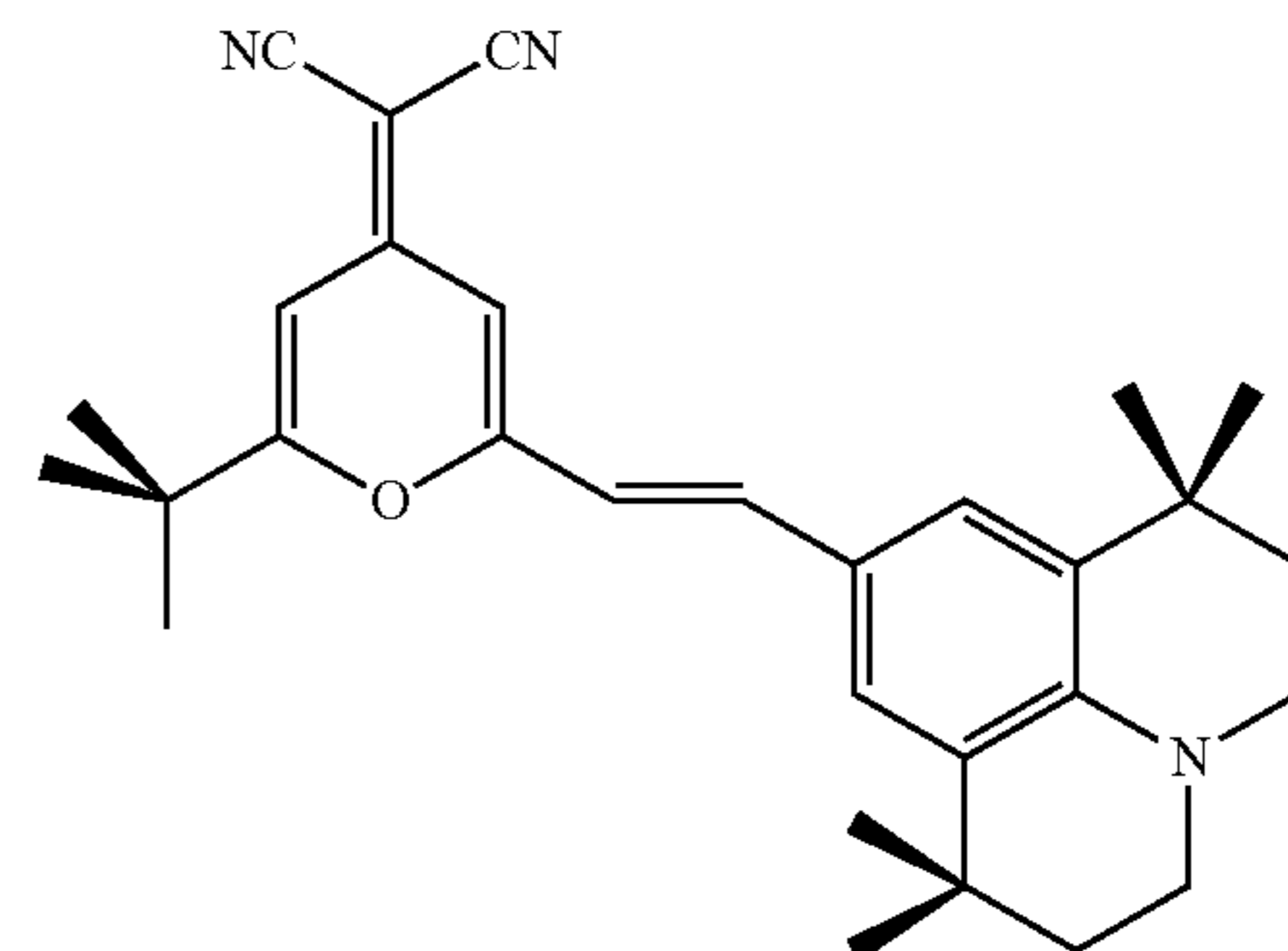
DCJTb
