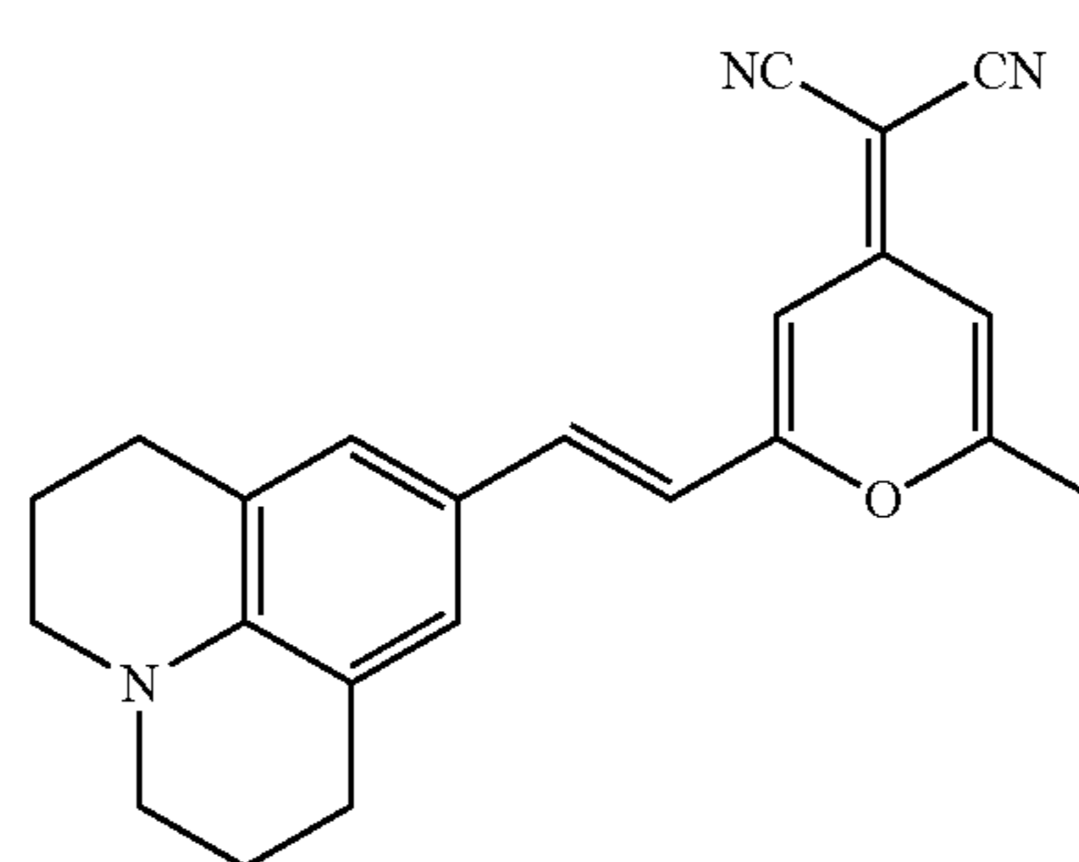
DCM
