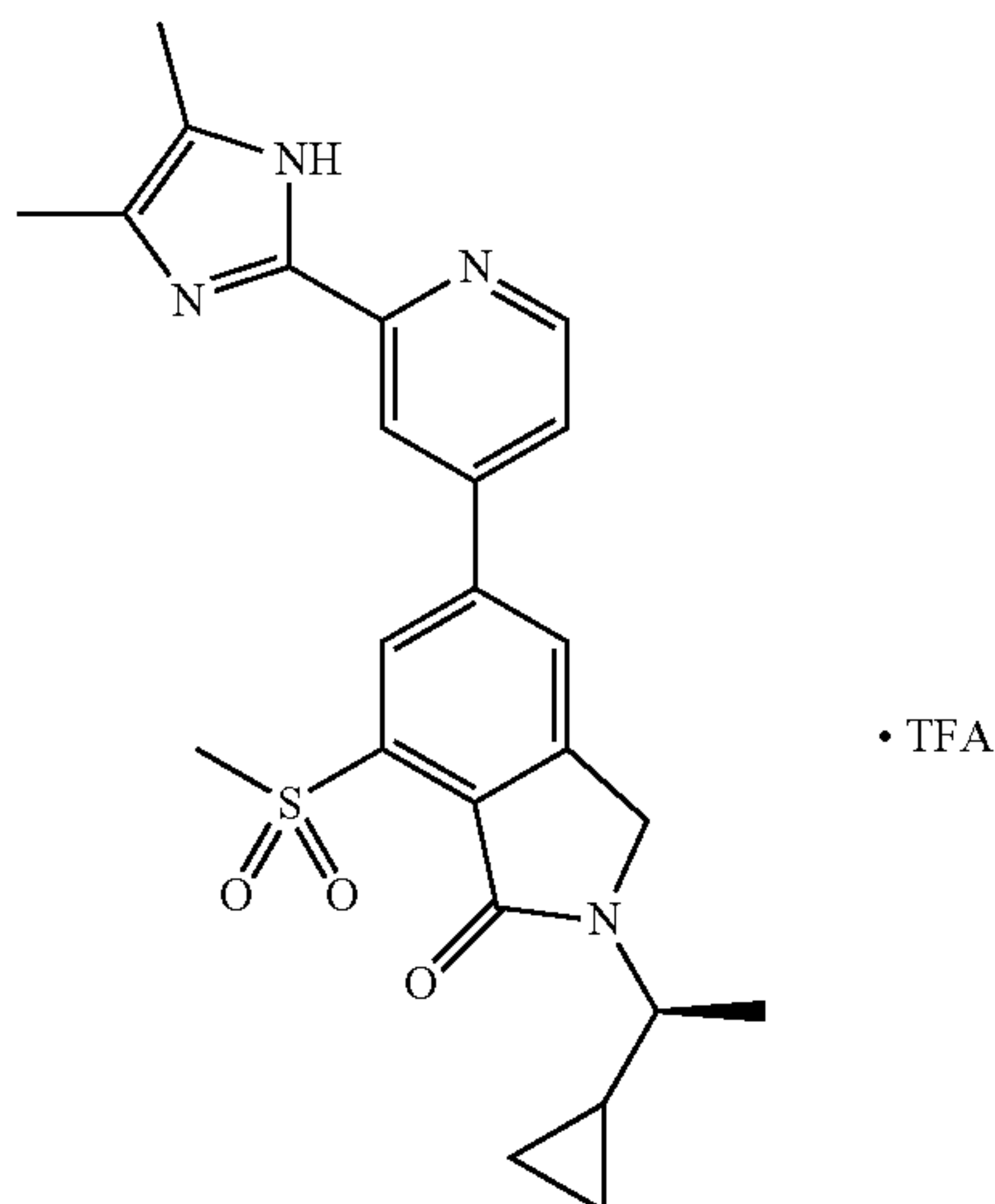
Step 1. (S)-5-Bromo-2-(1-cyclopropylethyl)-7-(methylthio)isoindolin-1-one
