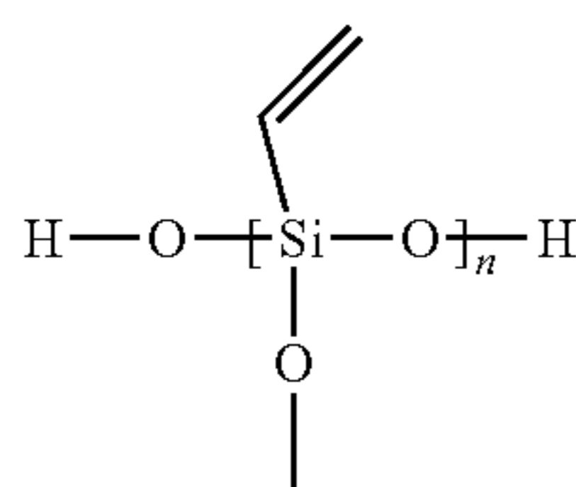
Vinylsilsesquioxane
