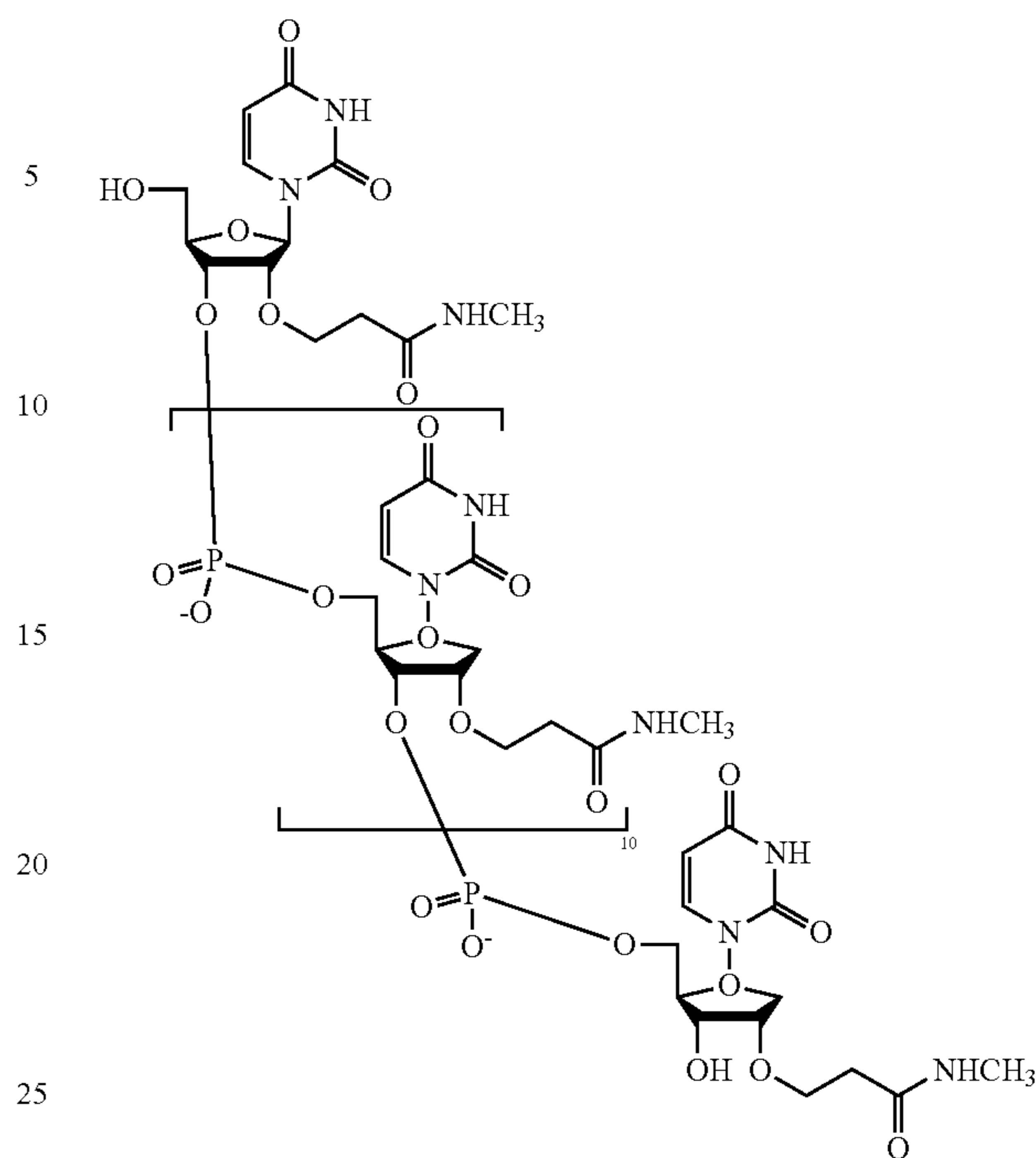
MCE (SEQ ID NO: 10)
