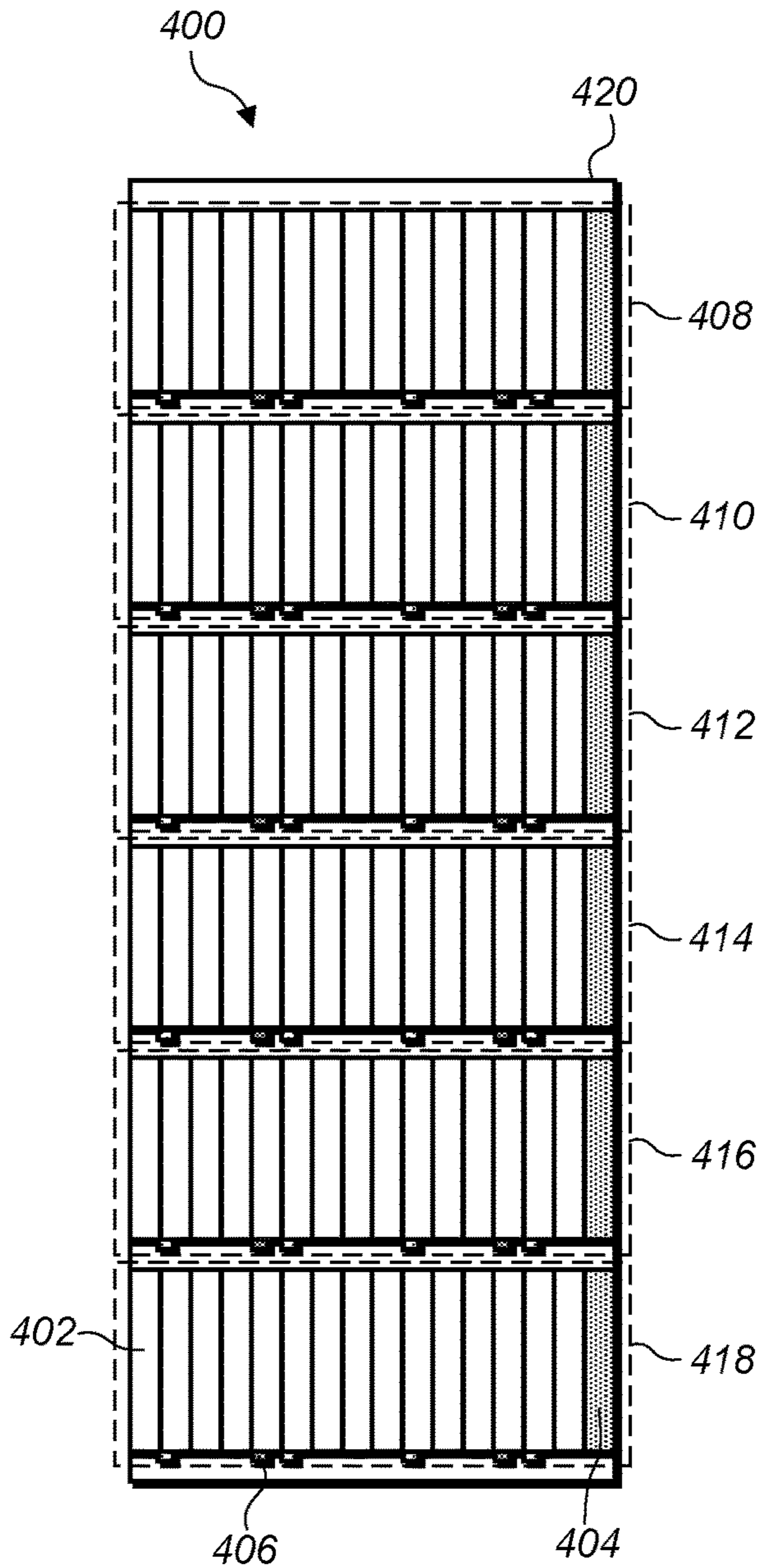
FIG. 4A
