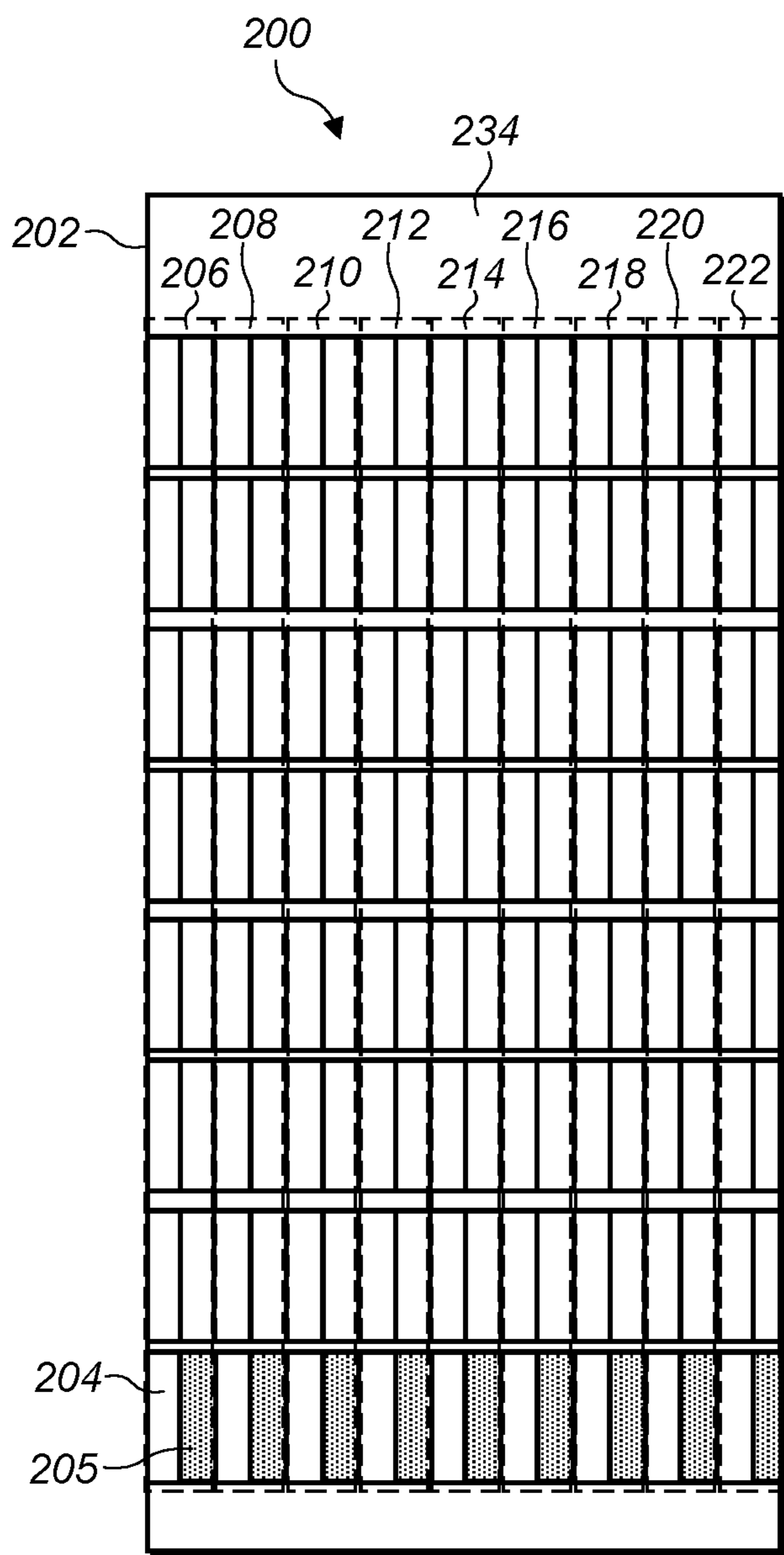
FIG. 2A
