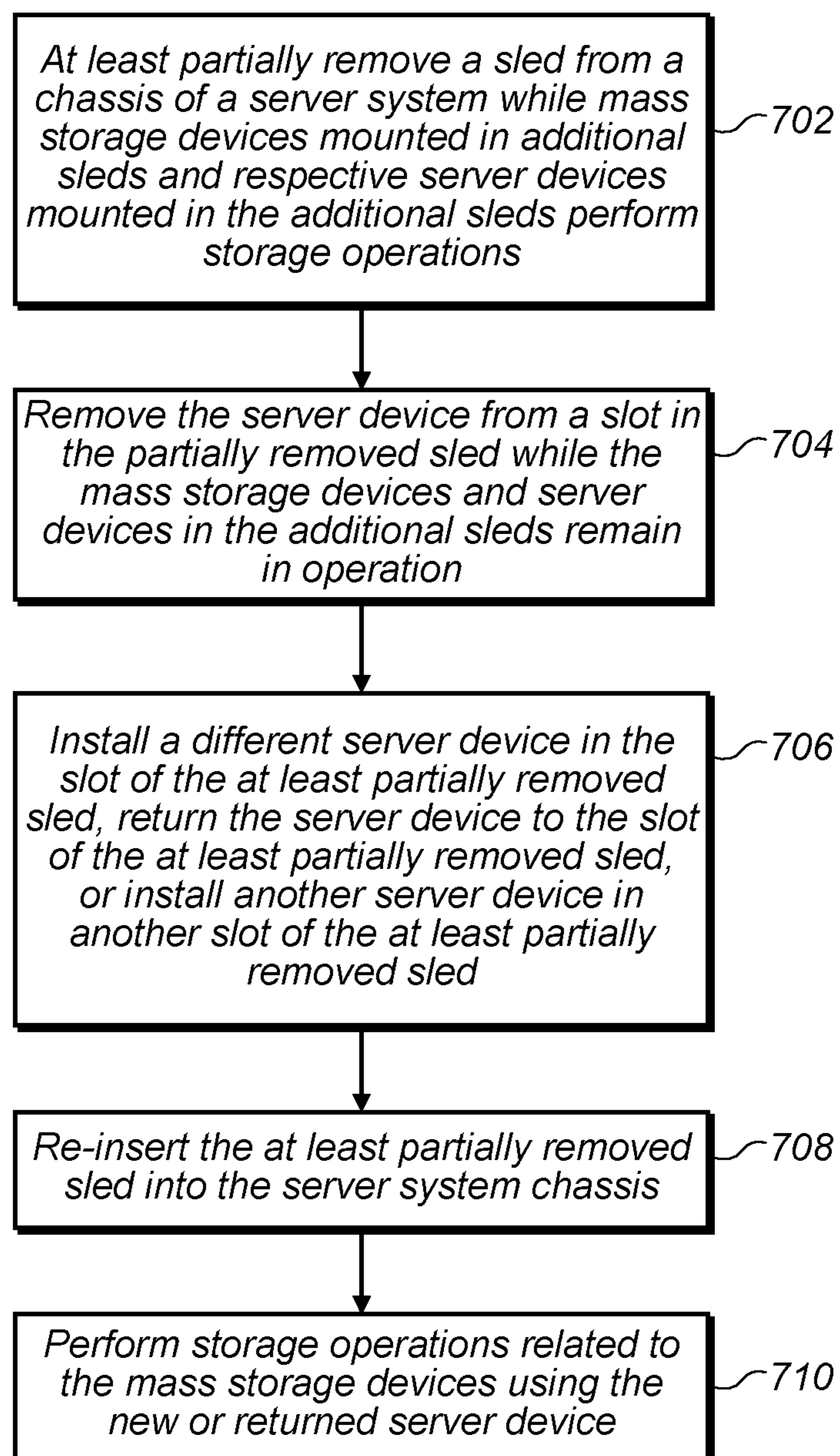
FIG. 7
