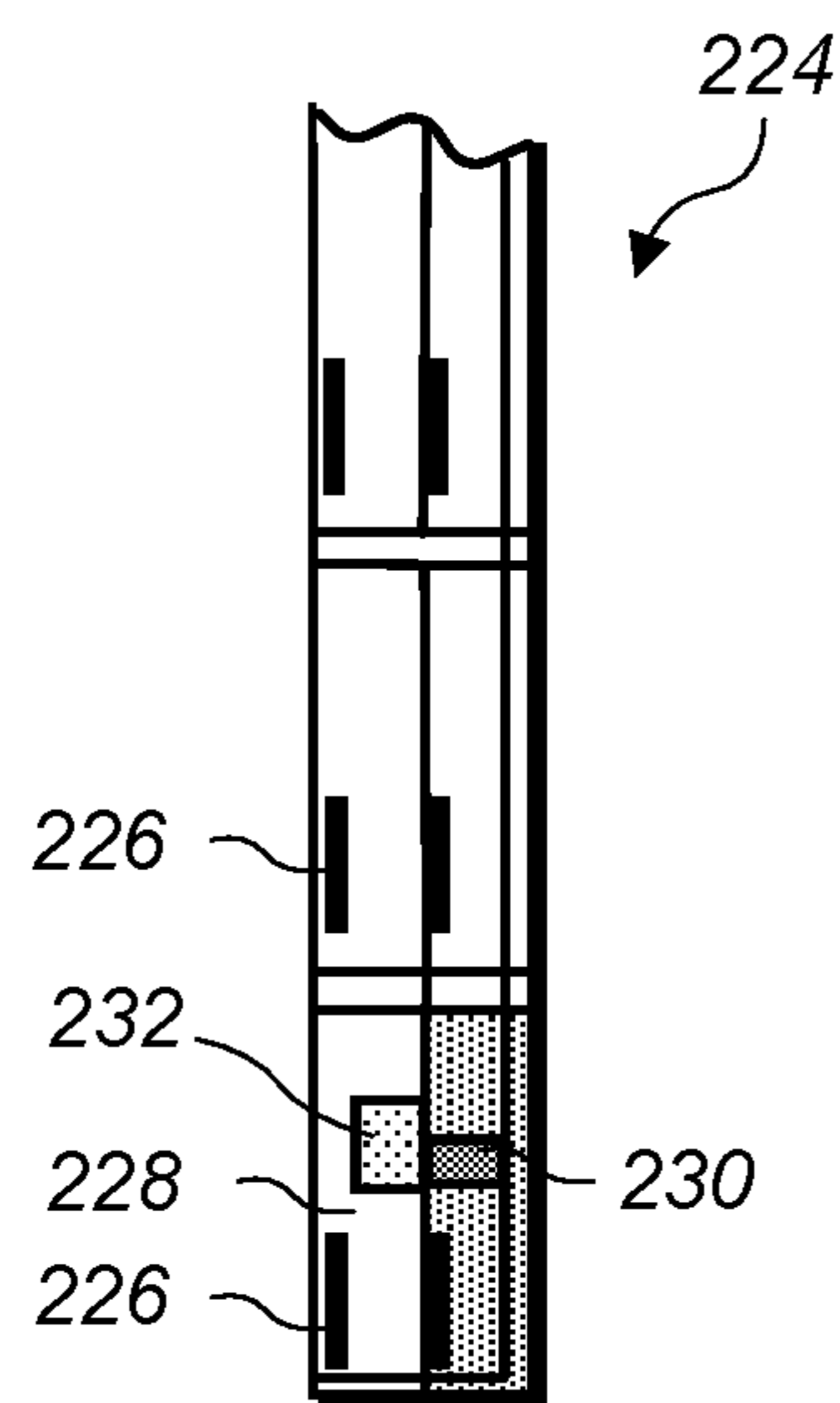
FIG. 2C
