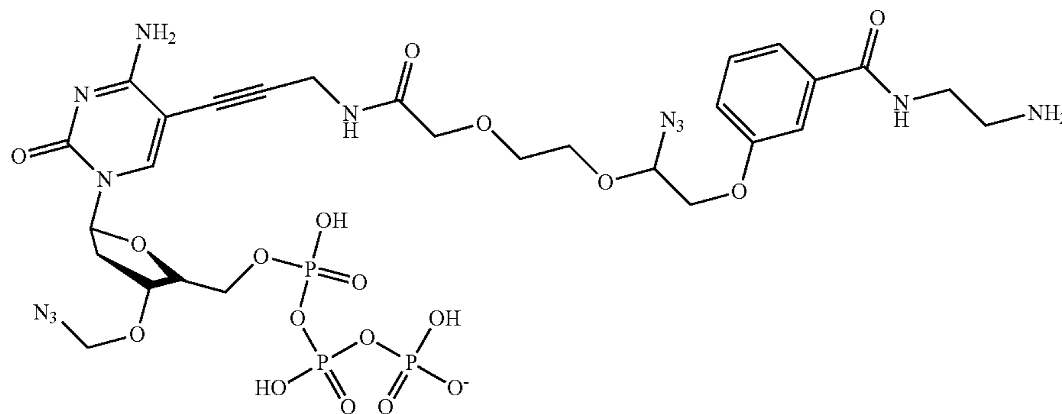
C-LN3-NH 2
