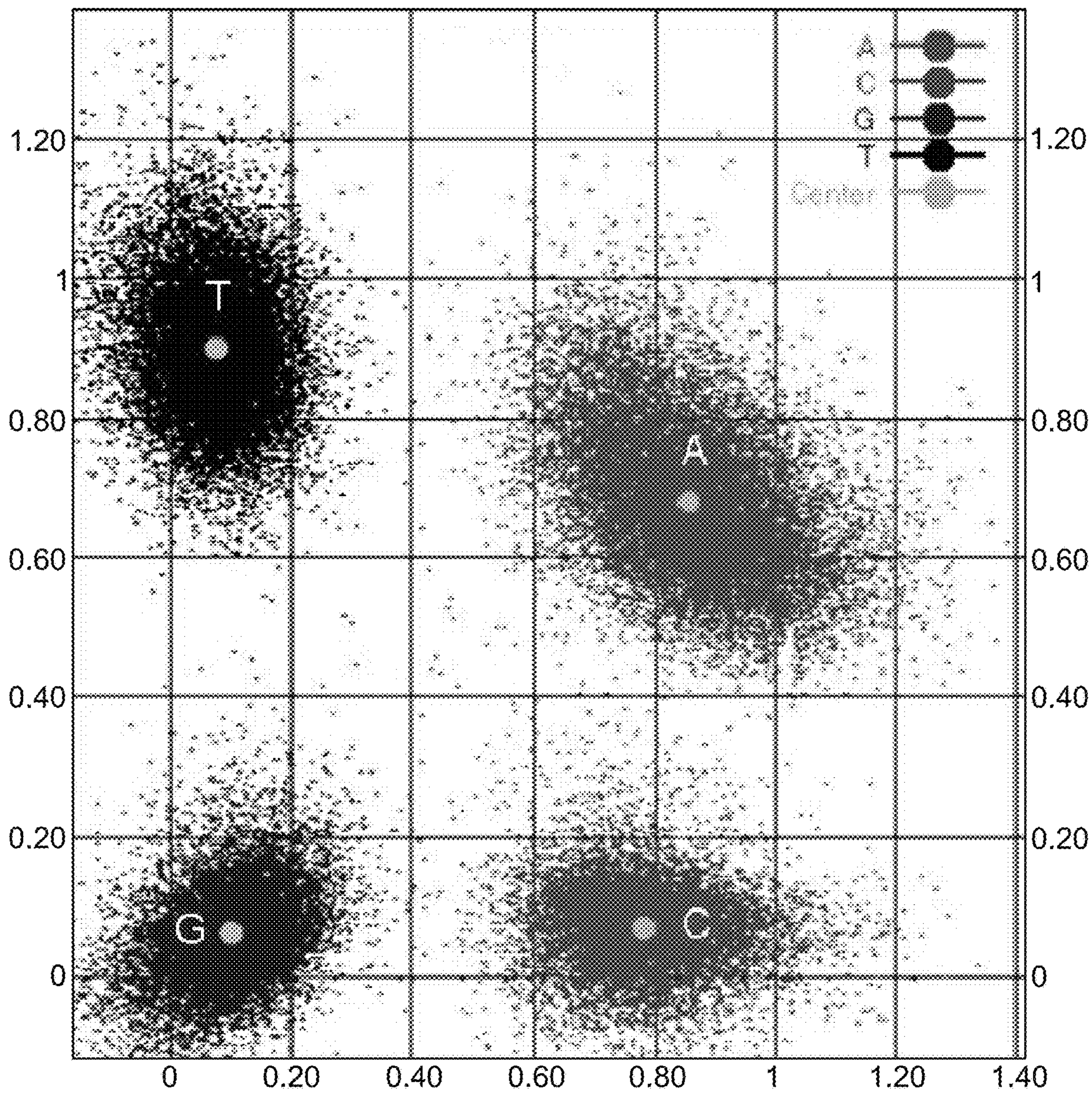
A- (Dye I-5)
