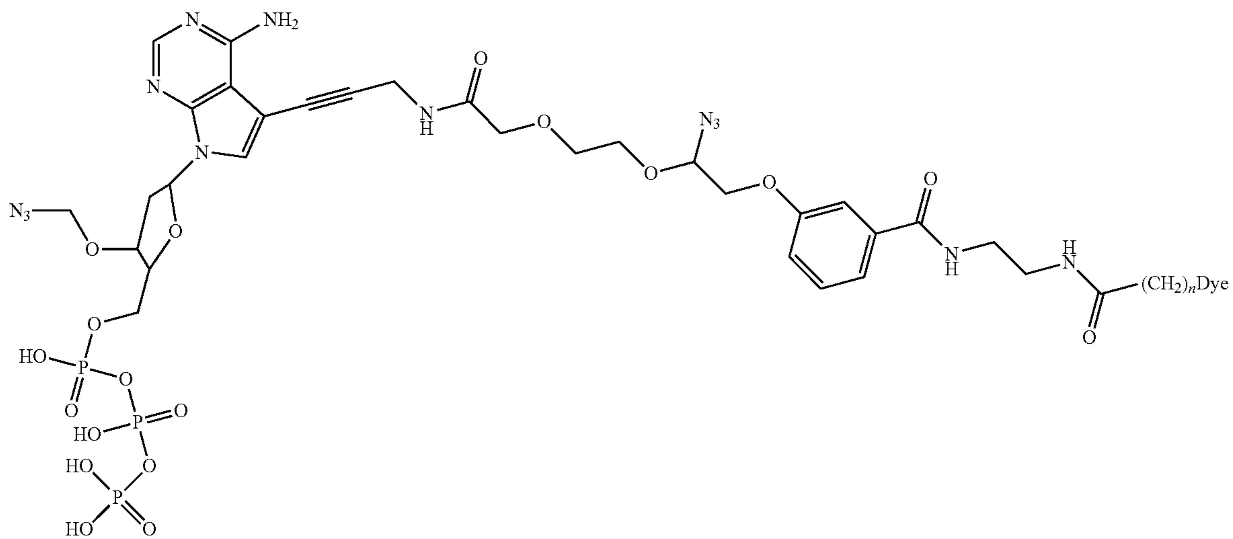
ffA-LN3-Dye
