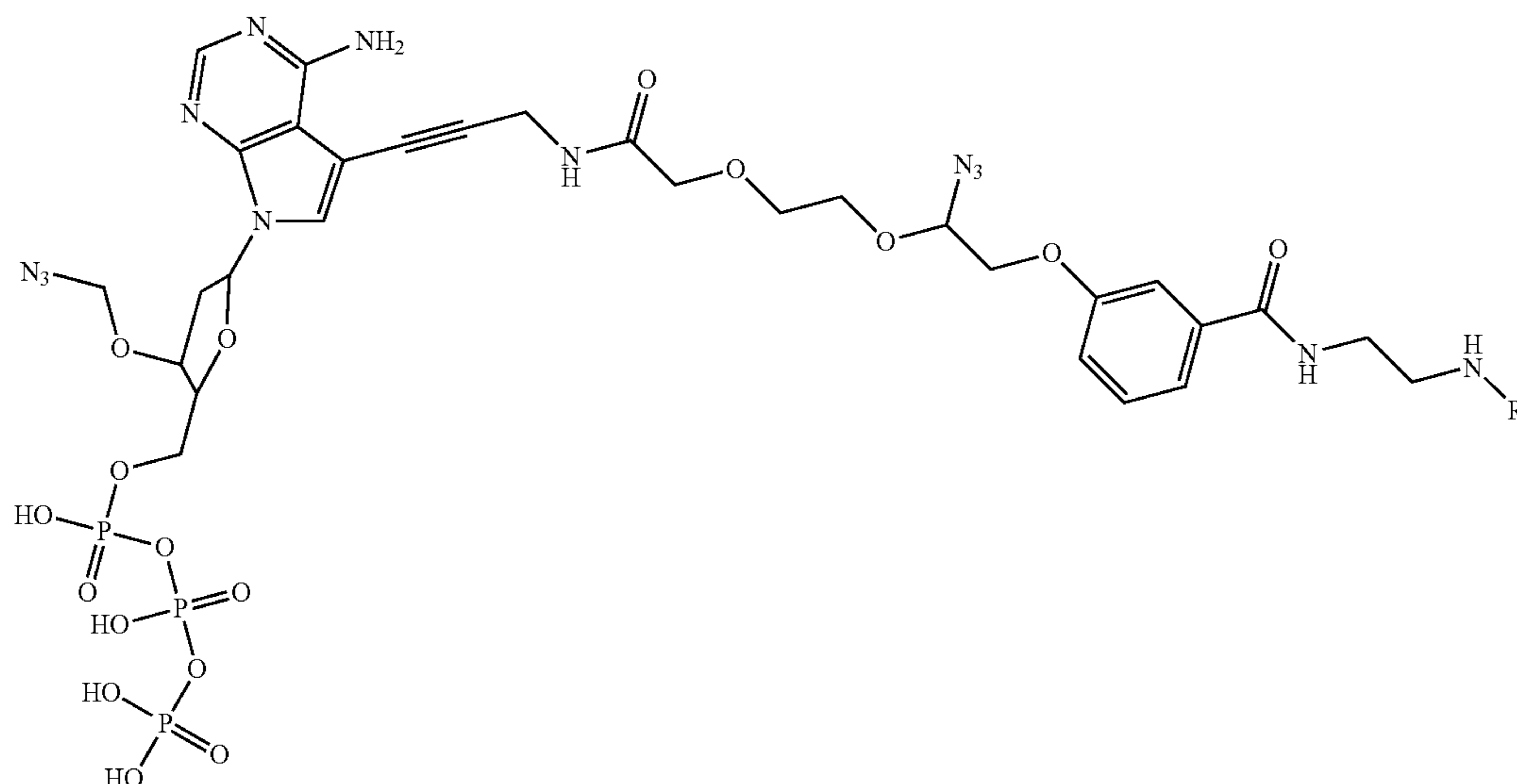
ffA-LN3-Dye
