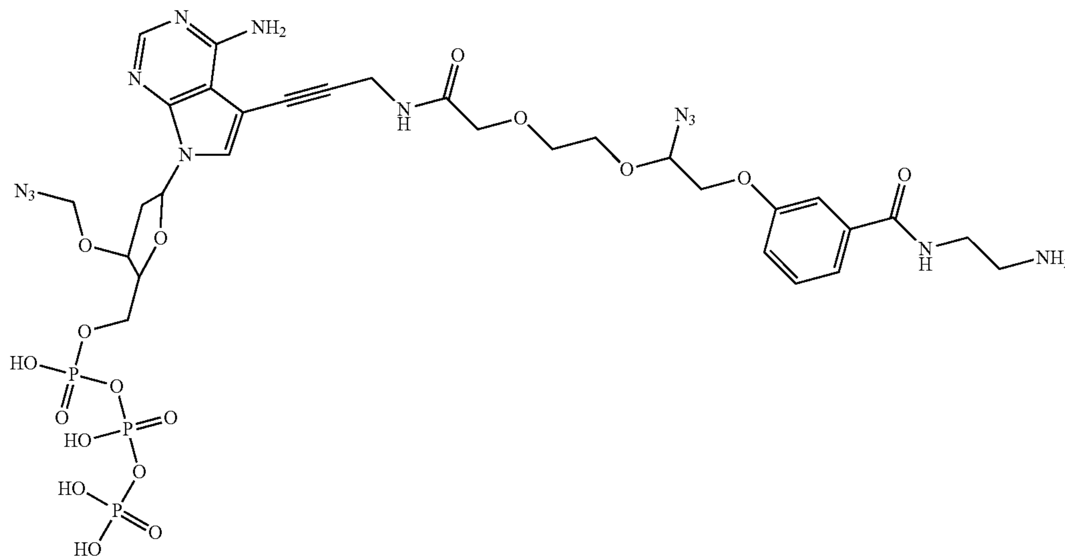
A-LN3-NH 2
