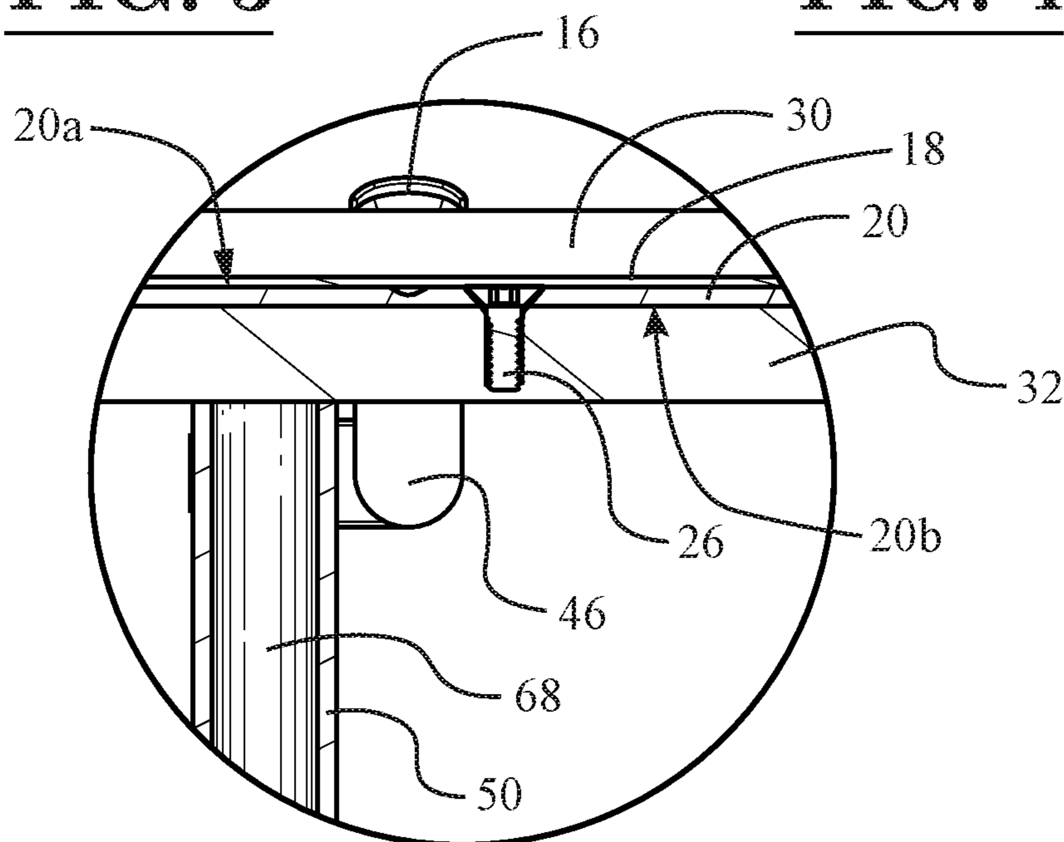
Section A-A FIG. 5
