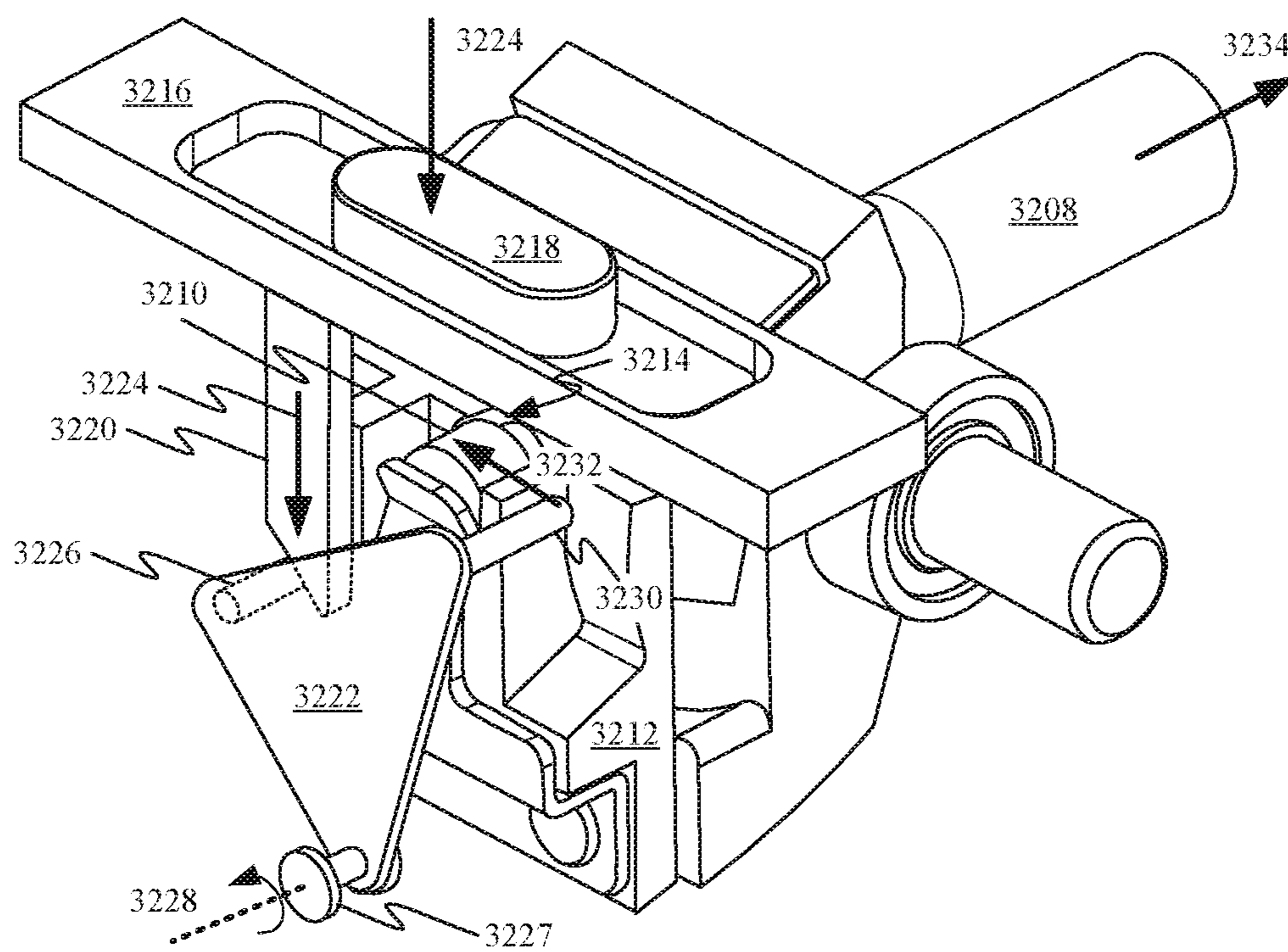
FIG. 32B
