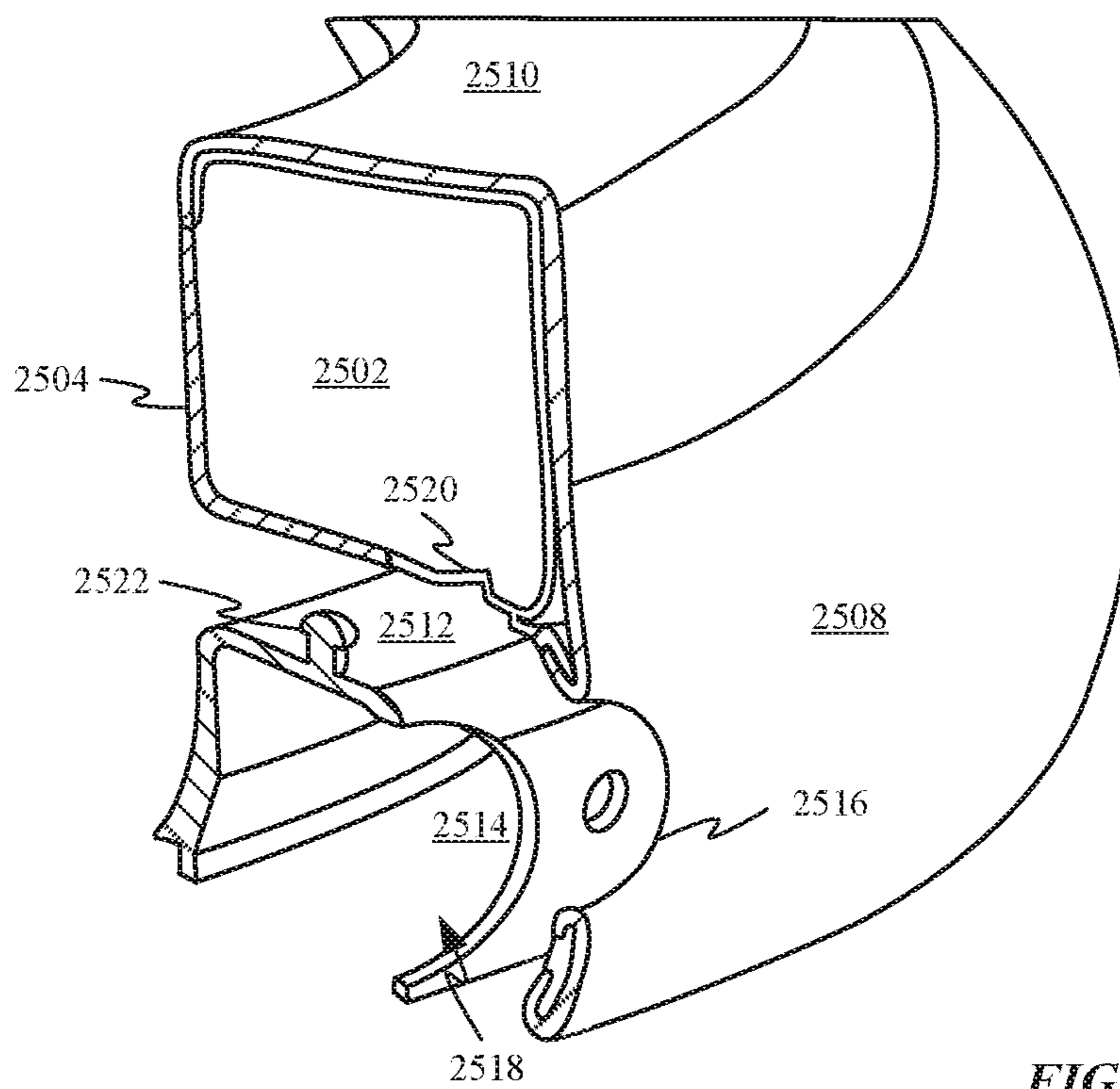
FIG. 25A
