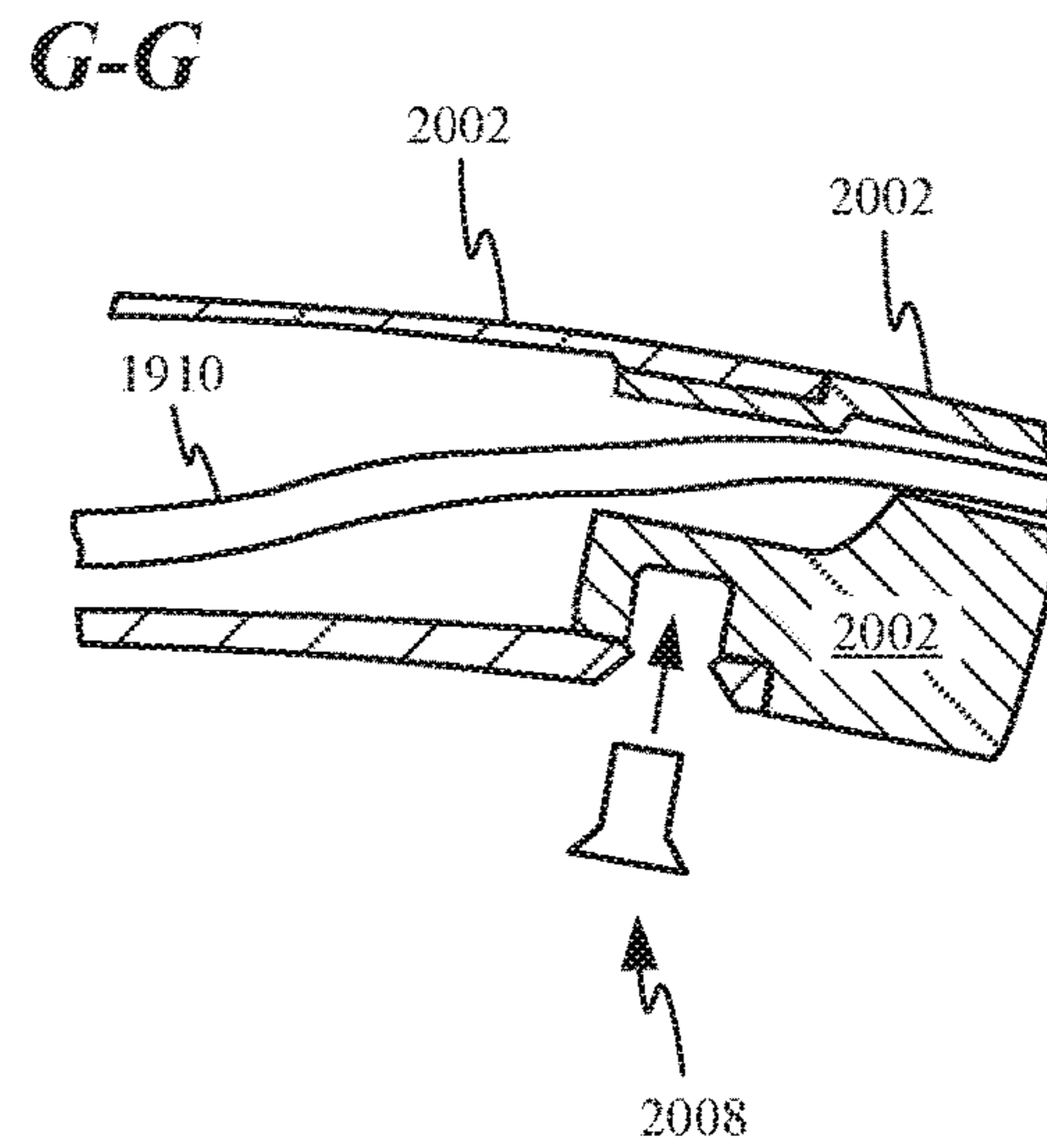
FIG. 20C
