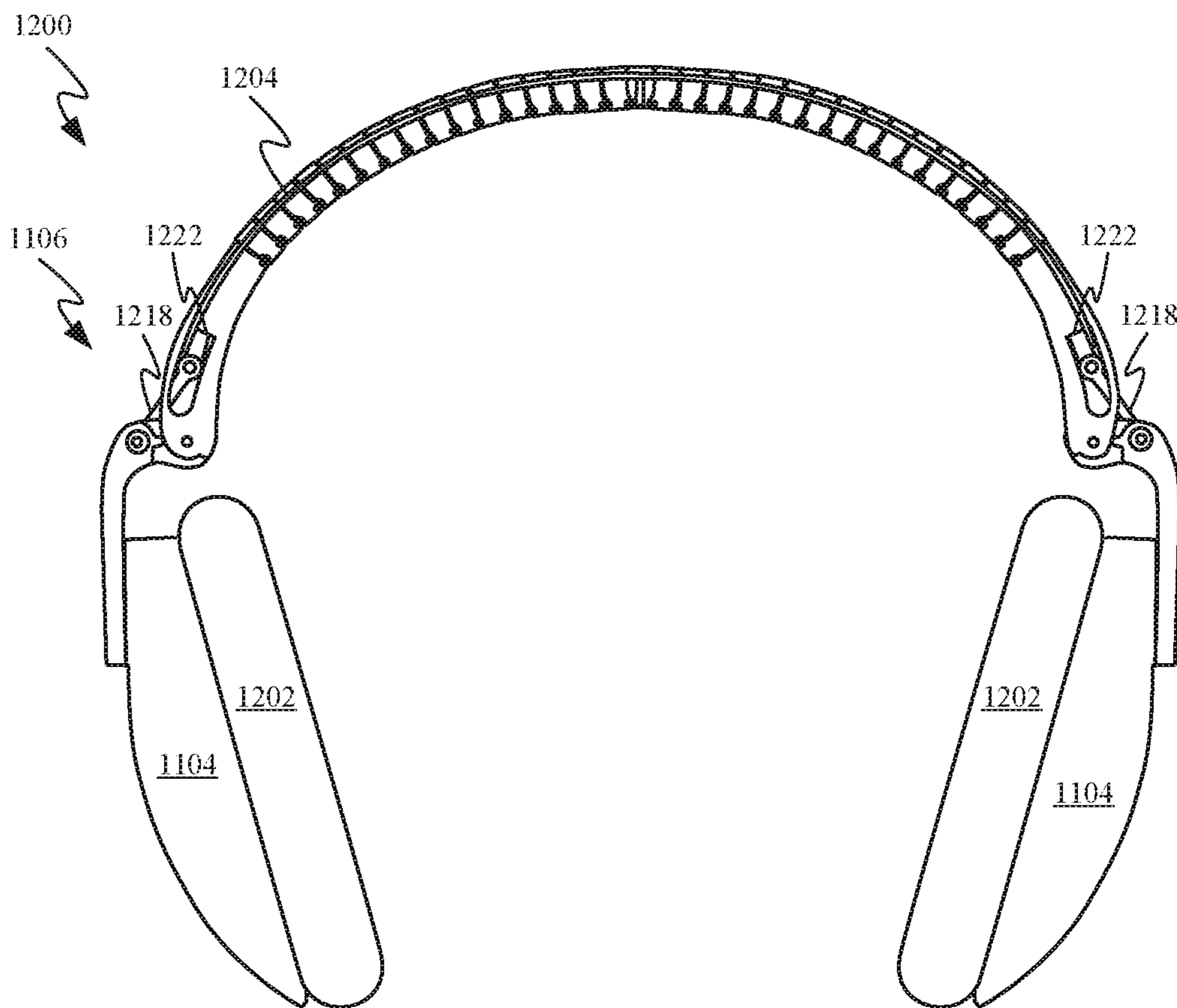
FIG. 12A
