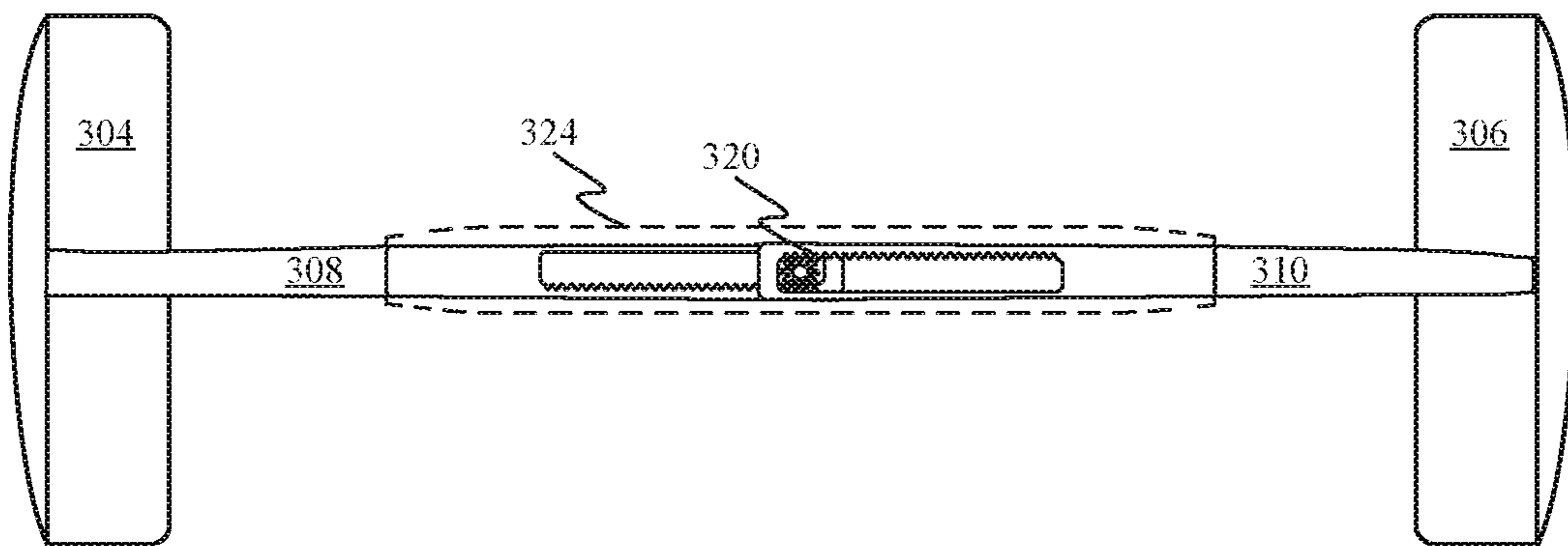
FIG. 3E
