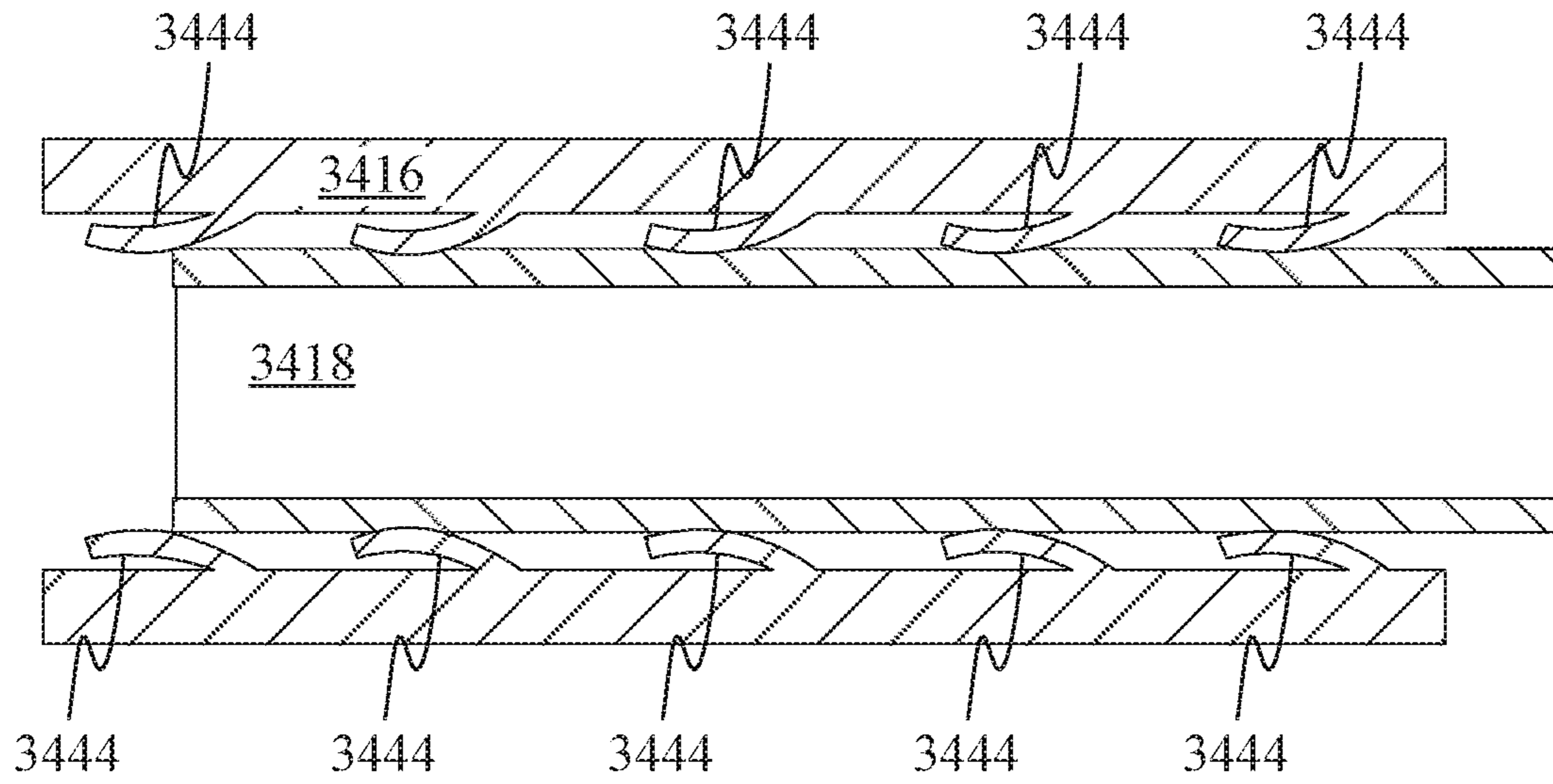
FIG. 34I
