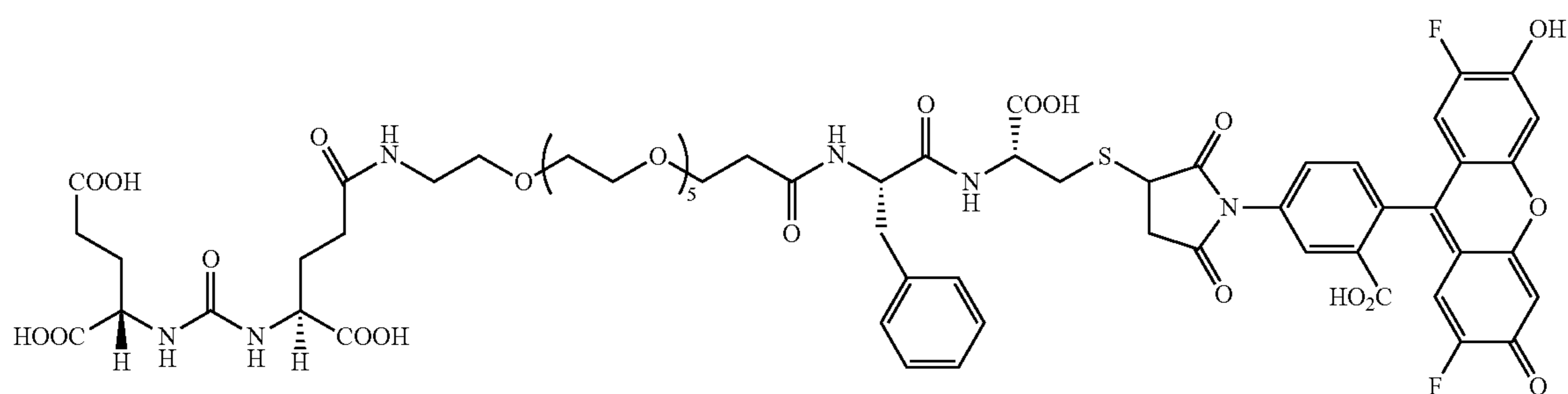
PC01SK56 C 52 H 70 F 2 N 6 O 25 S Mol. Wt.: 1369.31
