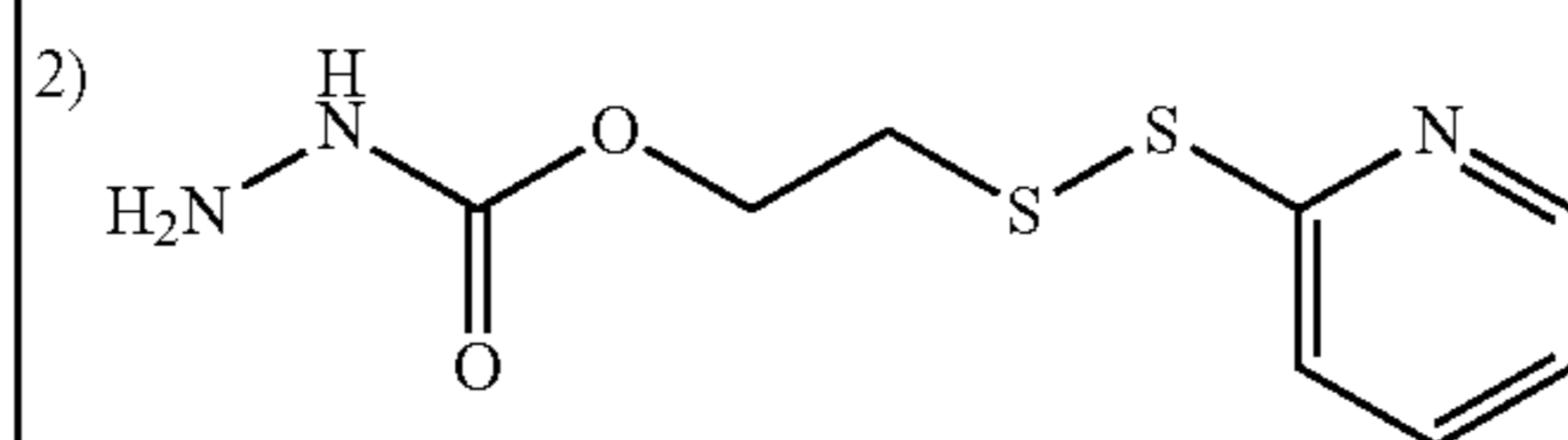
EC0311 C_8H_{11}N_3O_2S_2 Mol. Wt.: 245.32
