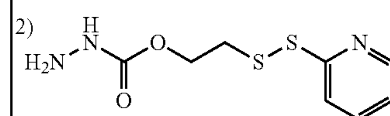
EC0311 C_8H_{11}N_3O_2S_2 Mol. Wt.: 245.32
