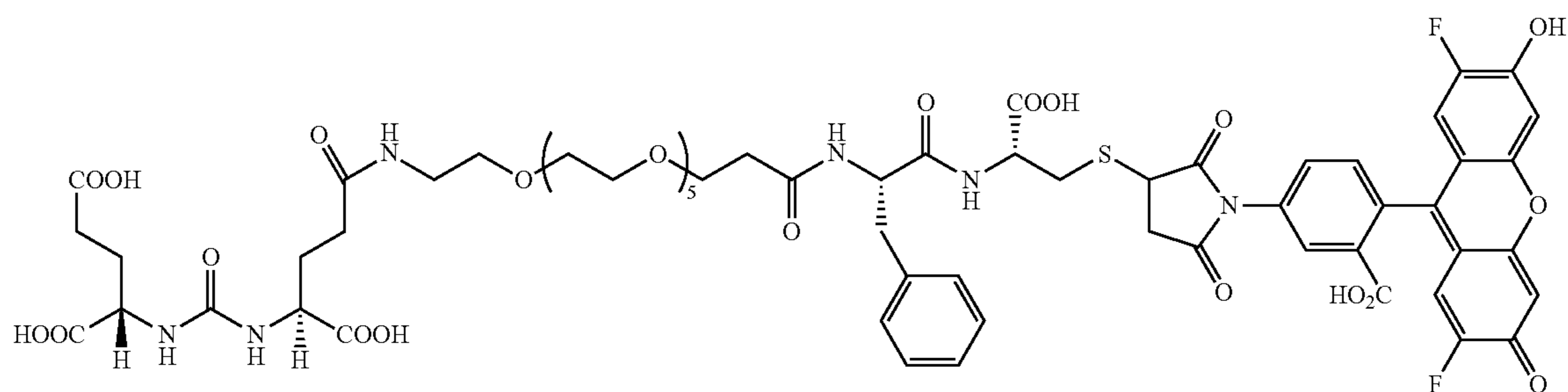
PC01SK56 C_{52}H_{70}F_2N_6O_{25}S Mol. Wt.: 1369.31
