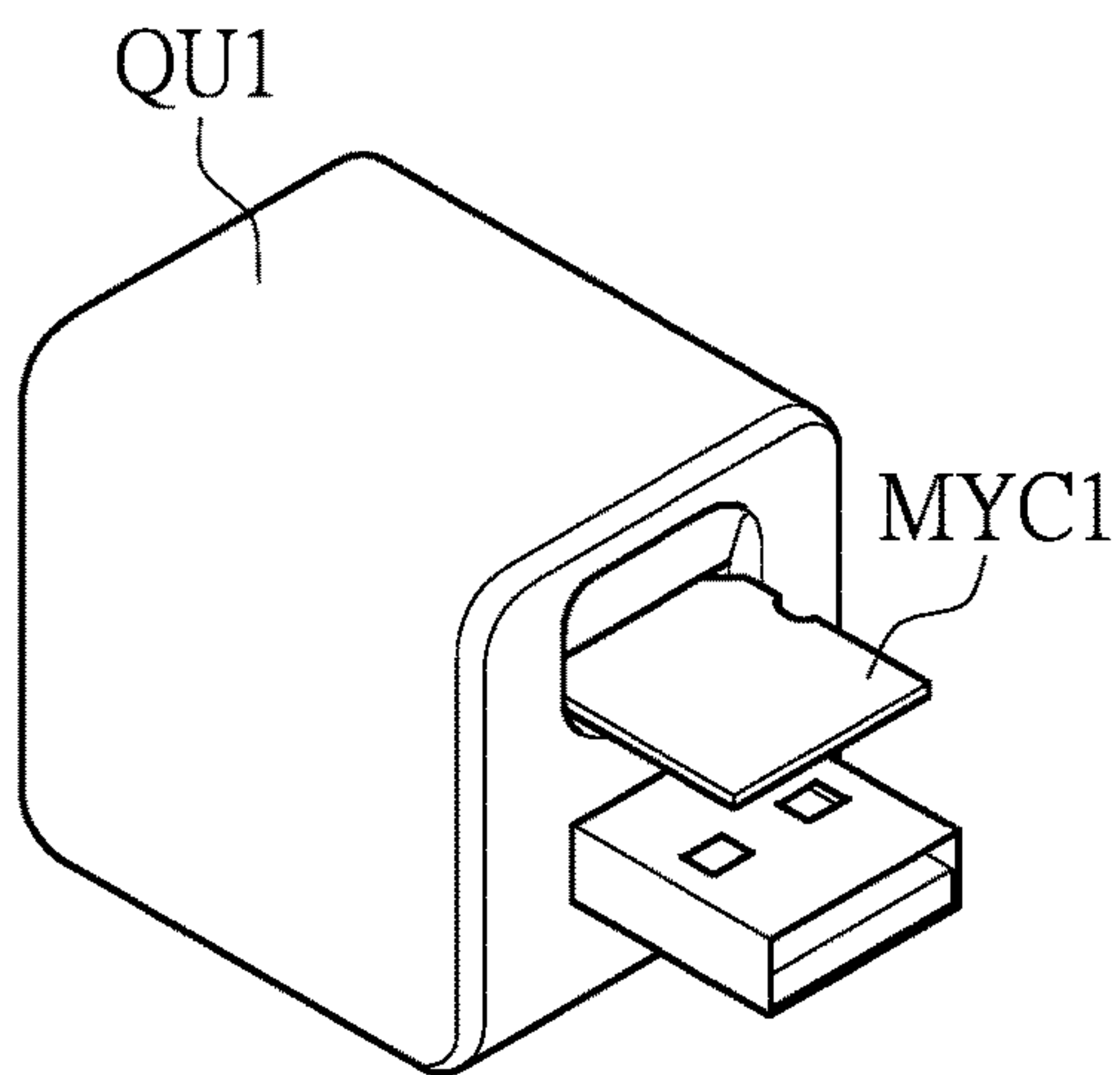
FIG. 2B
