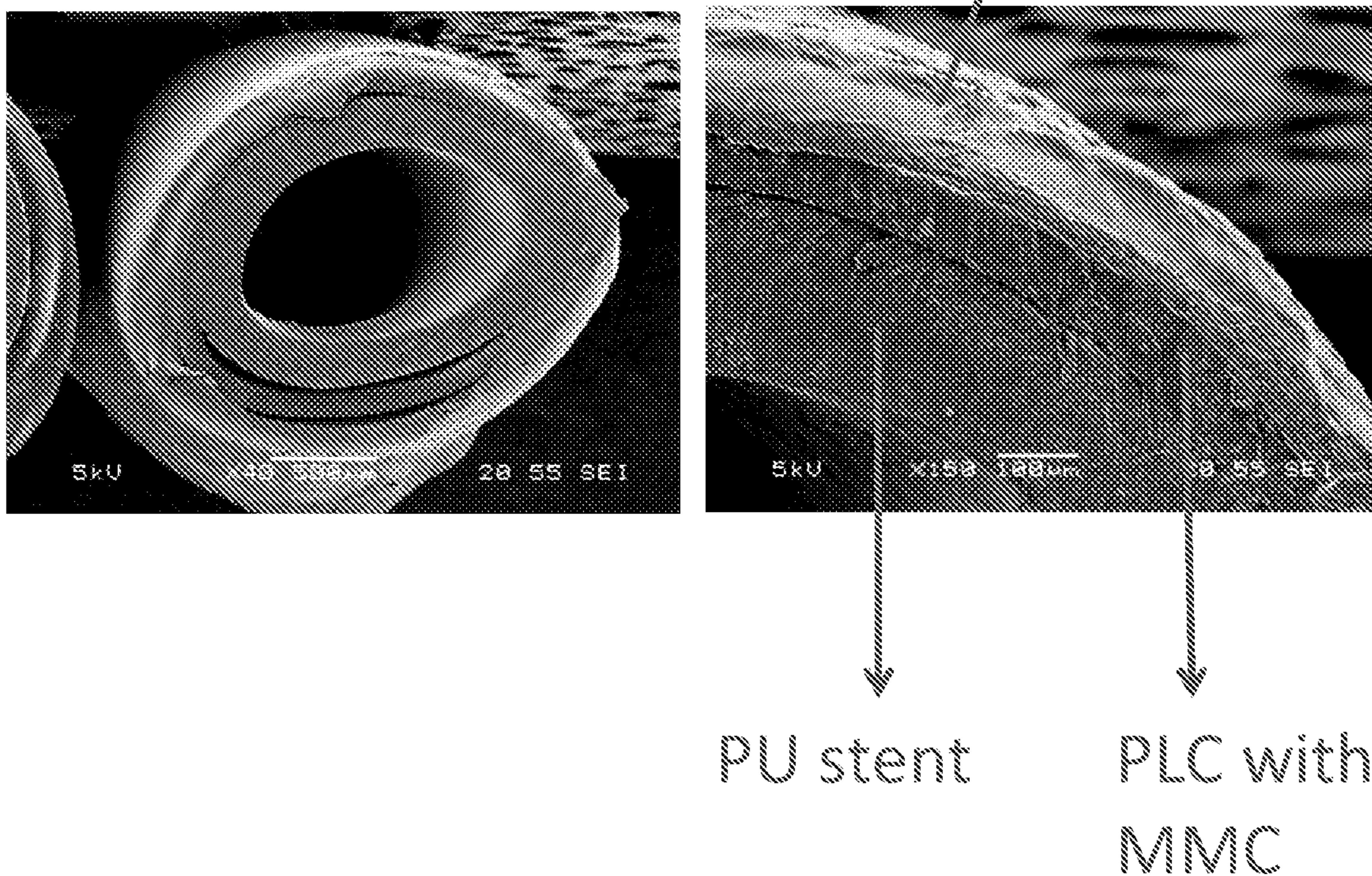
(D) 5% MMC, with PEGDA
