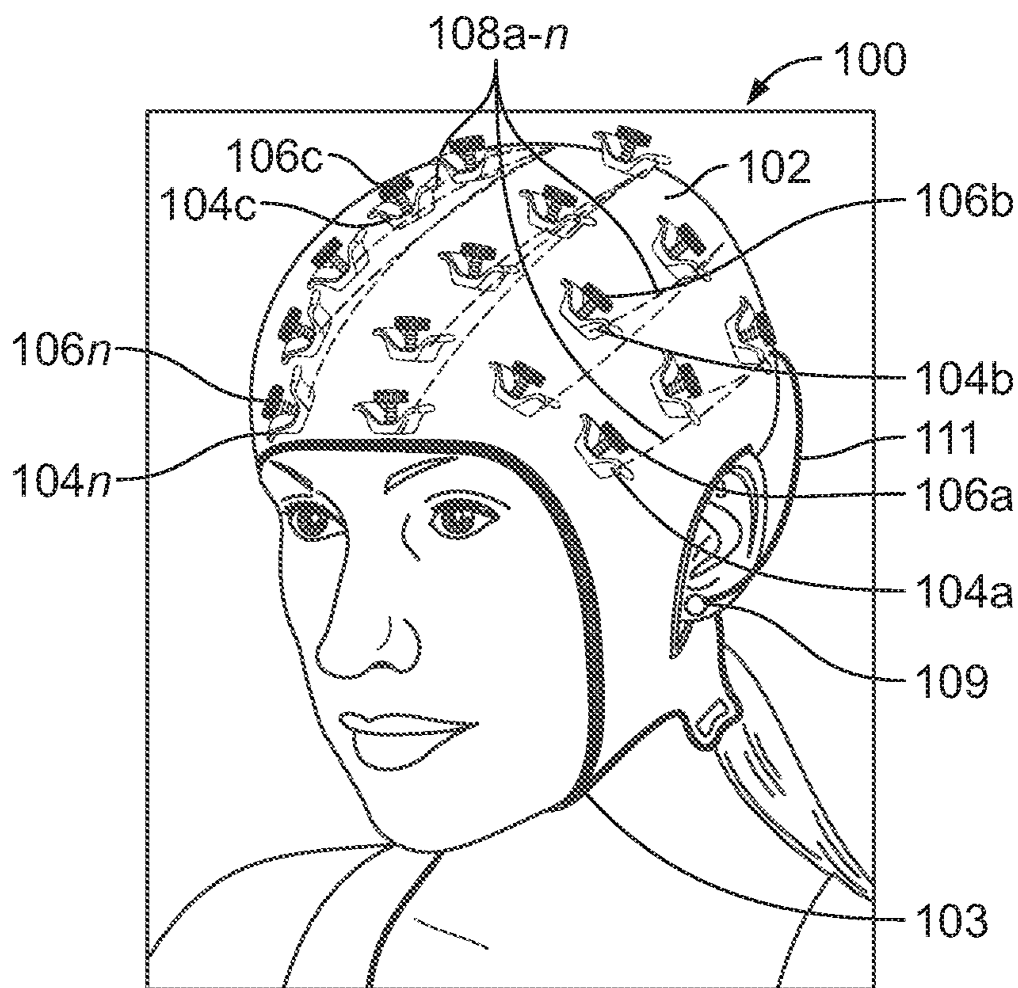
FIG. 1A
