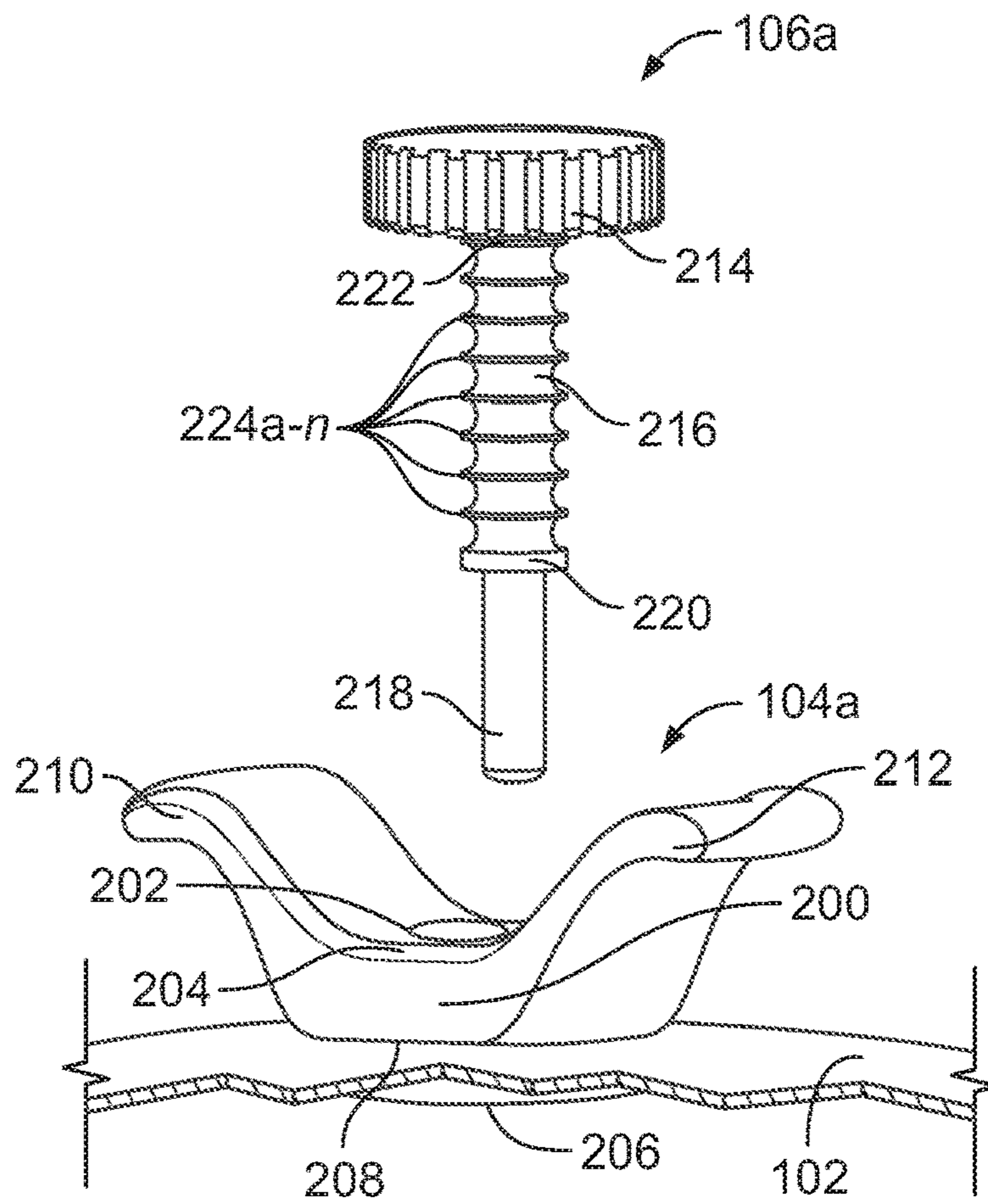
FIG. 2A
