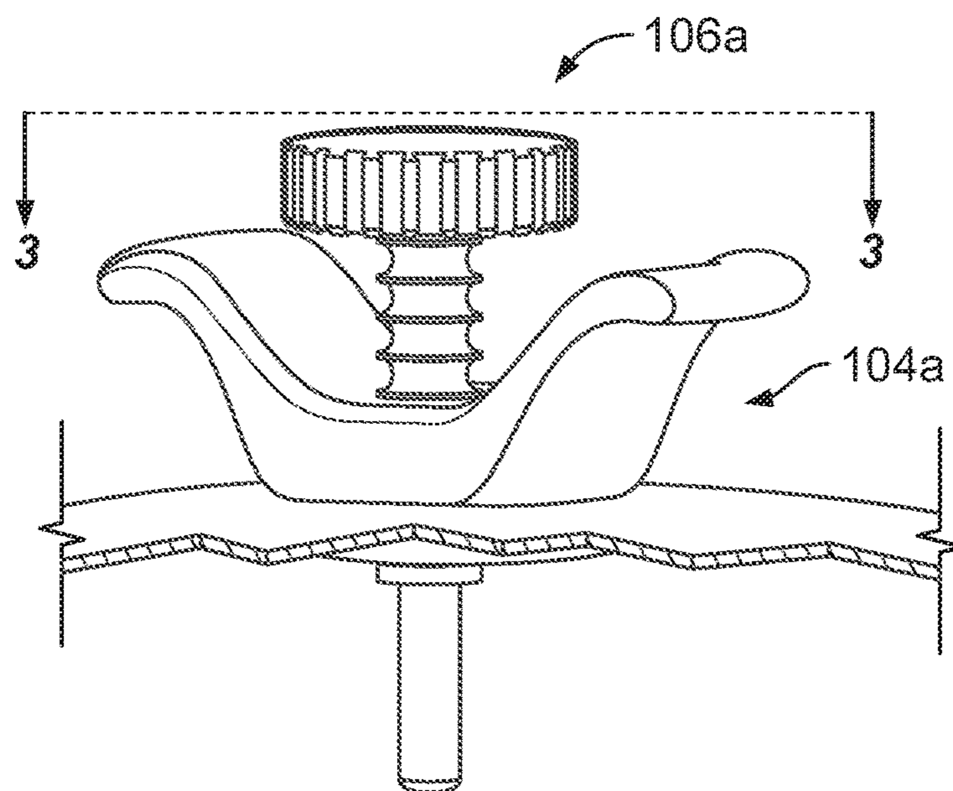
FIG. 2B
