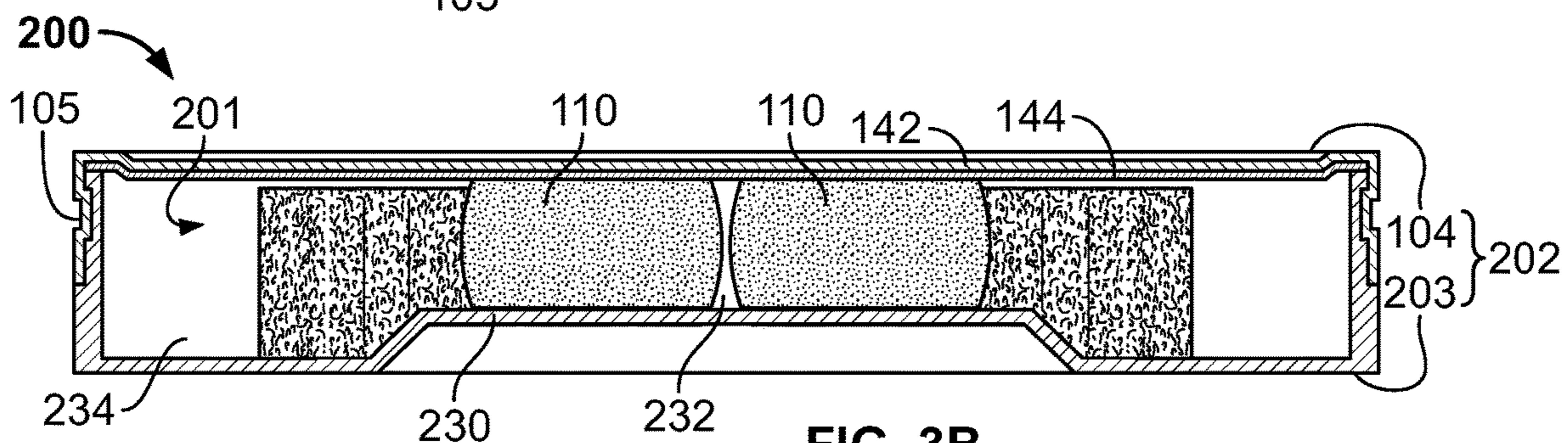
FIG. 3A
