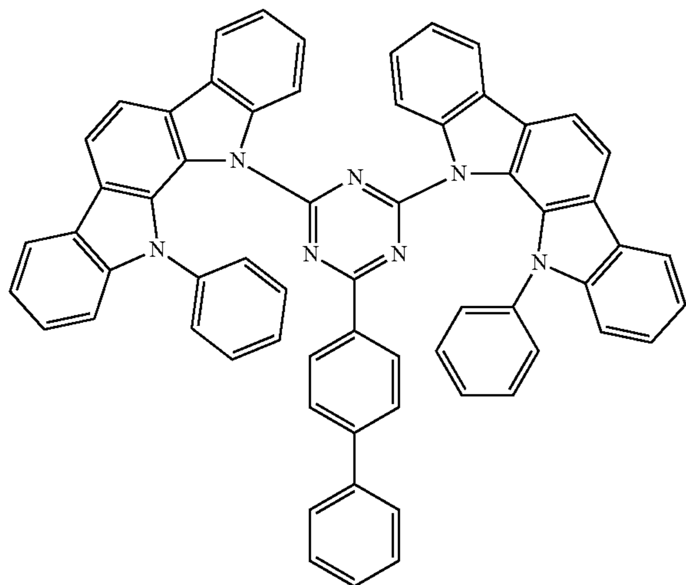
PIC-TRZ
