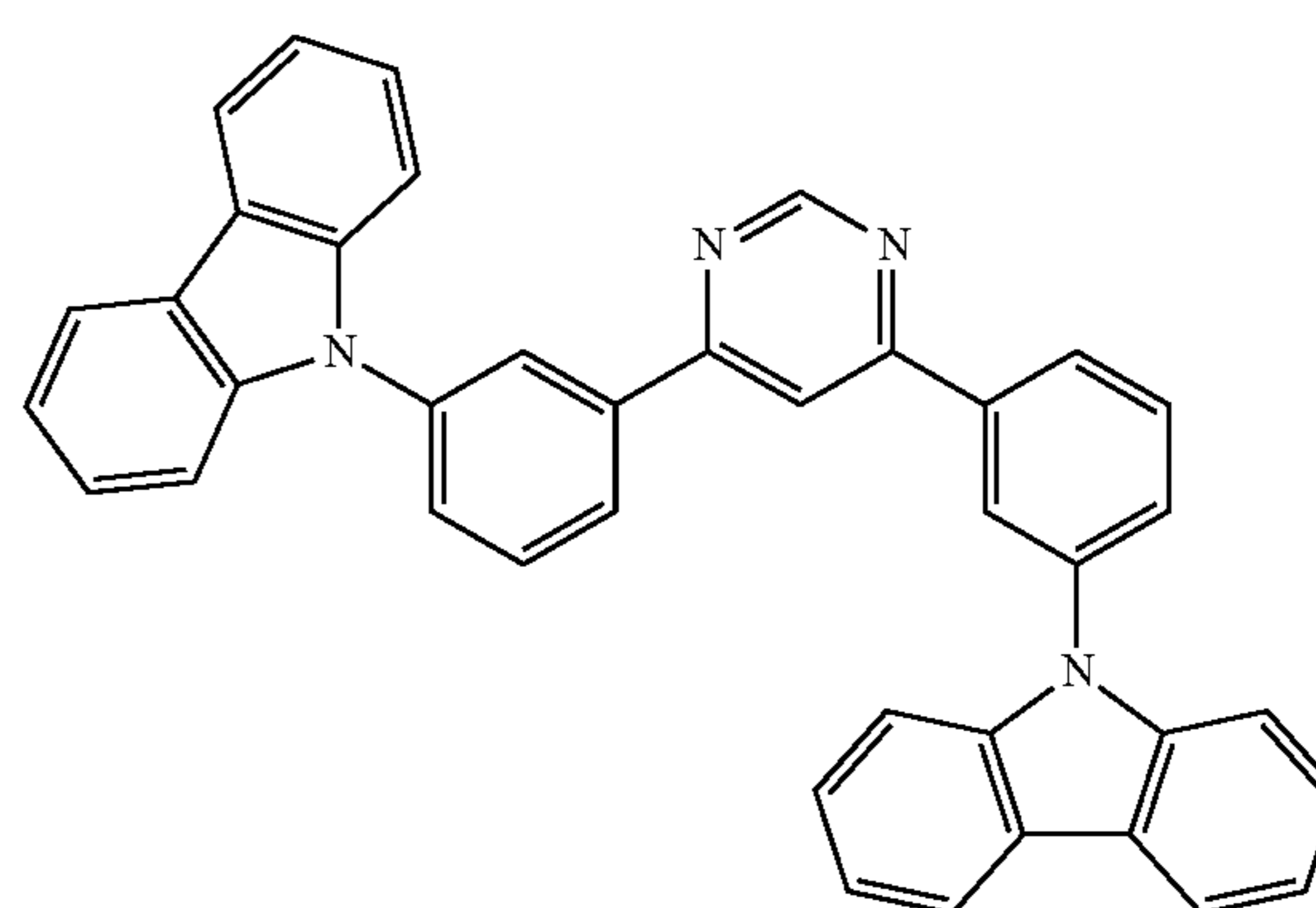
4,6mCzP2Pm
