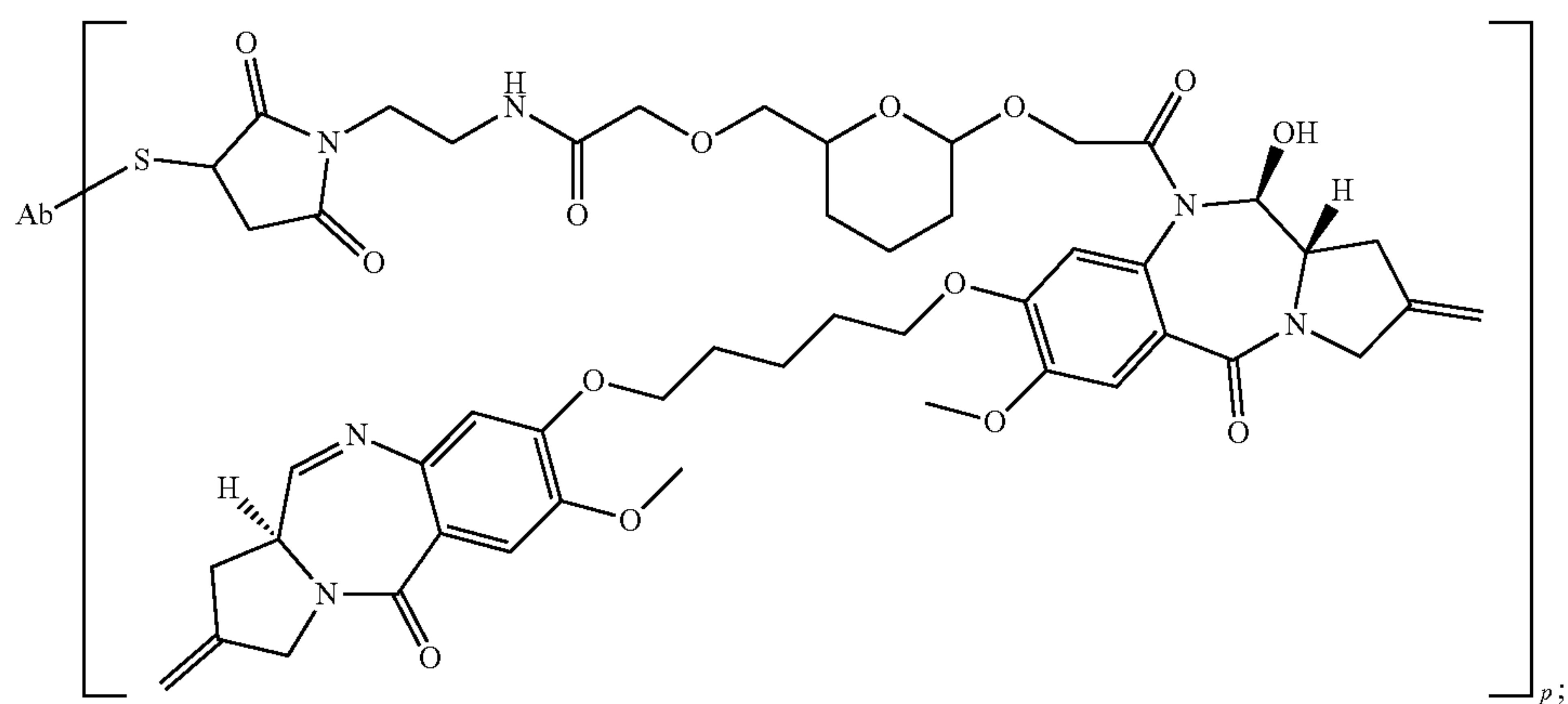
PBD dimer-val-cit-PAB-Ab
