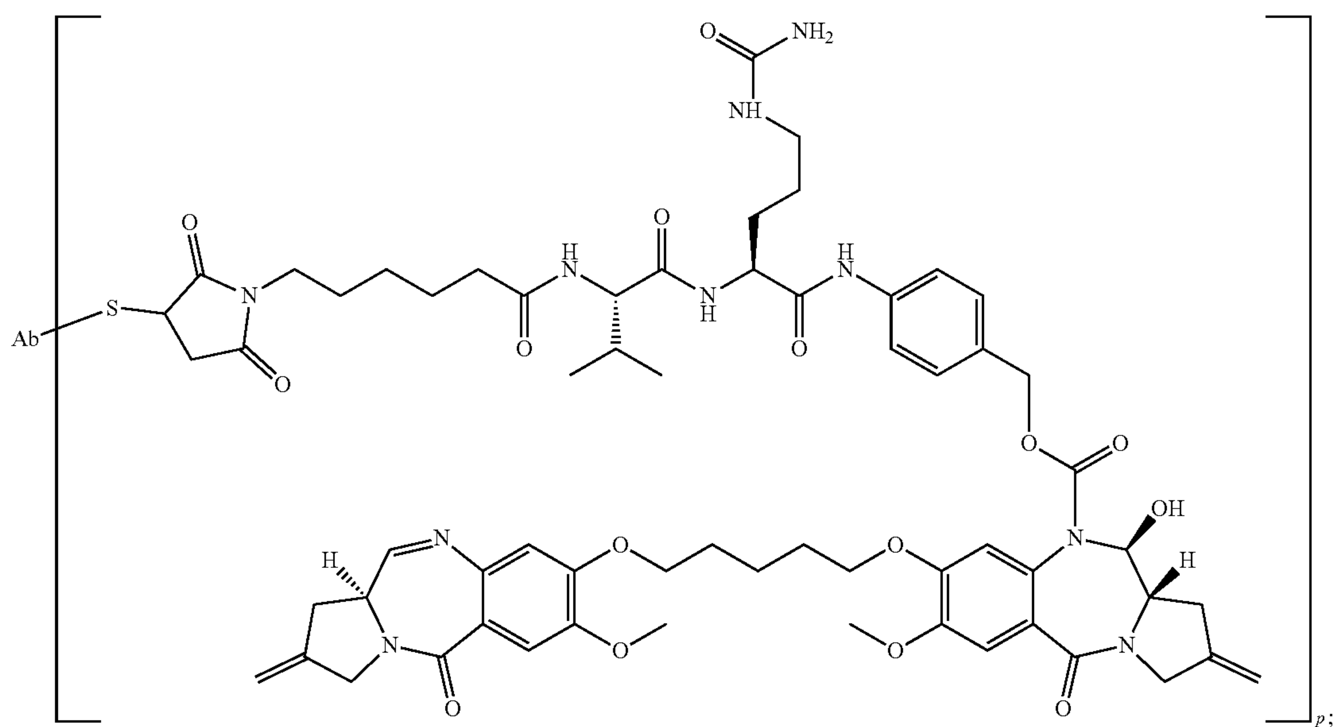
PBD dimer-val-cit-PAB-Ab
