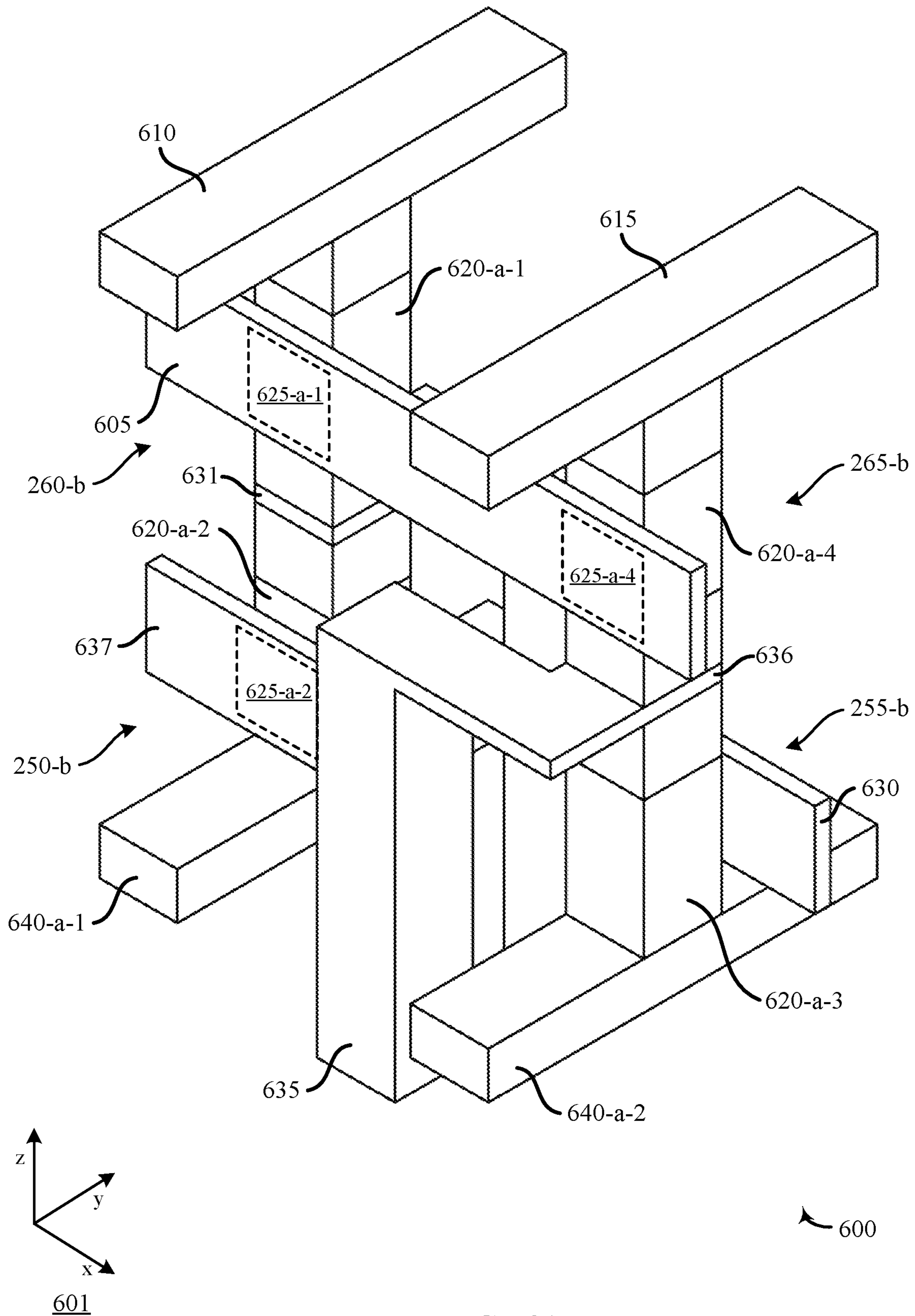
FIG. 6A
