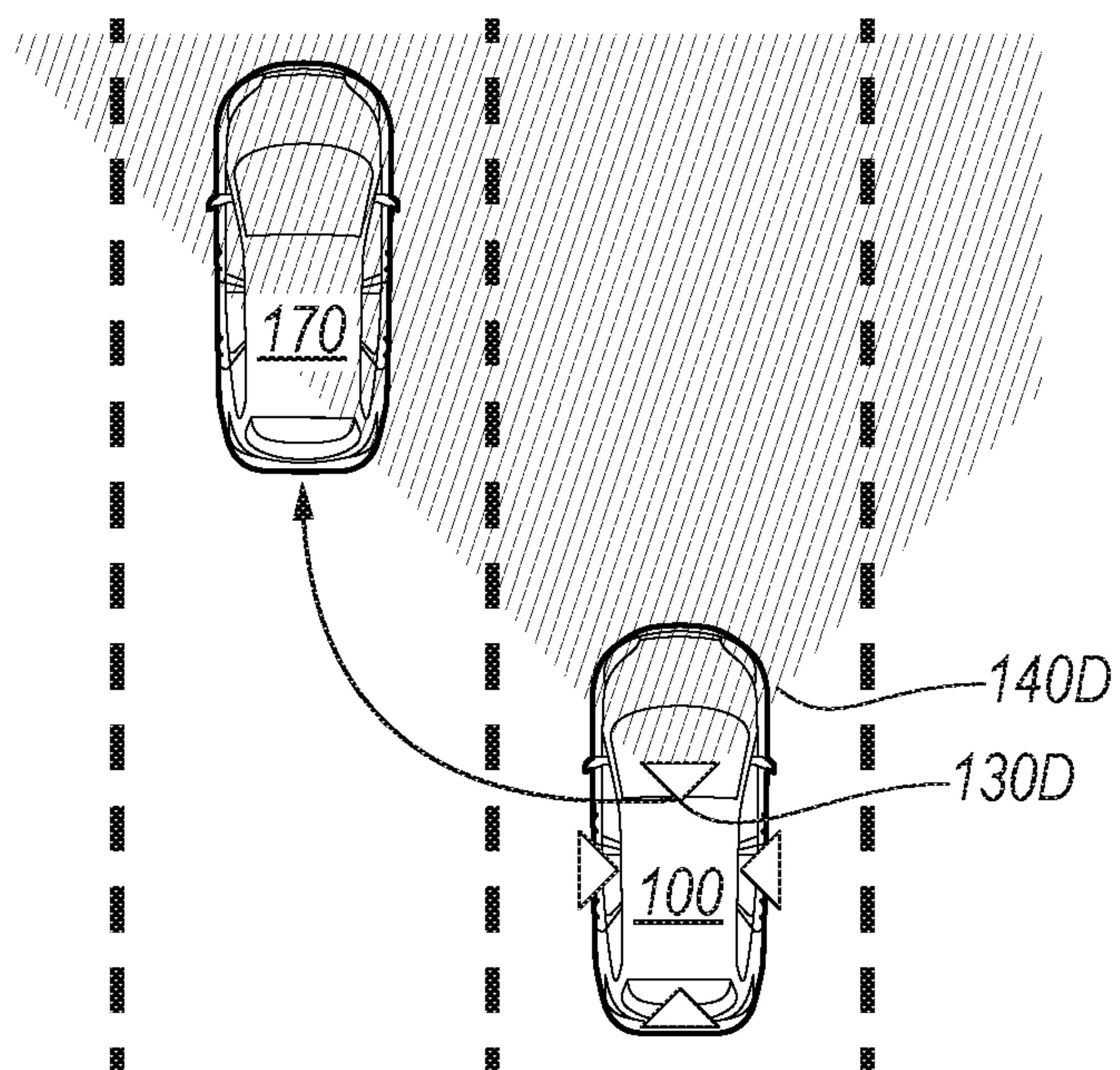
FIG. 7B
