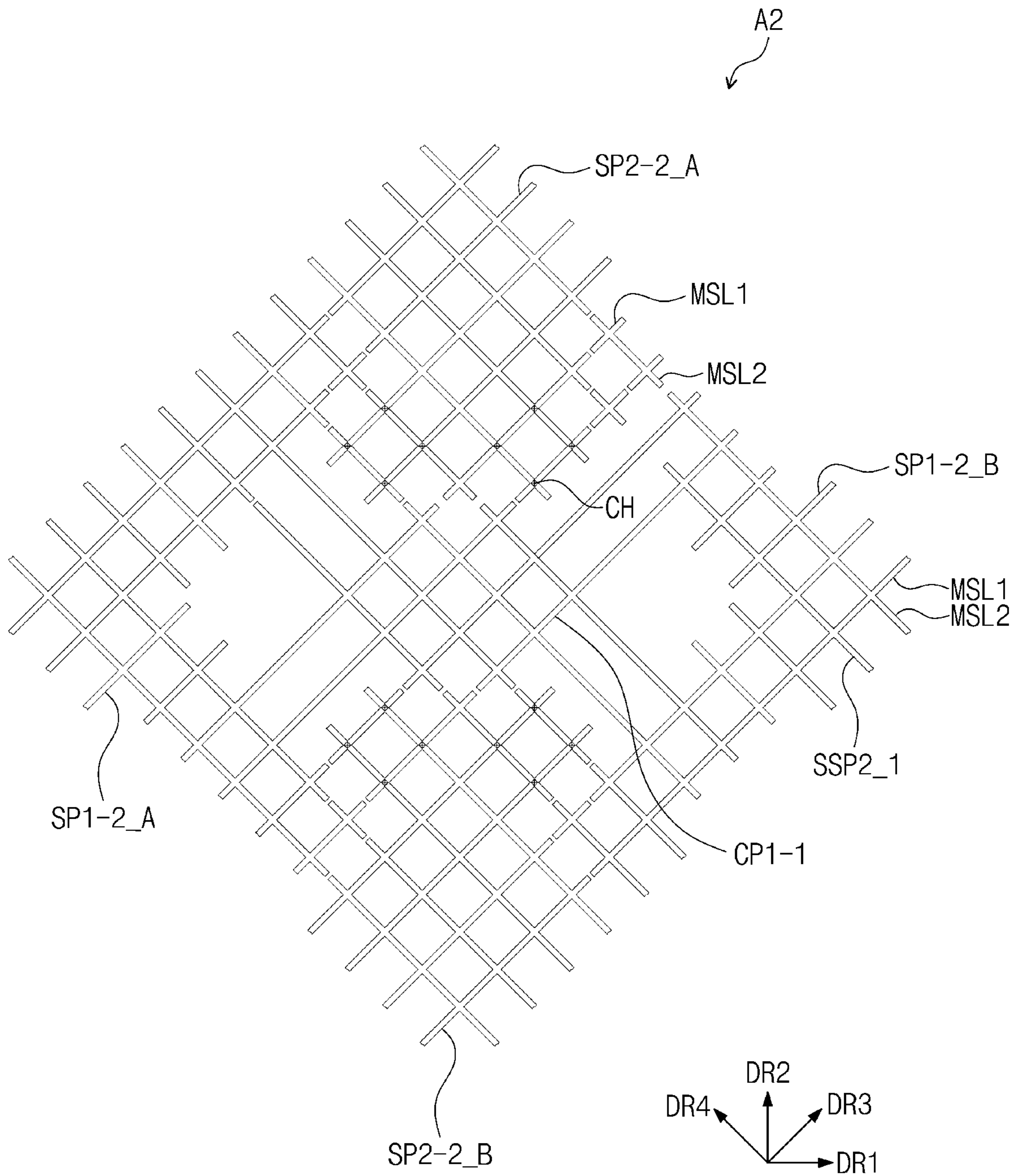
FIG. 7C
