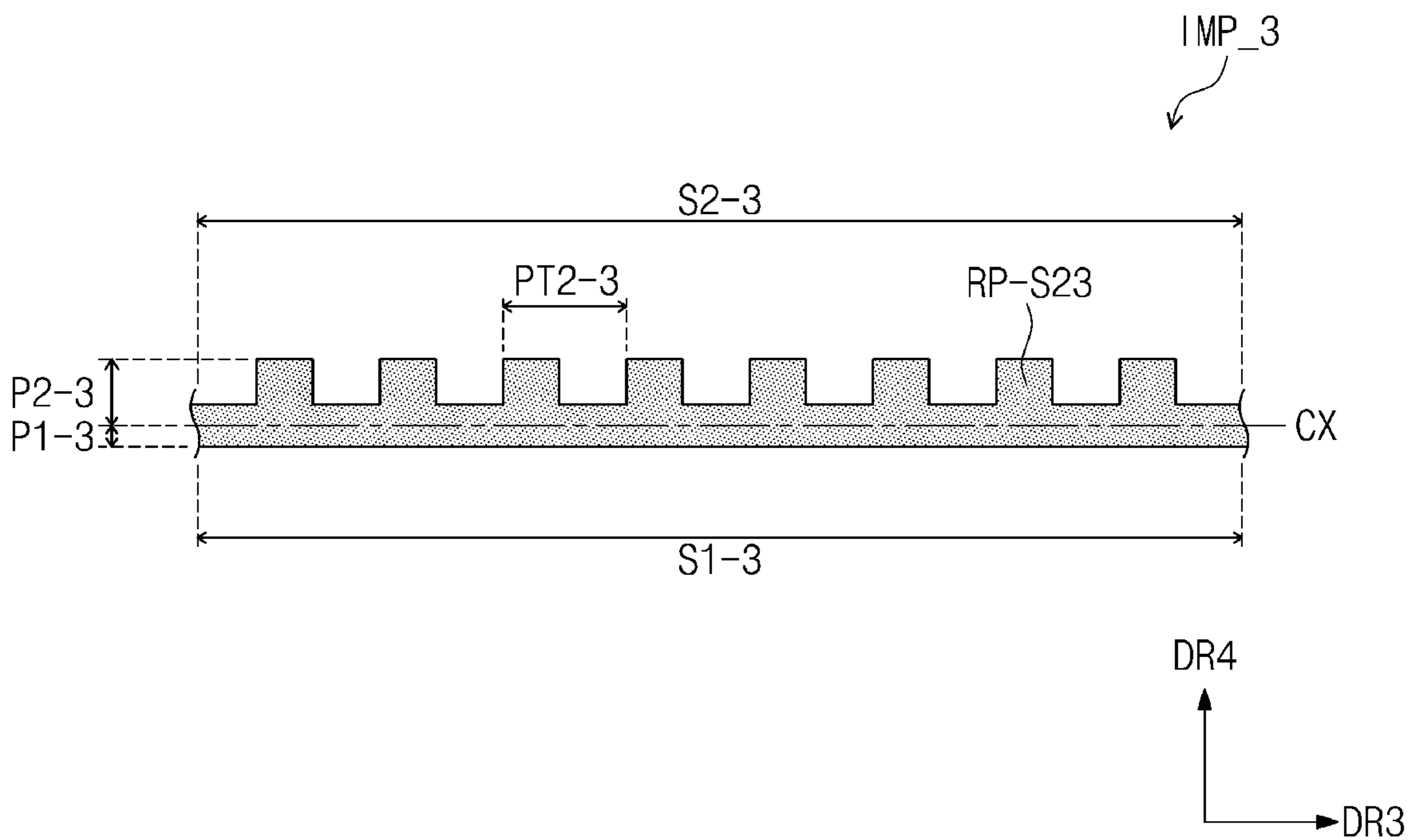
FIG. 4C
