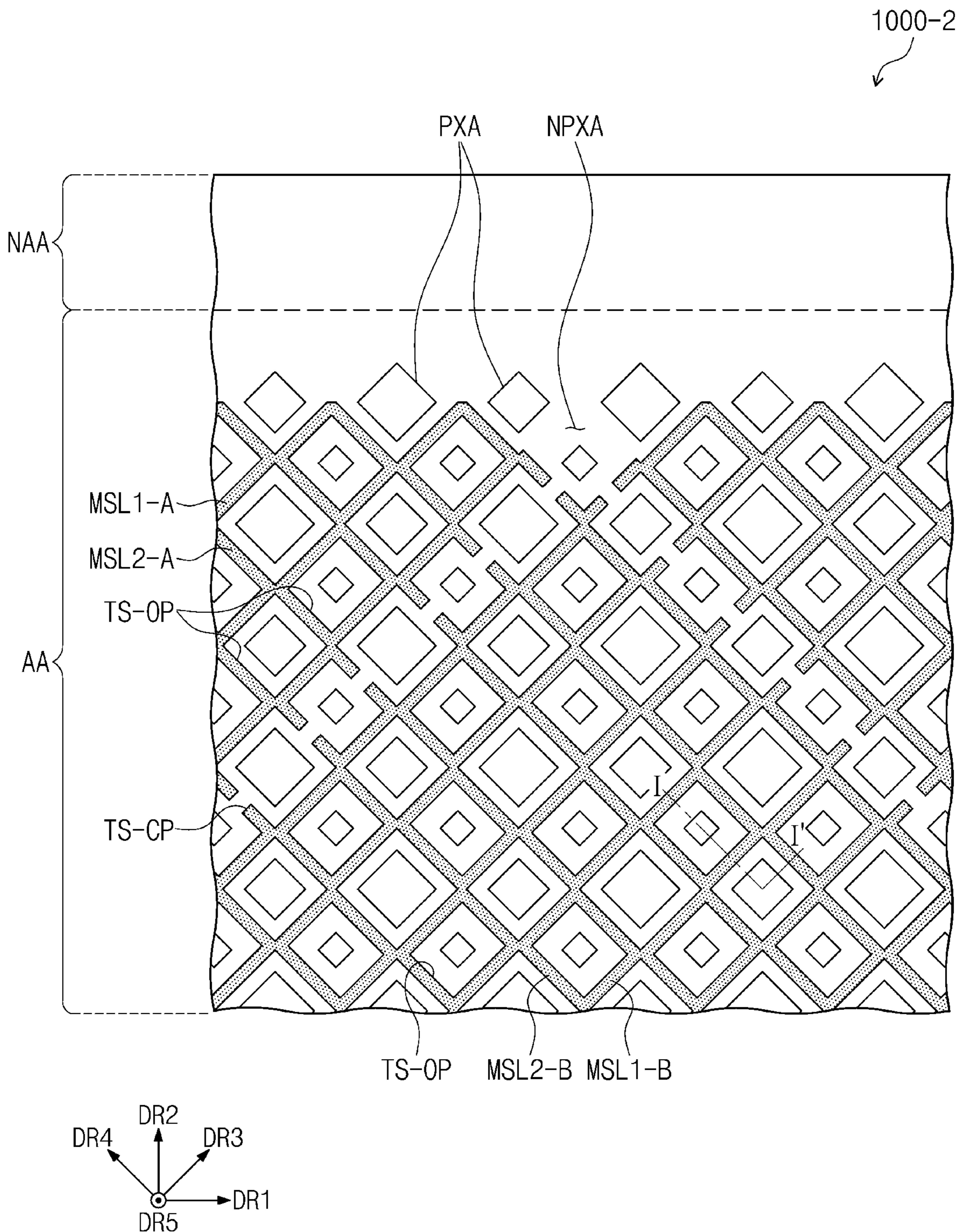
FIG. 13A
