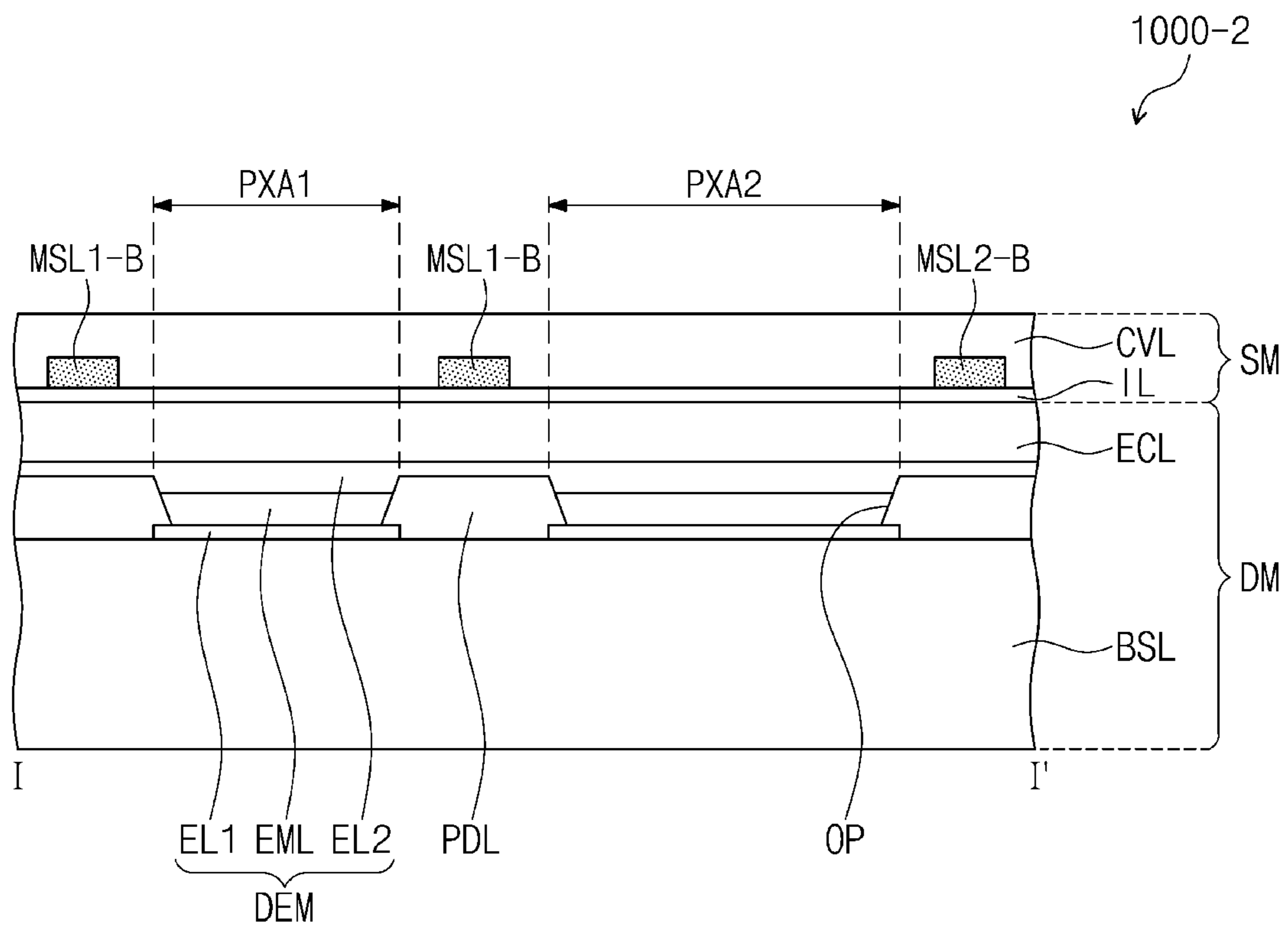
FIG. 13B
