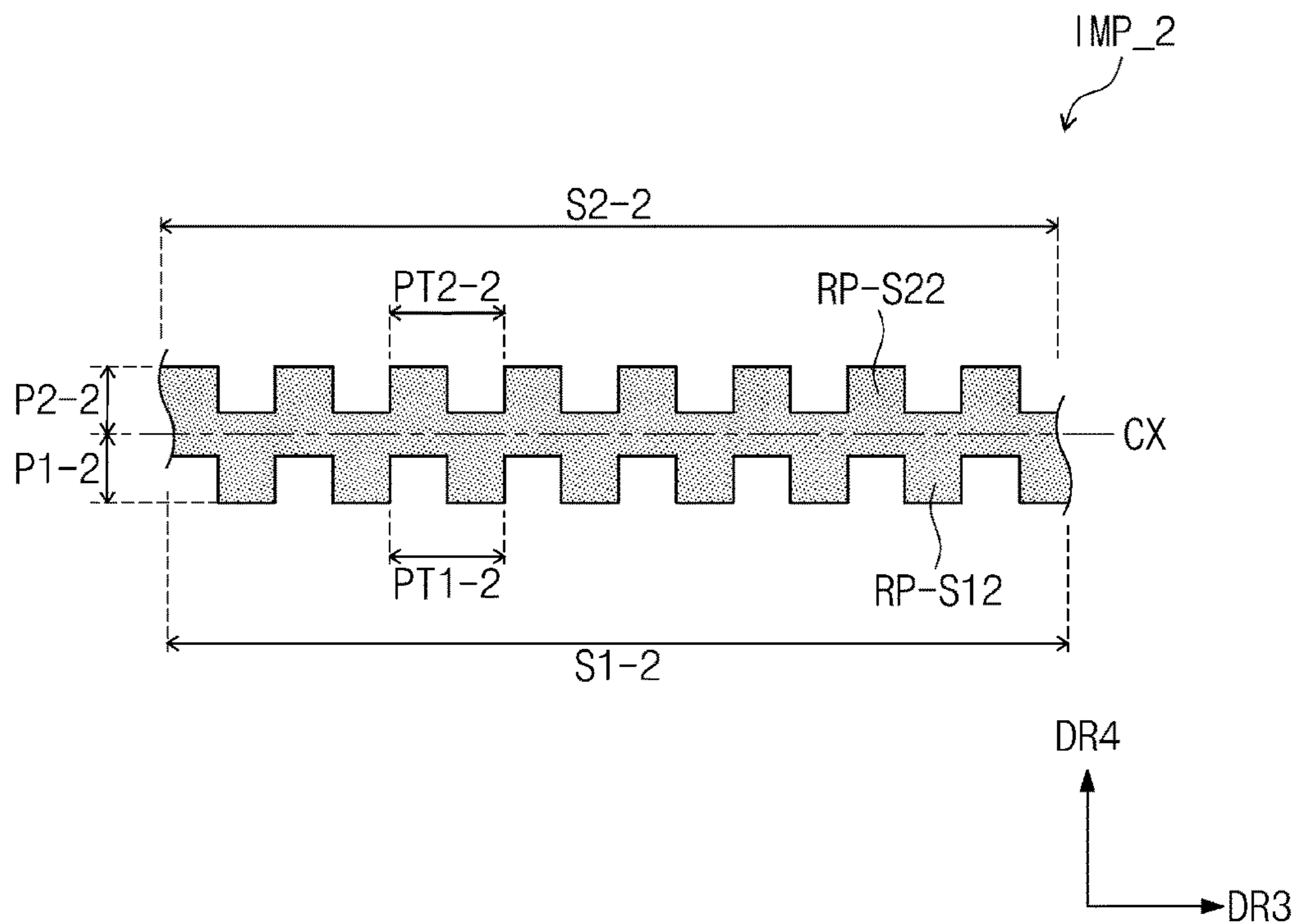
FIG. 4B
