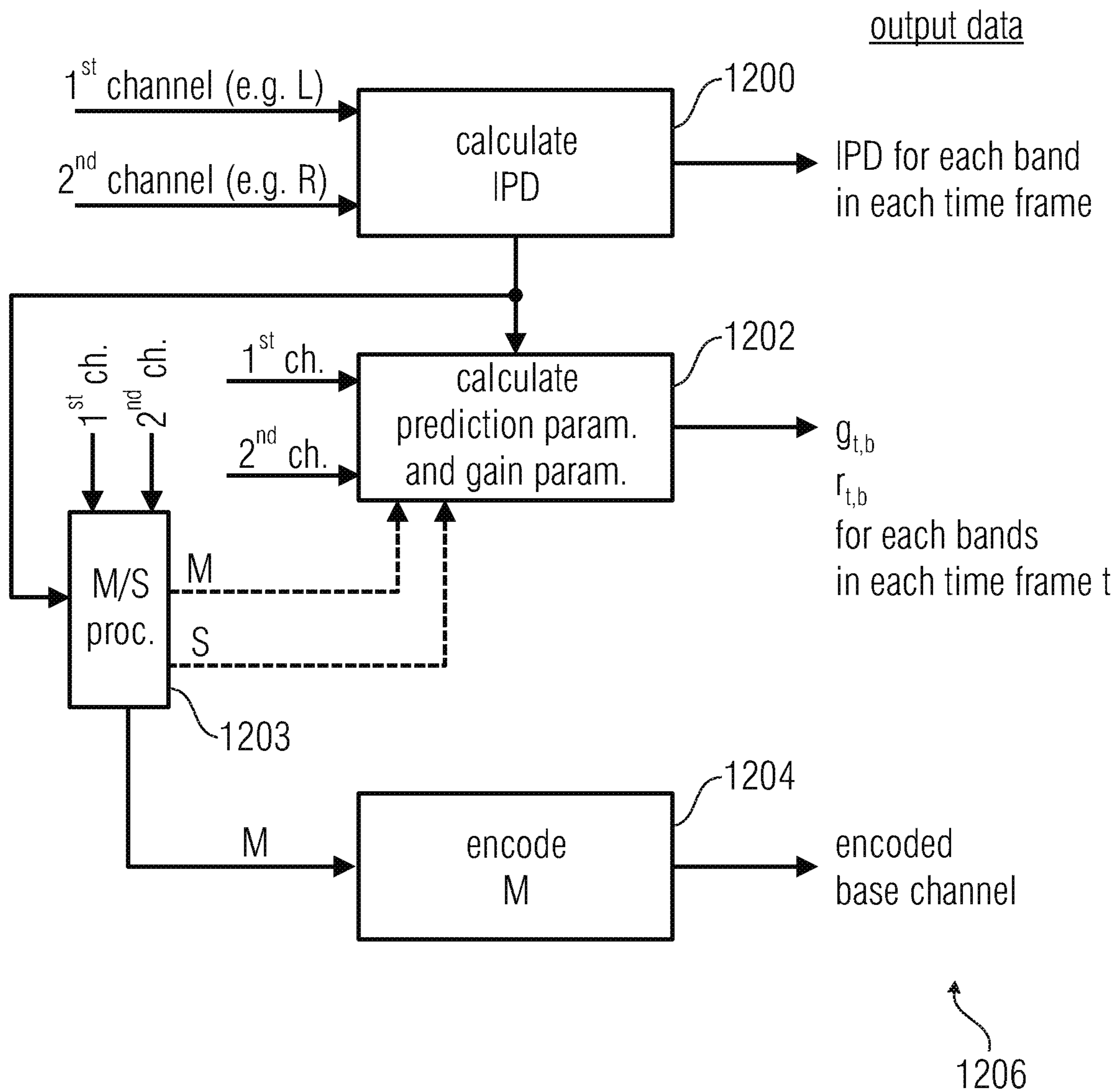
Fig. 12 (encoder side)
