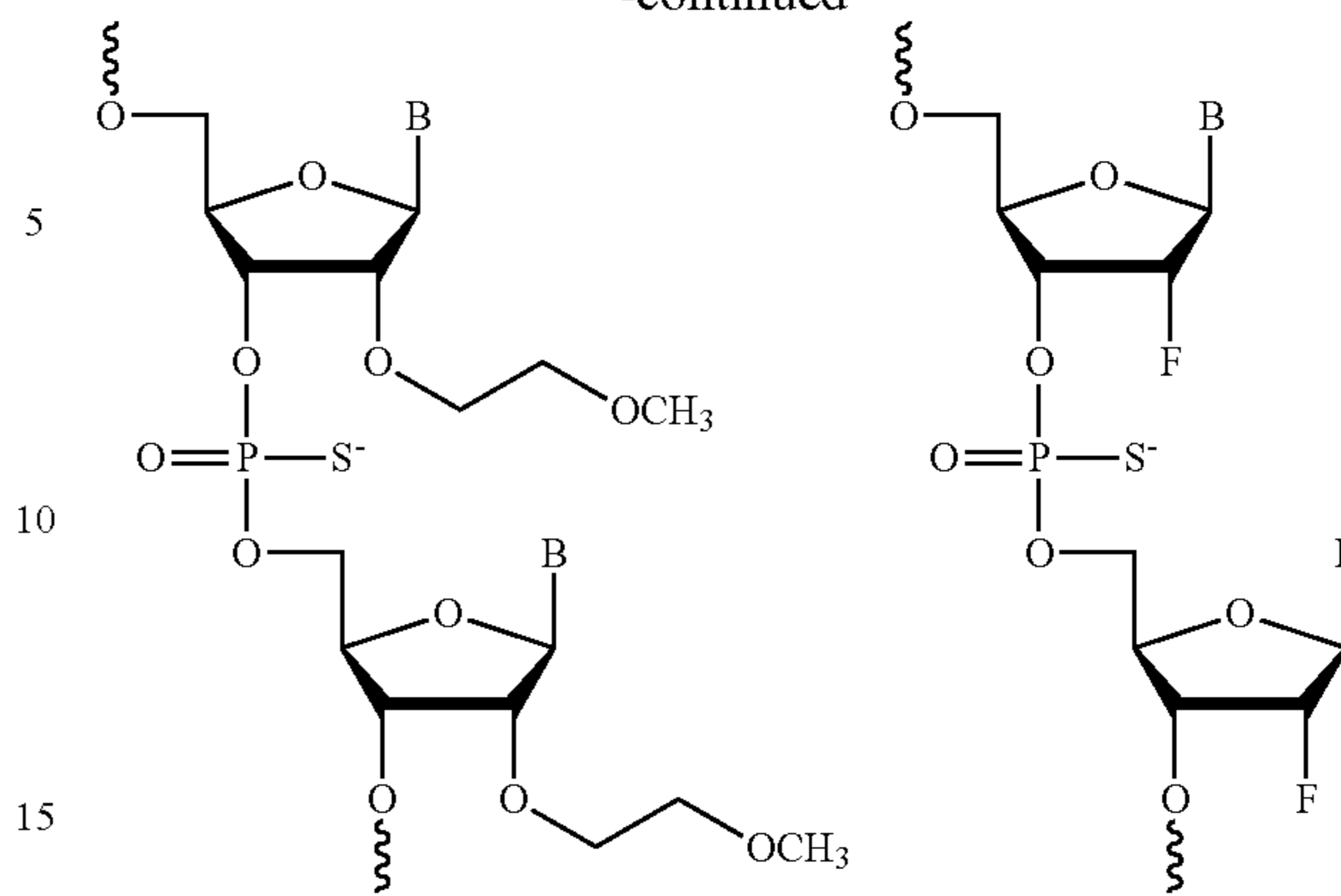
2'-O-MOE PS
