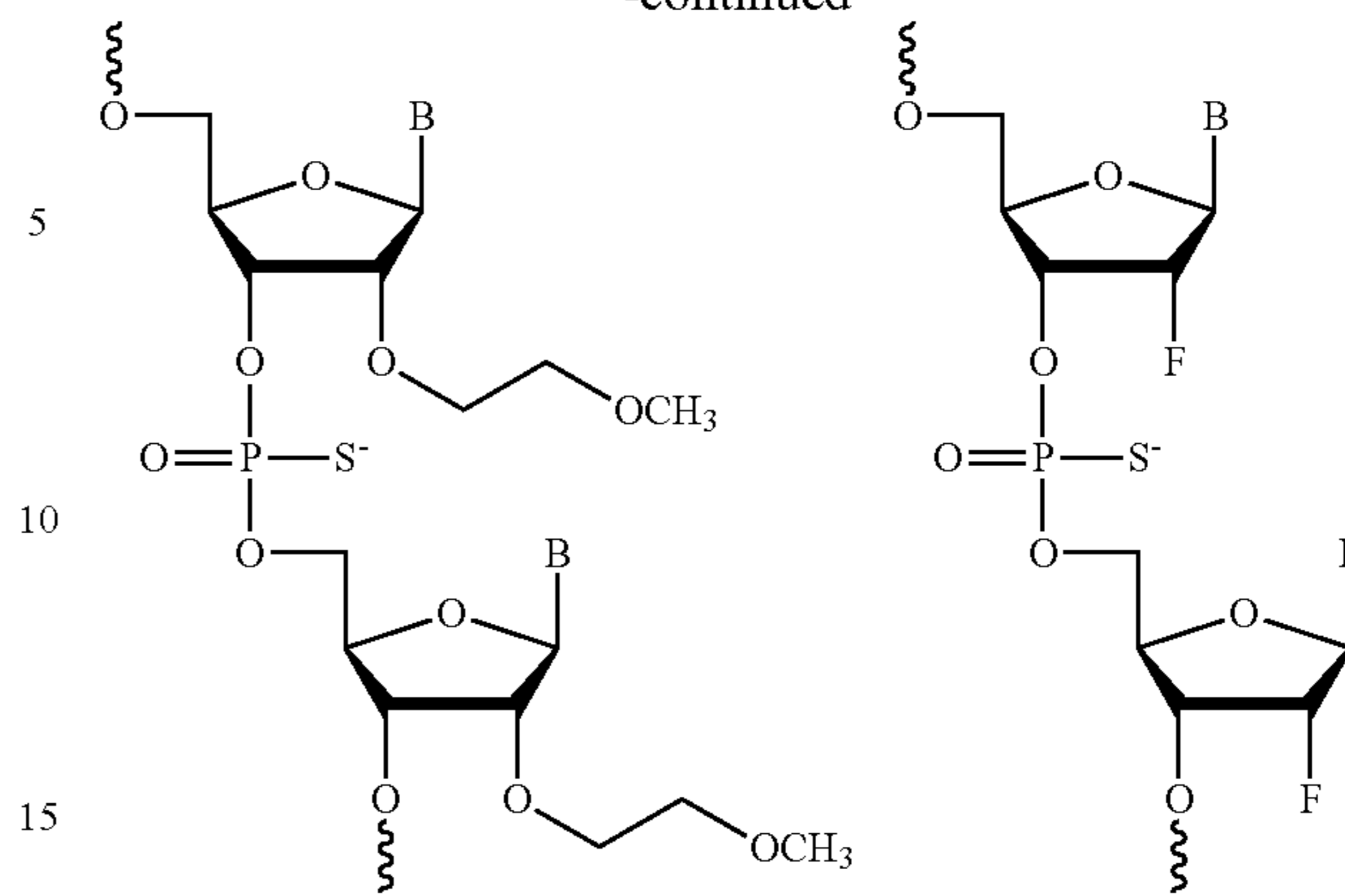
2'-O-MOE PS
