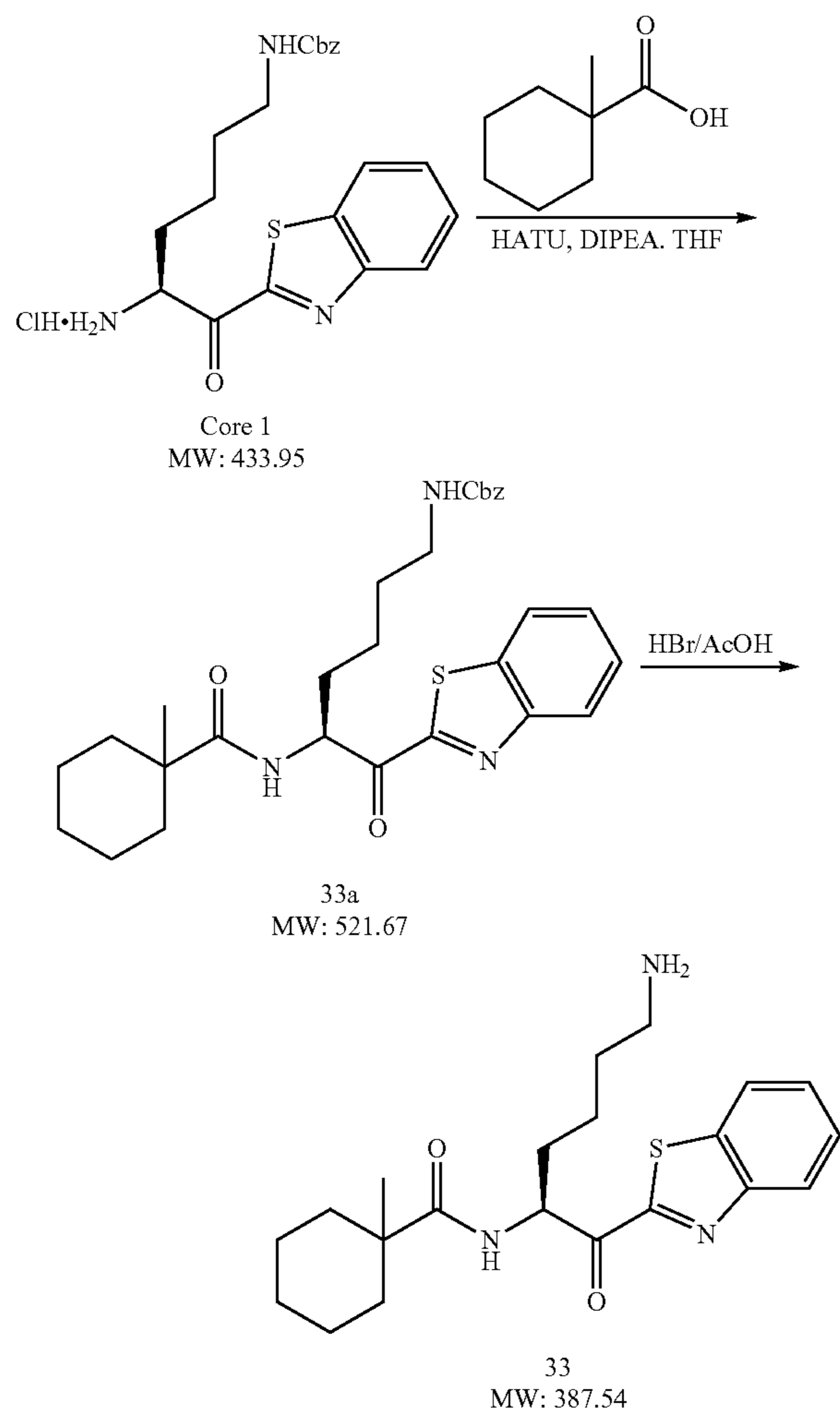
Scheme 27.
