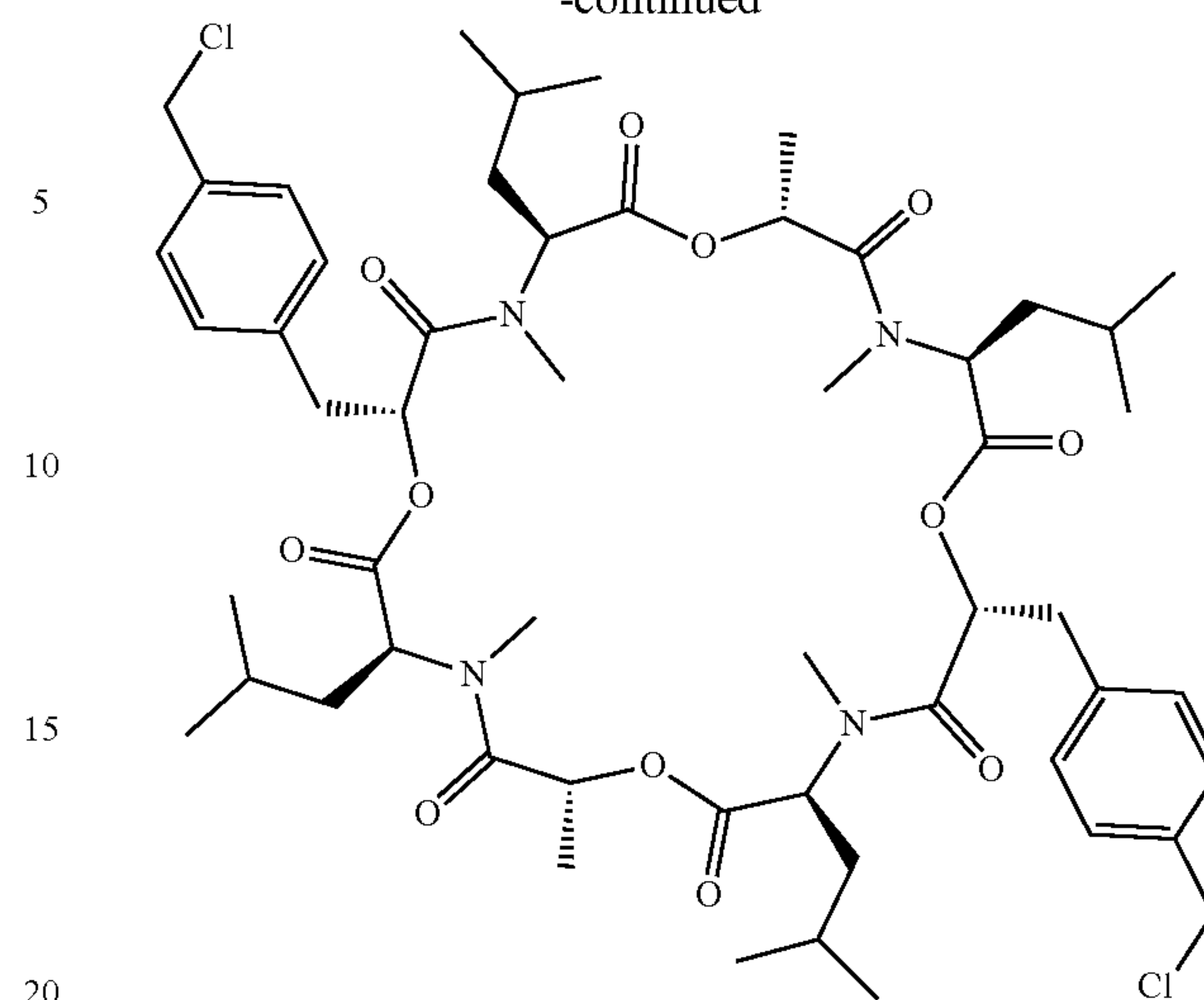
Bis-CH 2 Cl PF1022a
