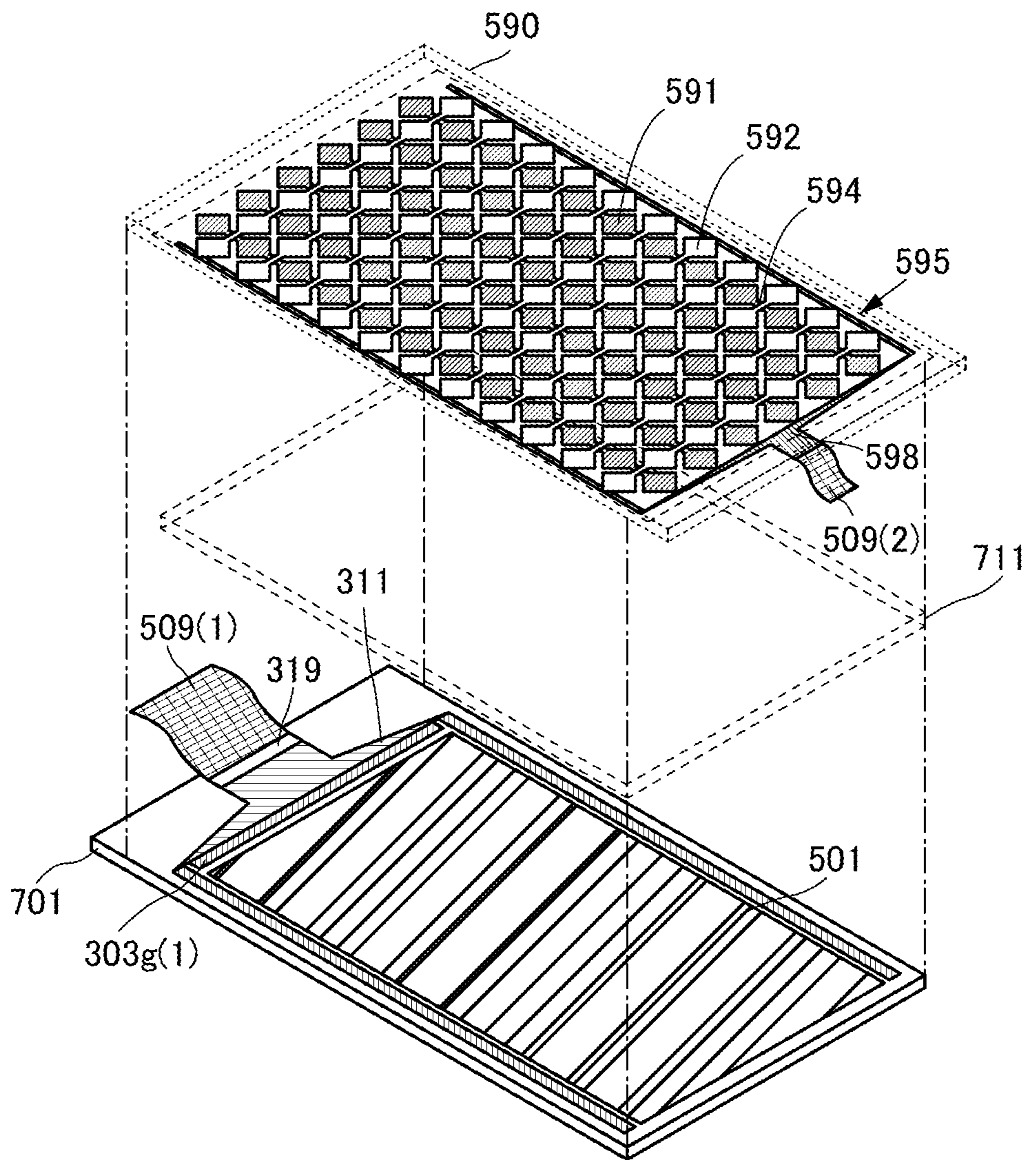
FIG. 19B
