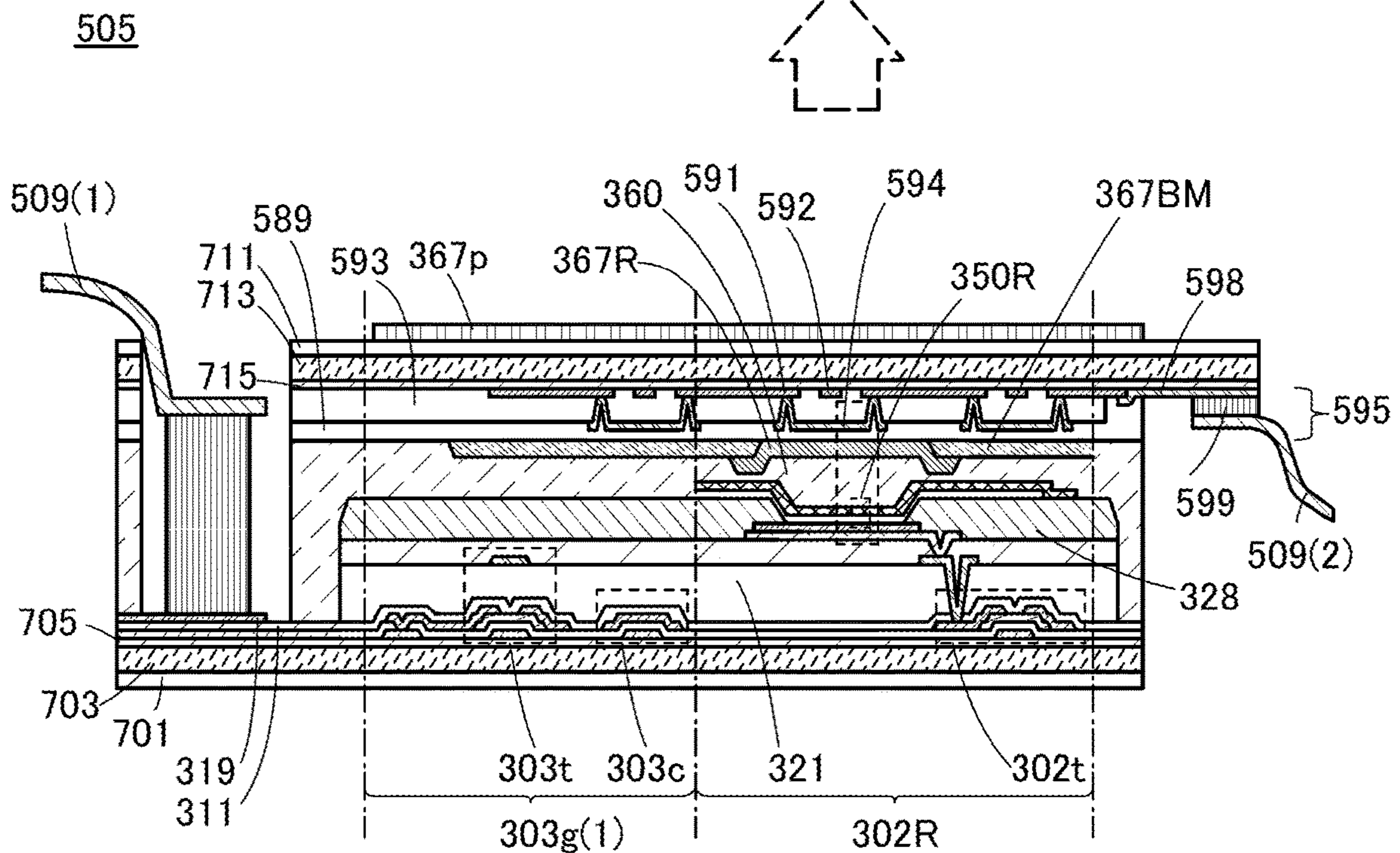
FIG. 20B
