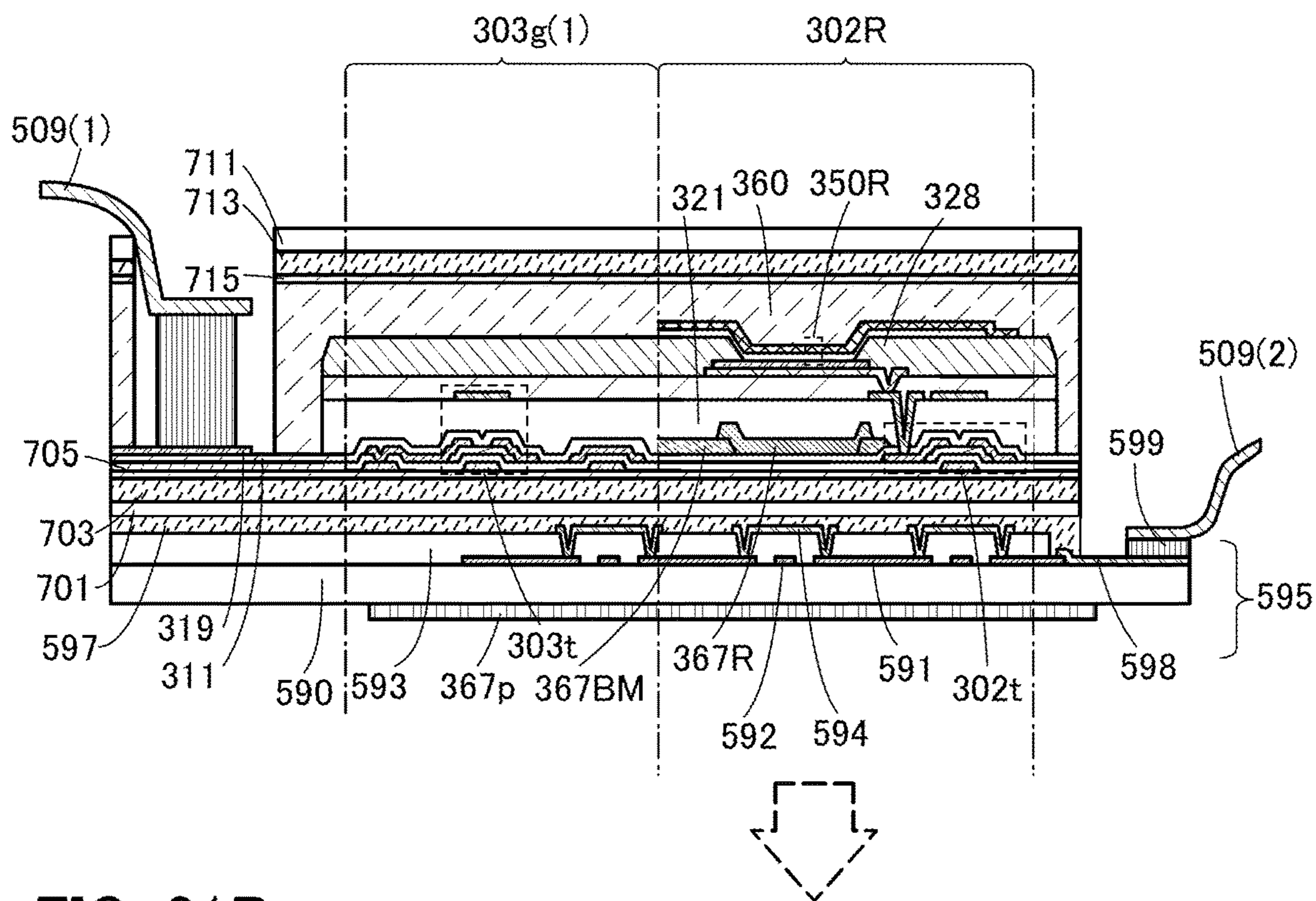
FIG. 21B
