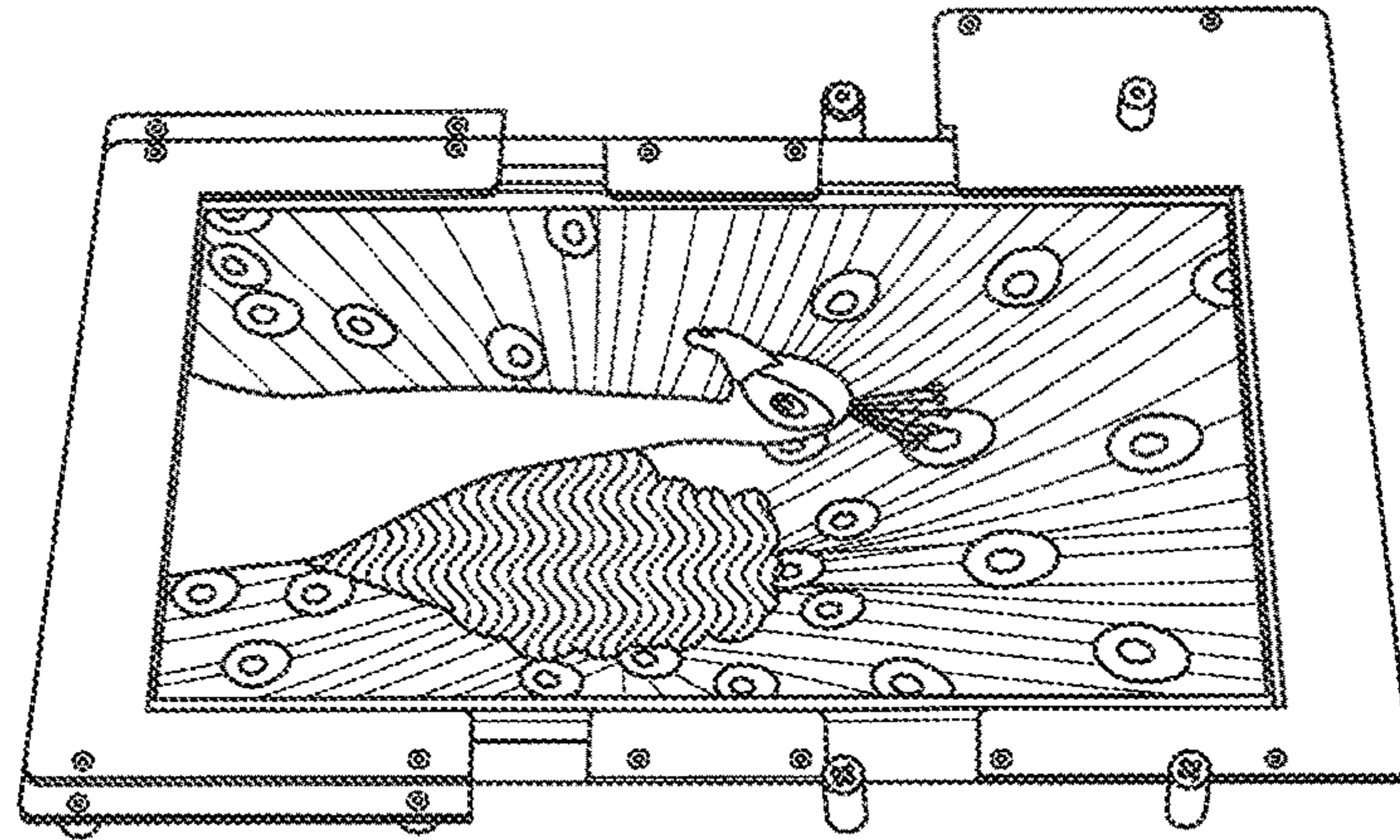
FIG. 23A
