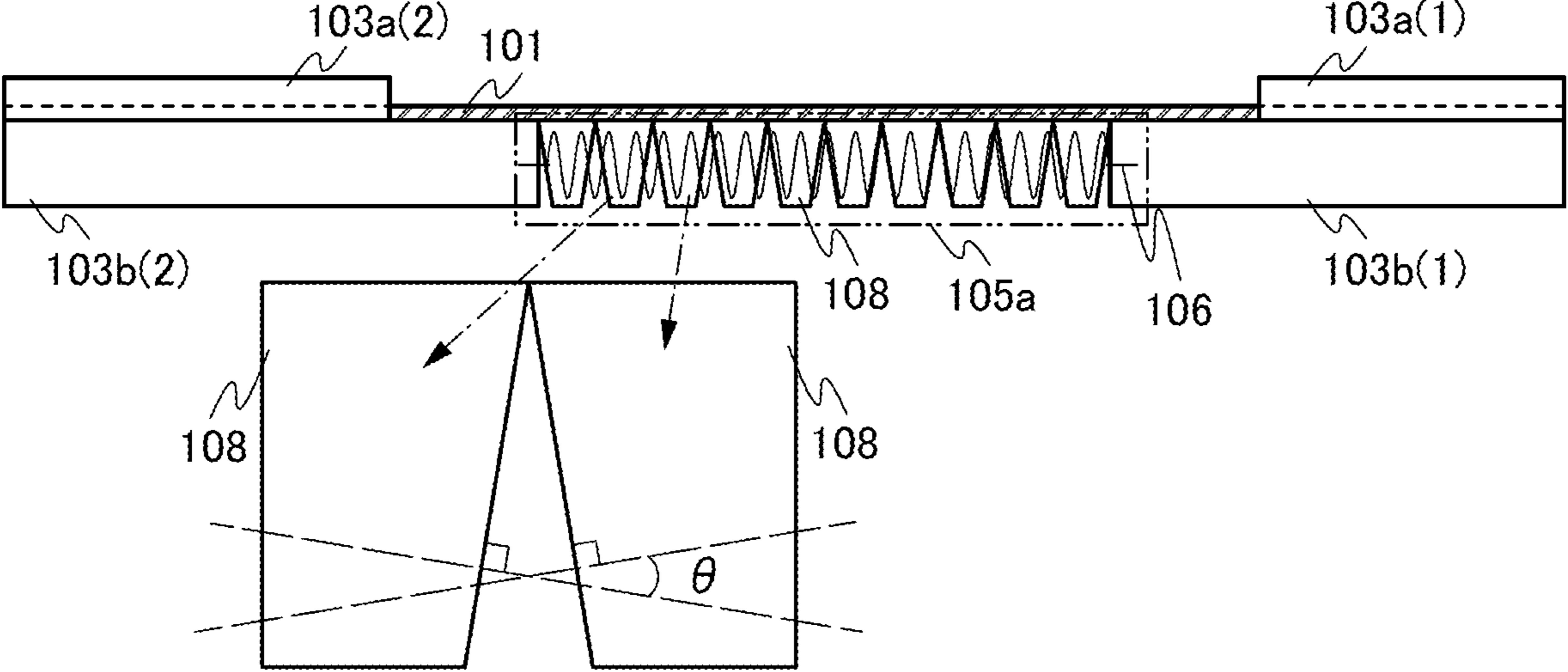
FIG. 10A
