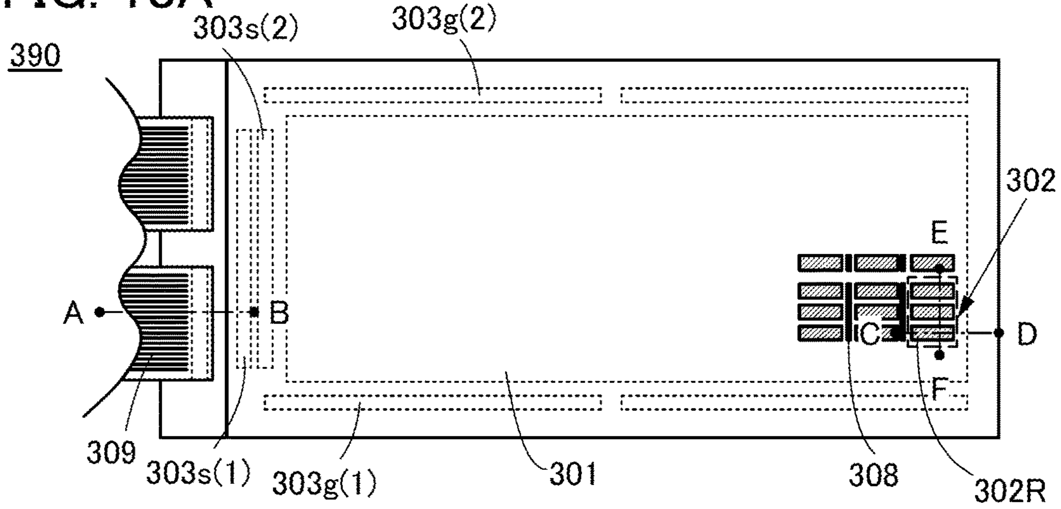
FIG. 18B
