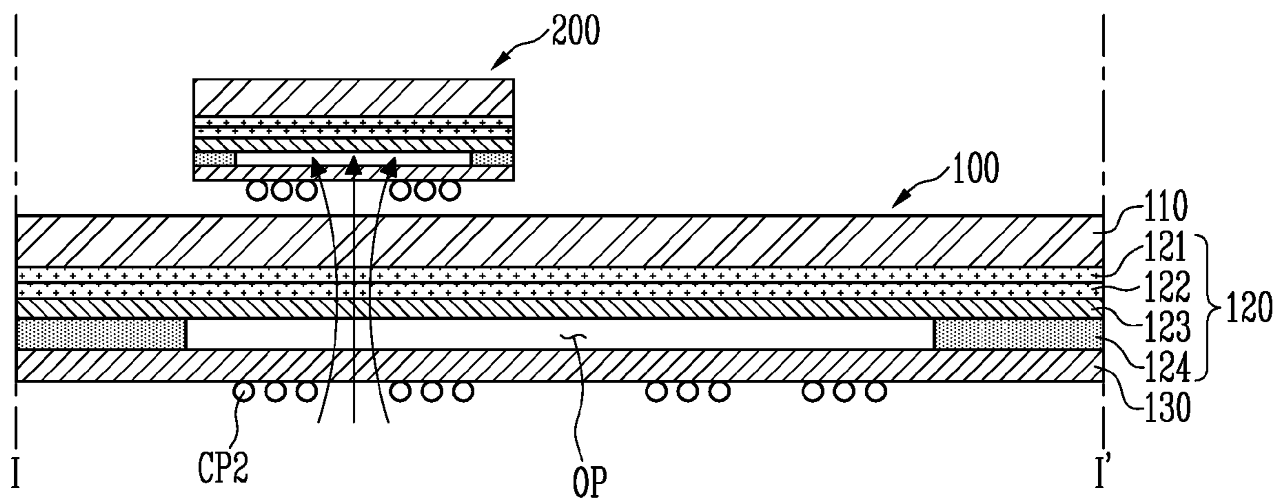
FIG. 5A
