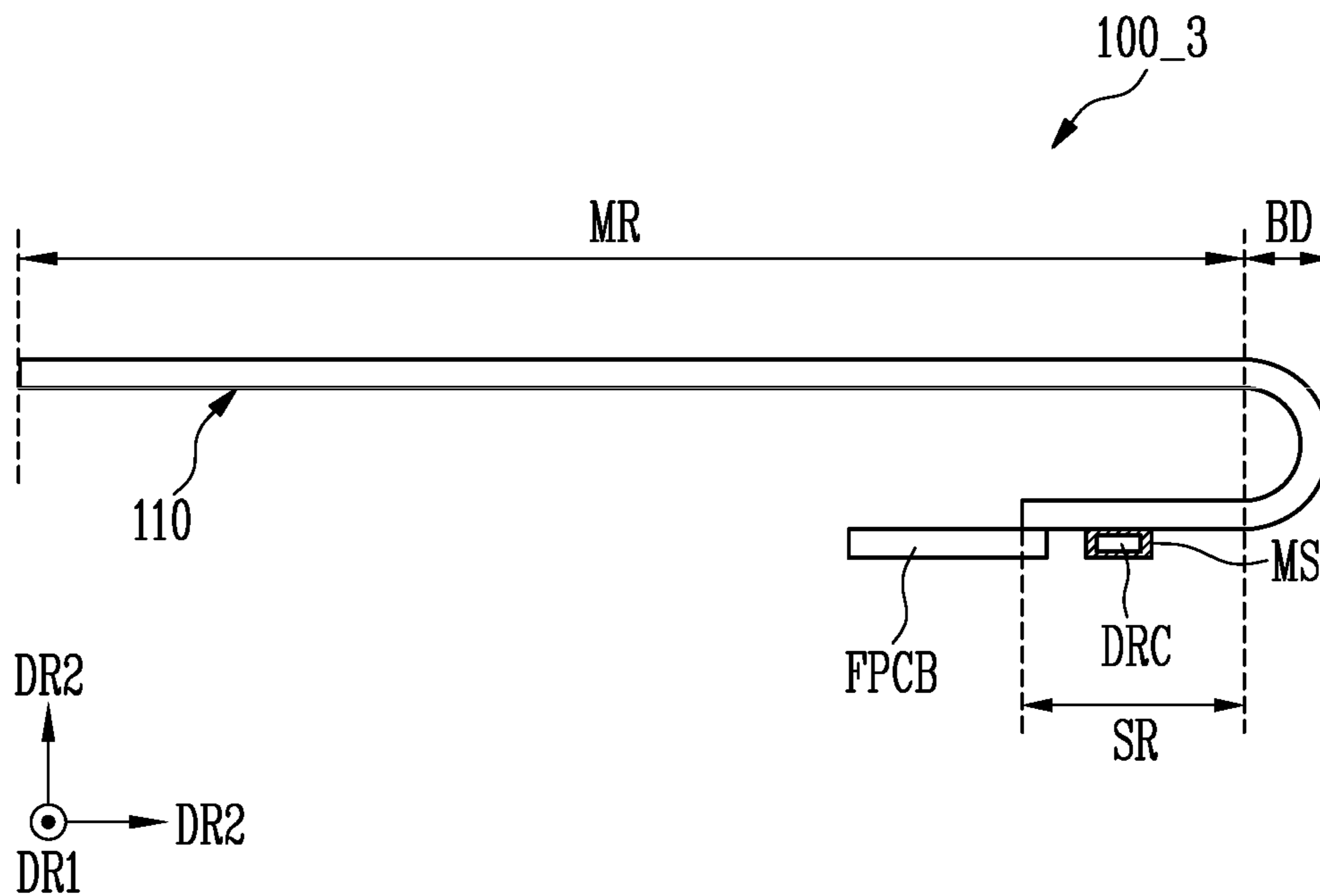
FIG. 22B
