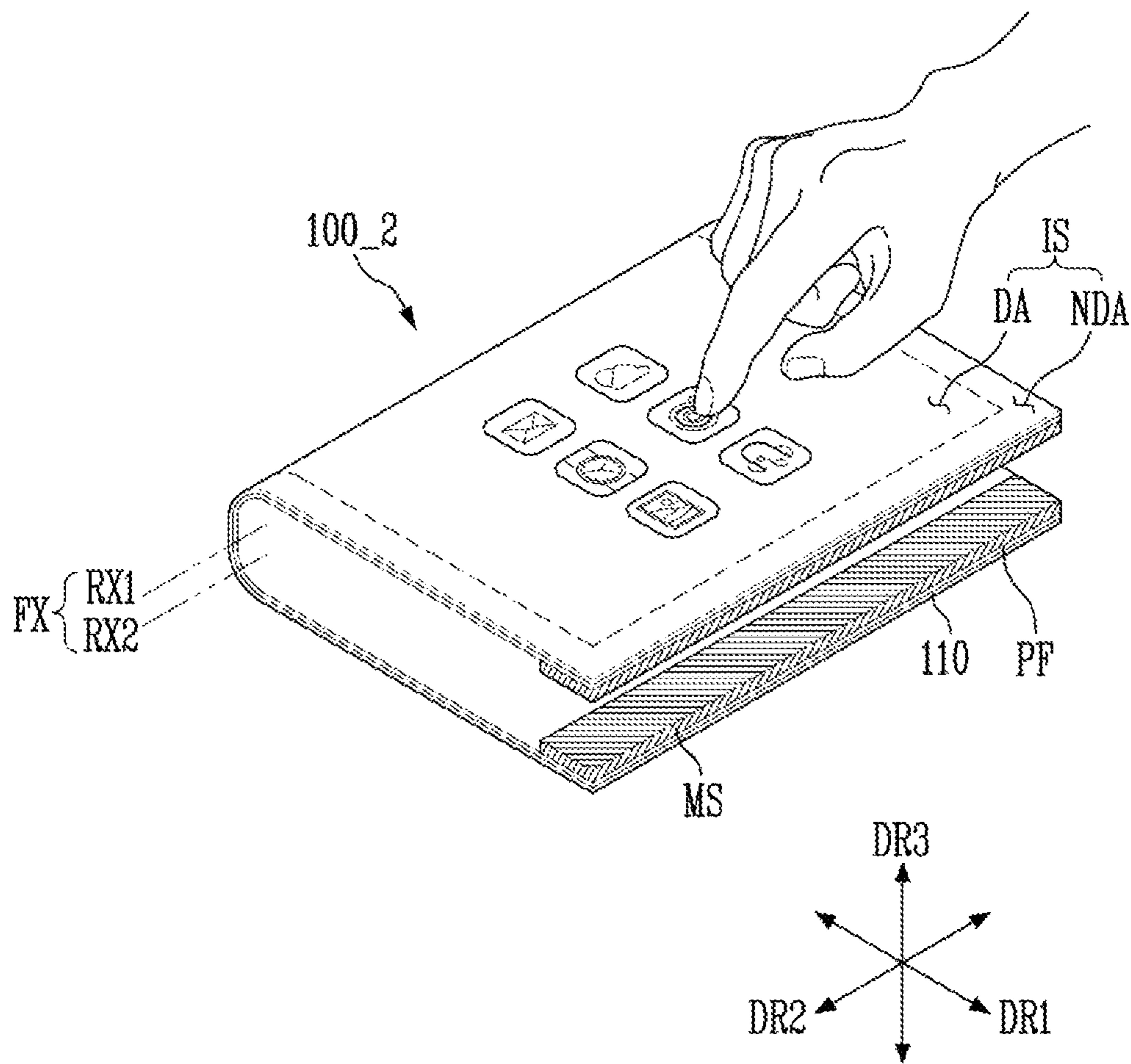
FIG. 19
