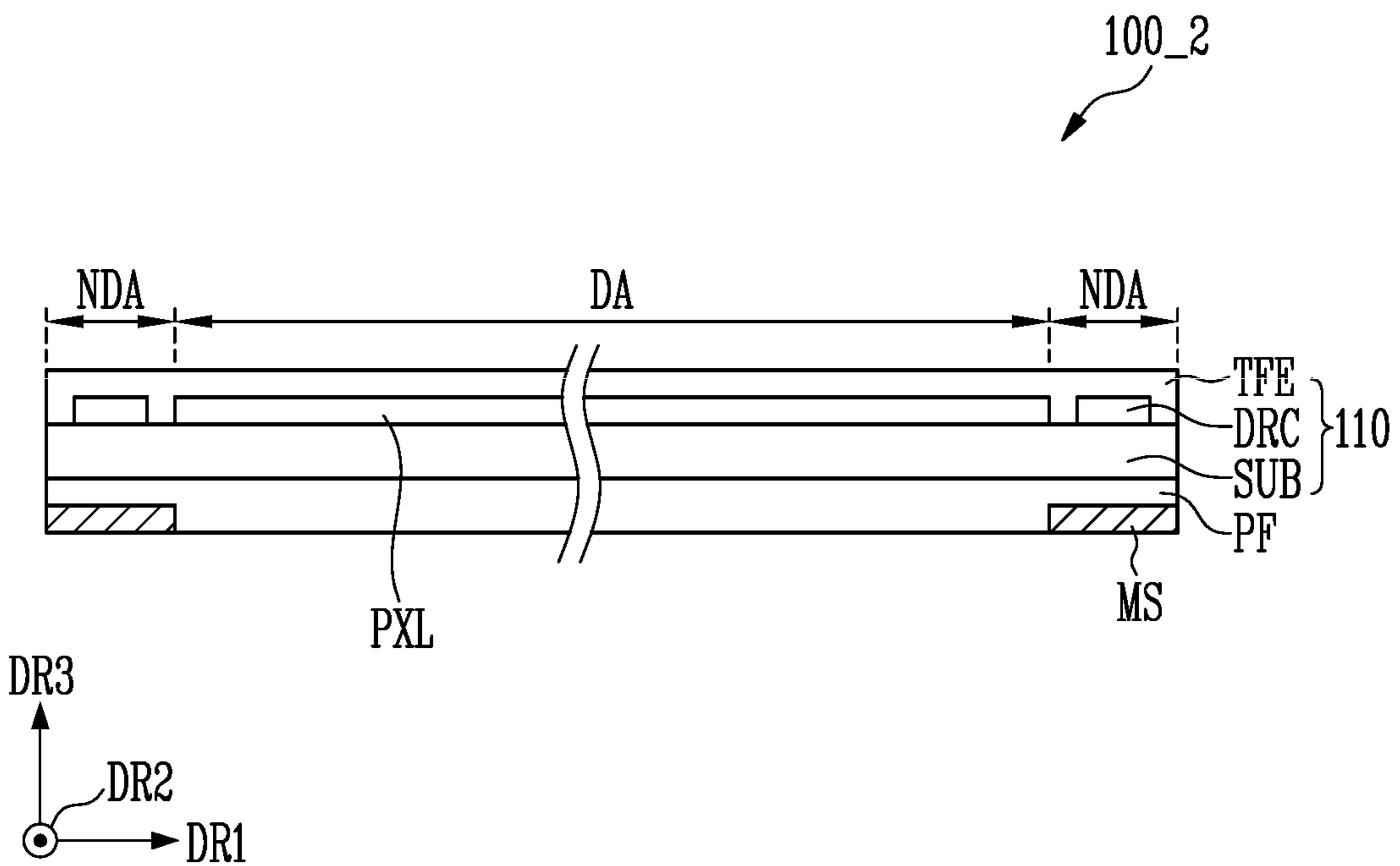
FIG. 20B
