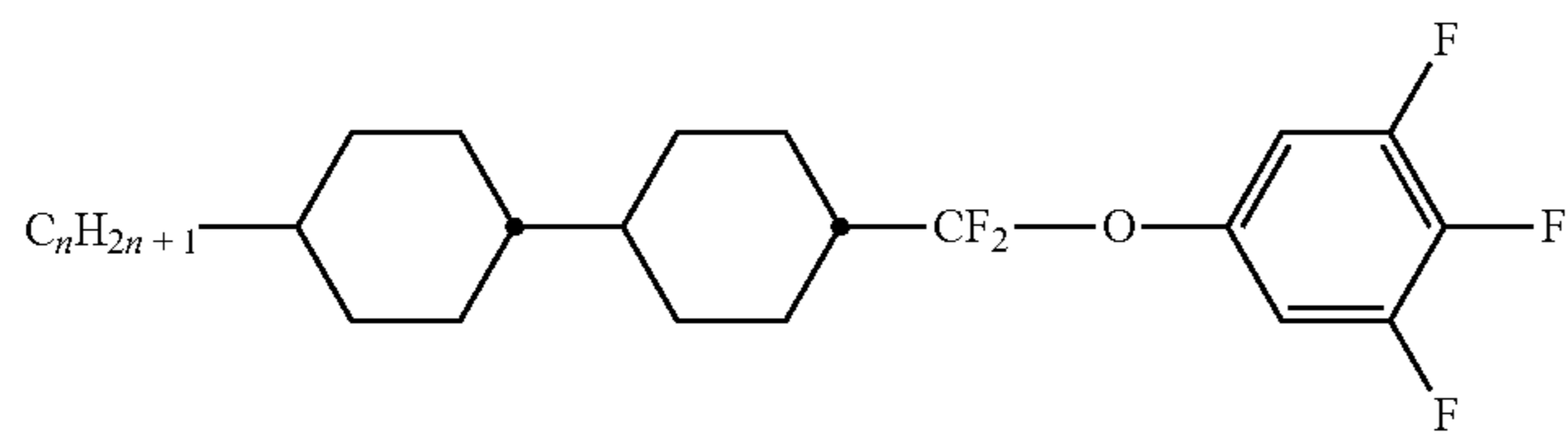
CCQU-n-F
