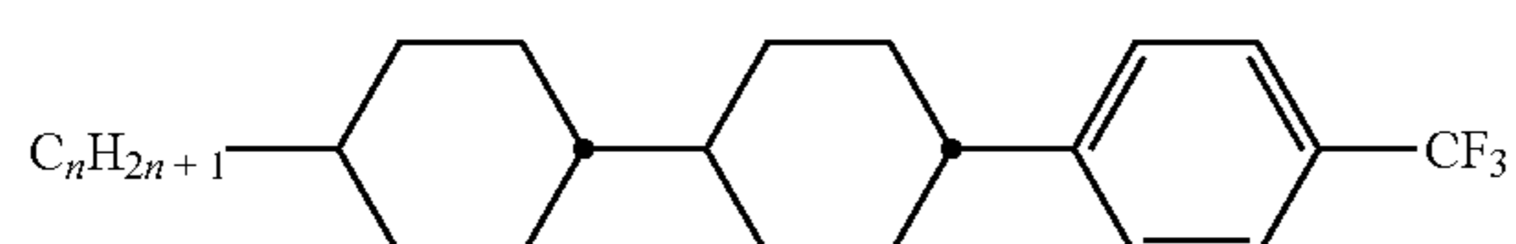
CCP-n-T
