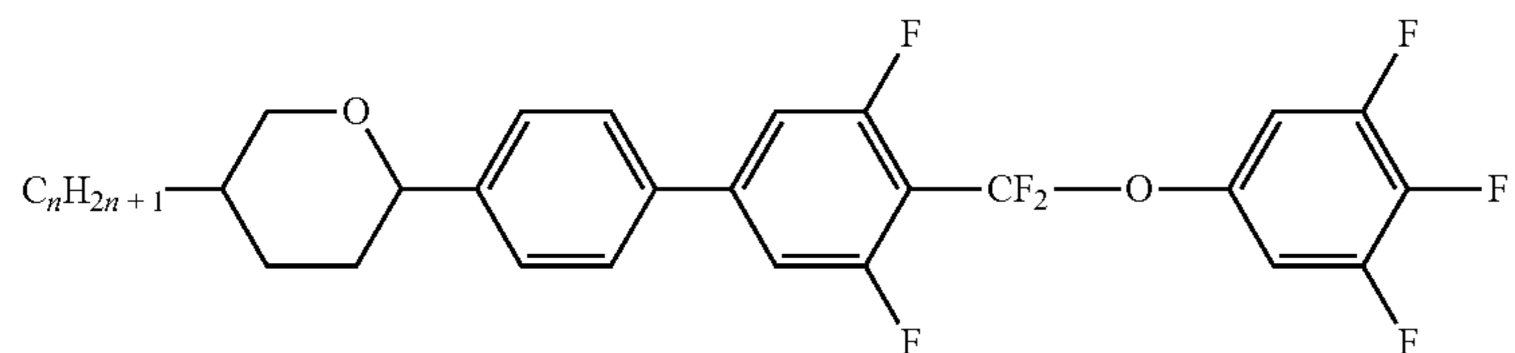
APUQU-n-F
