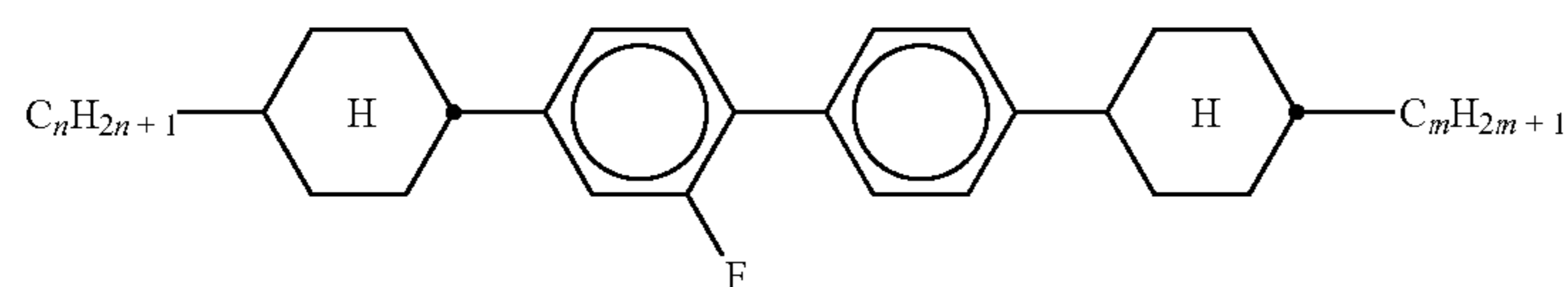
CBC-nmF
