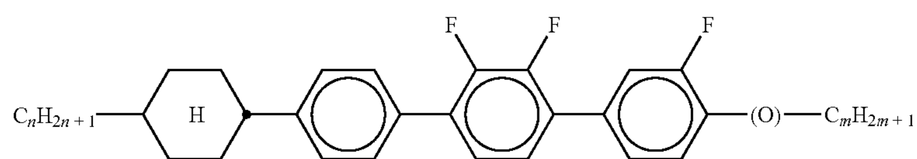
CPYG-n-(O)m
