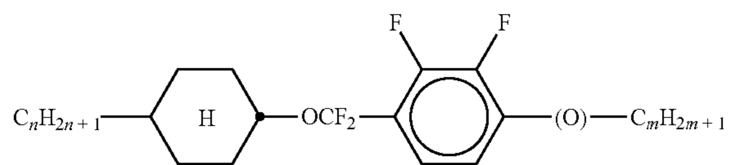
CQIY-n-(O)m
