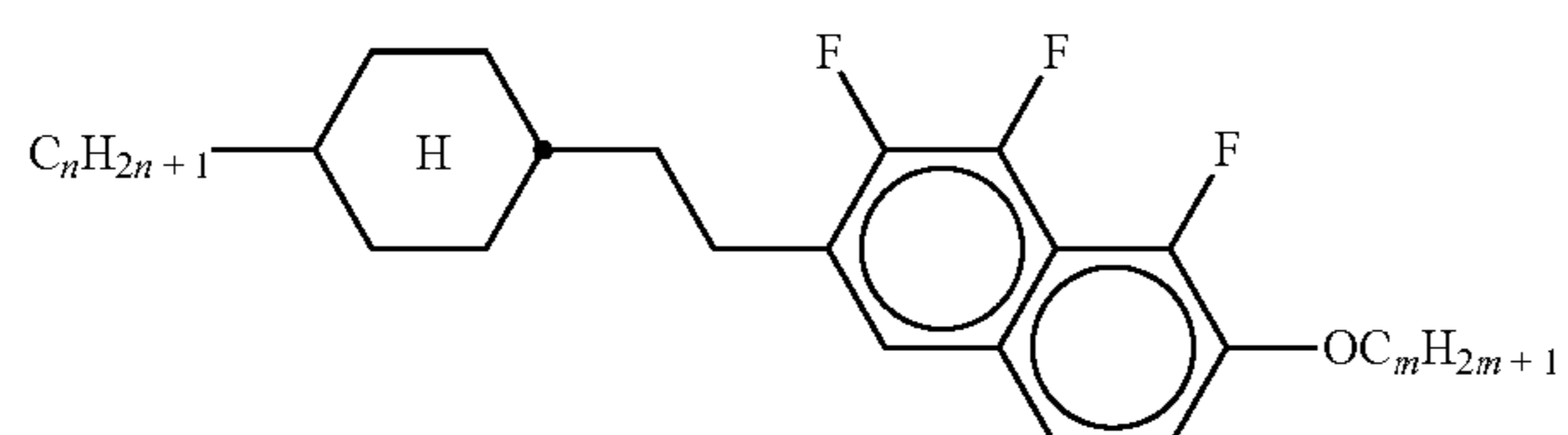
CENap-n-Om
