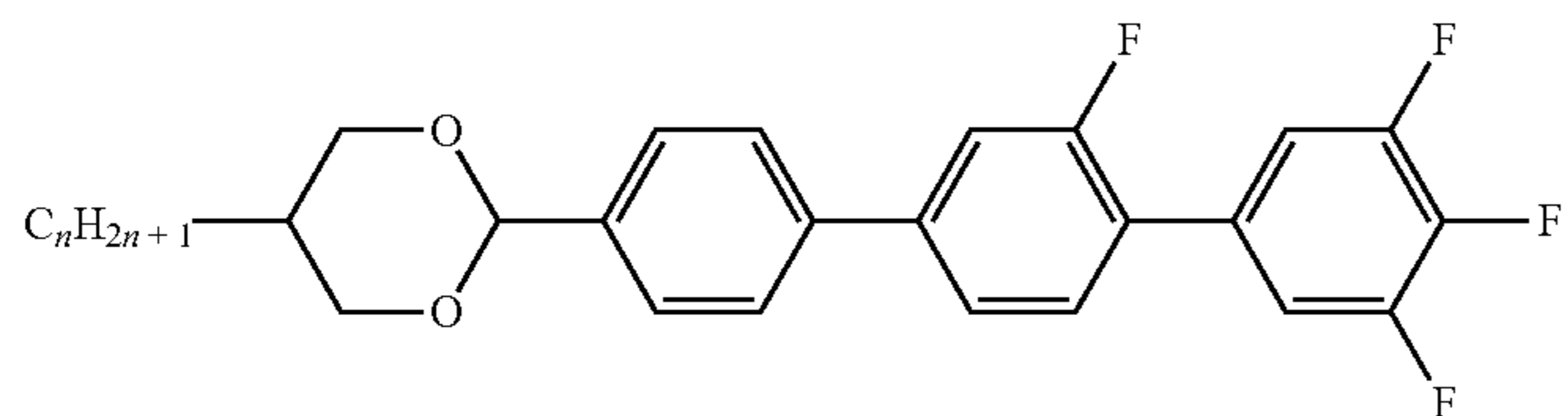
DPGU-n-F
