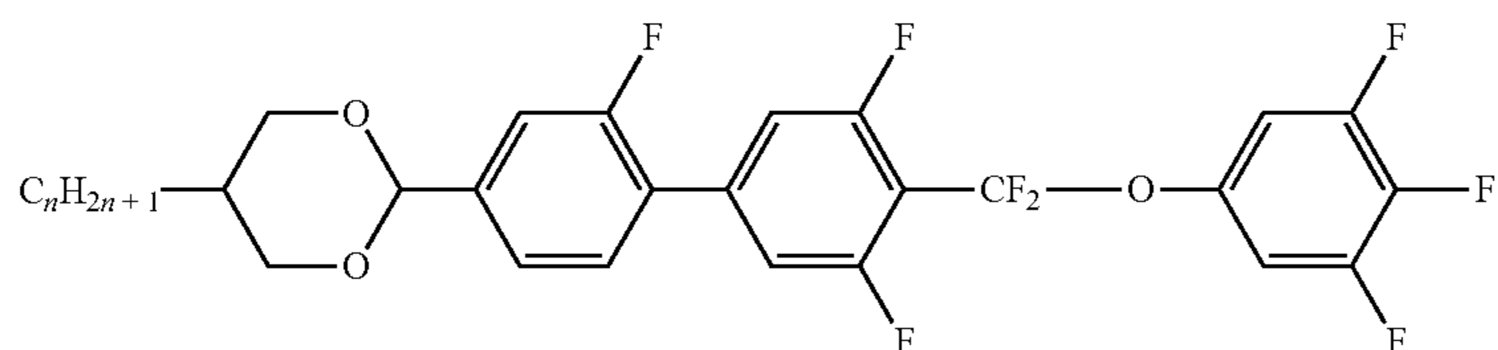
DGUQU-n-F
