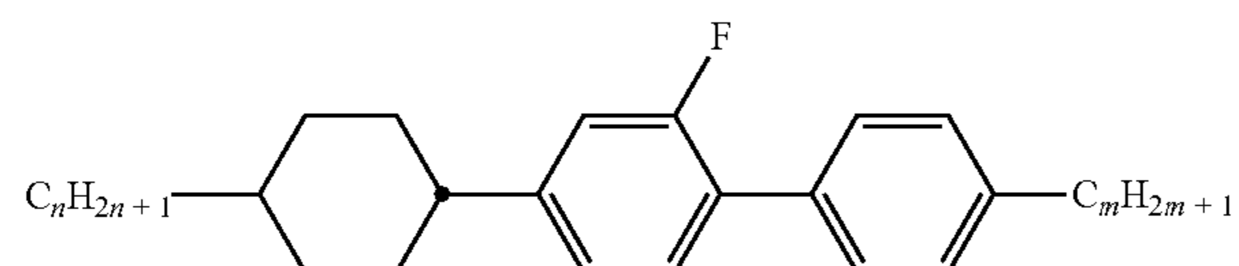
CGP-n-m
