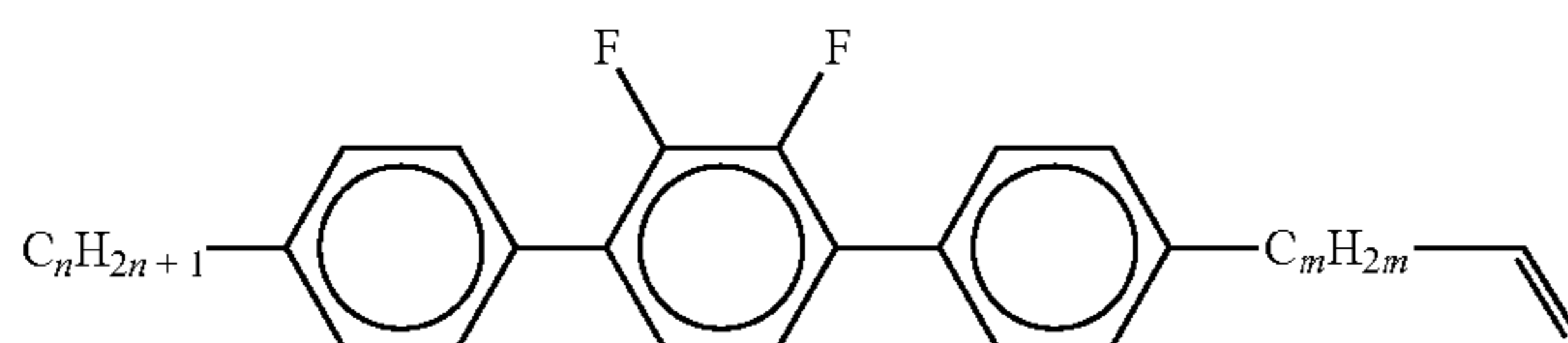
PYP-n-mV
