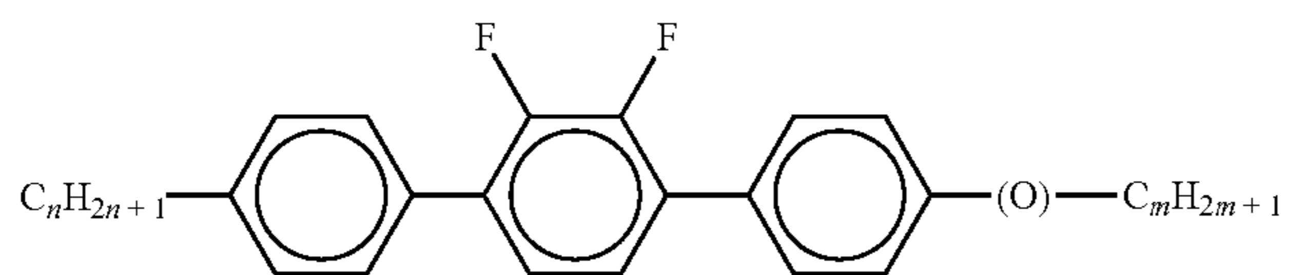
PYP-n-(O)m
