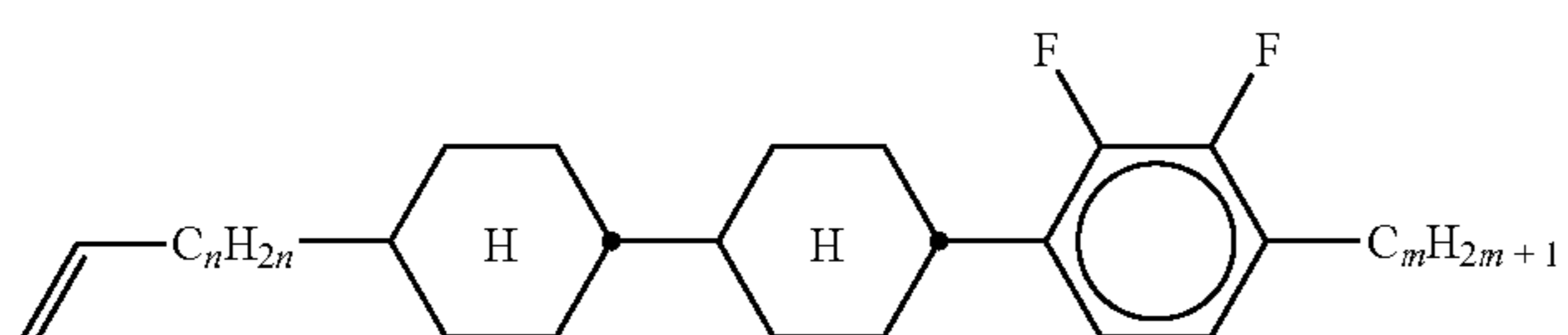
CCY-Vn-m
