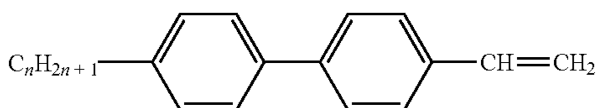
PP-n-V
