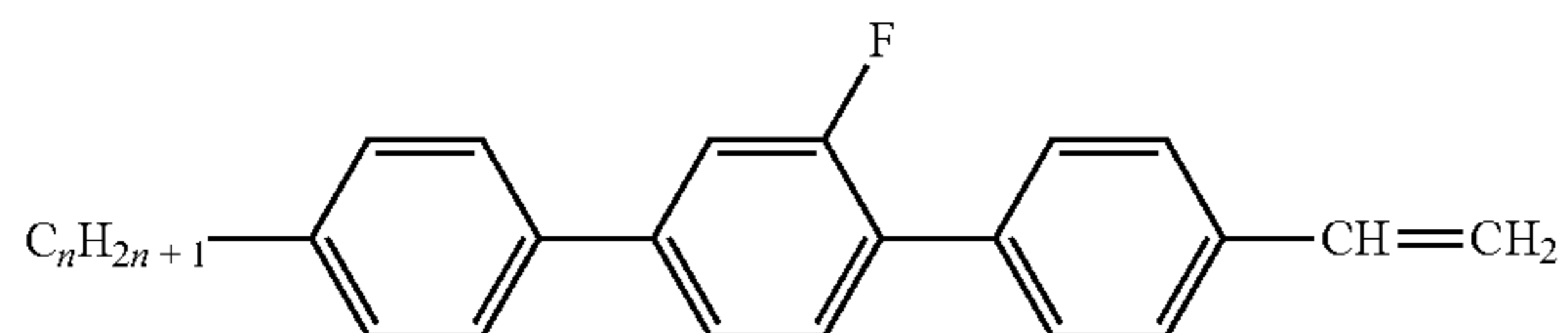
PGP-n-V
