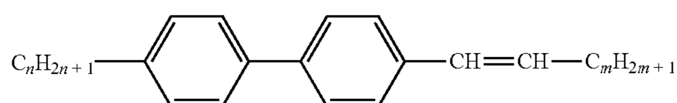
PP-n-Vm
