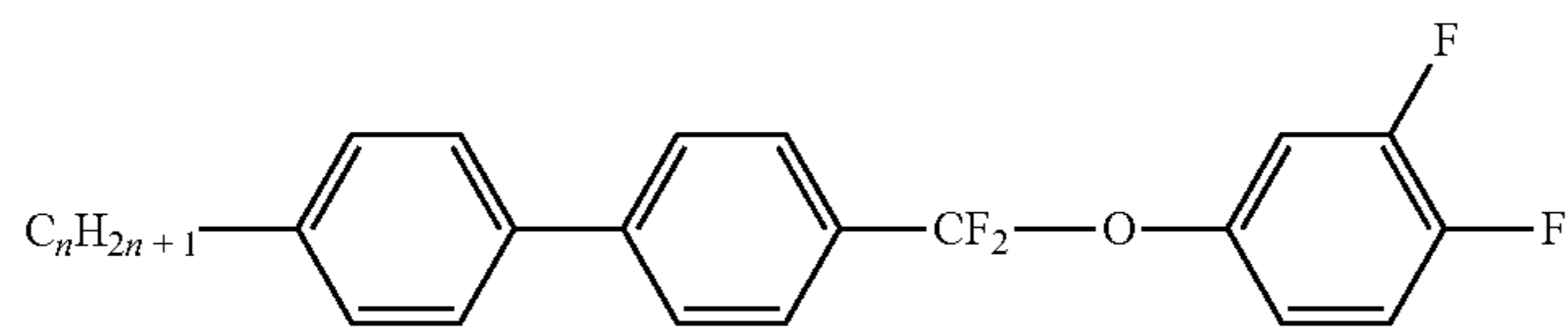
PPQG-n-F
