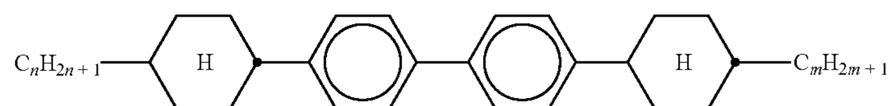
CBC-nm
