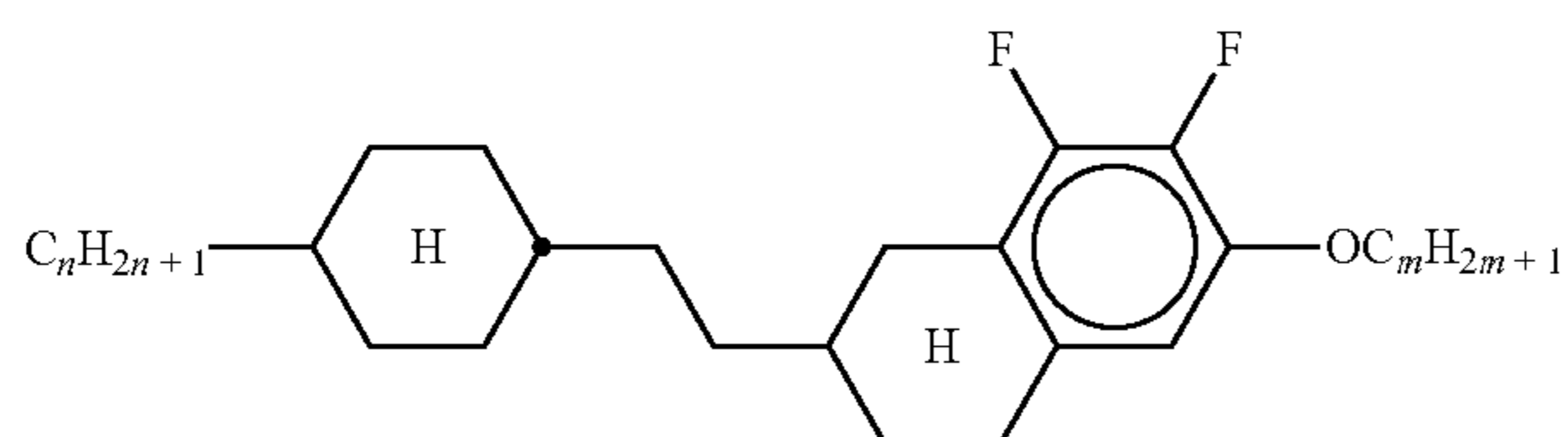
CETNap-n-Om
