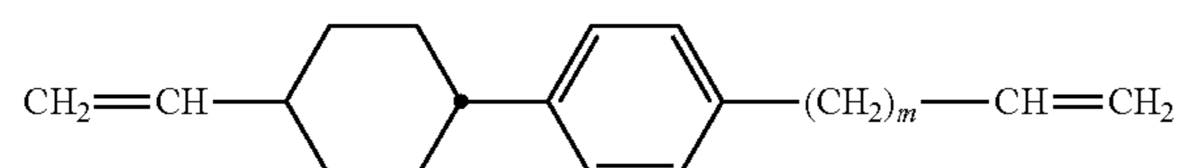
CP-V-mV
