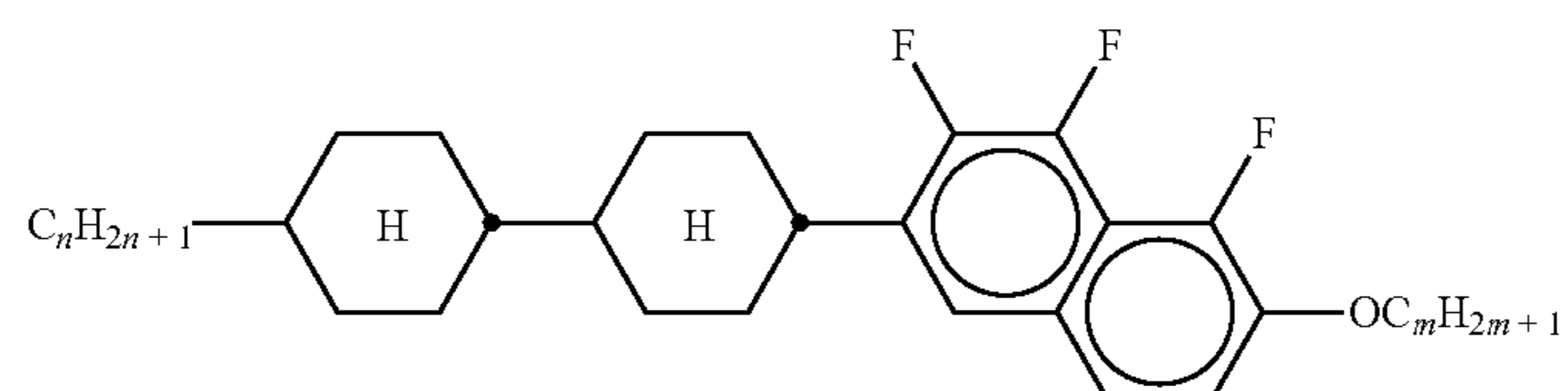
CCNap-n-Om
