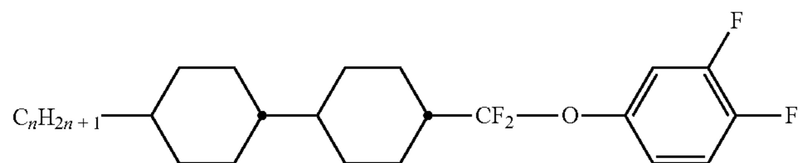
CCQG-n-F
