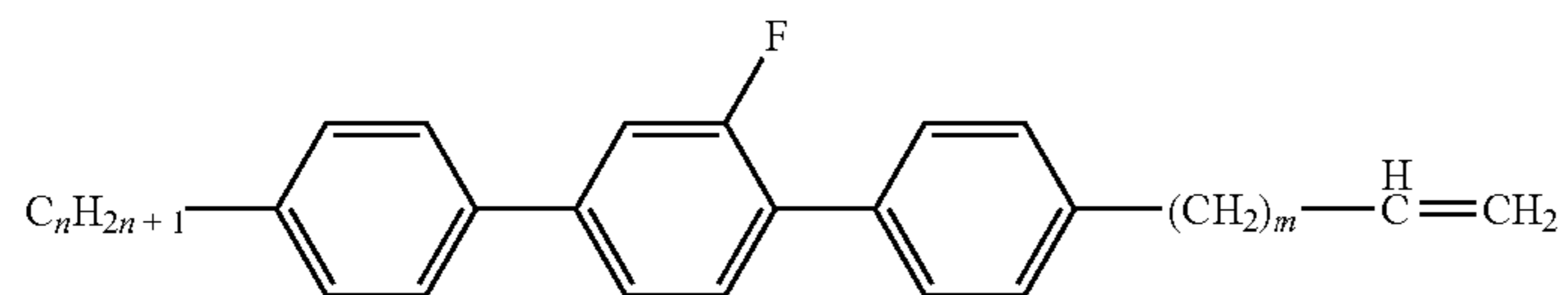
PGP-n-mV
