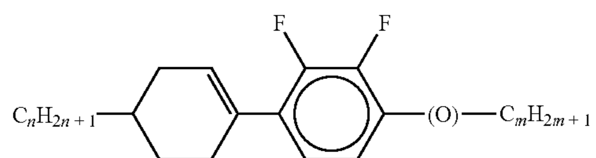
LY-n-(O)m
