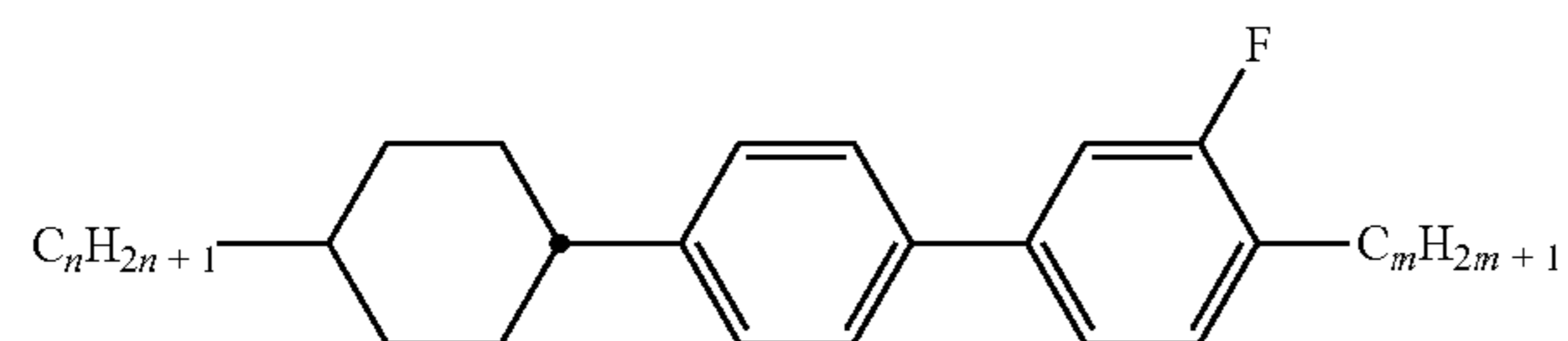
CPG-n-m
