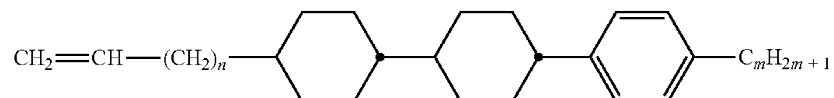
CCP-Vn-m
