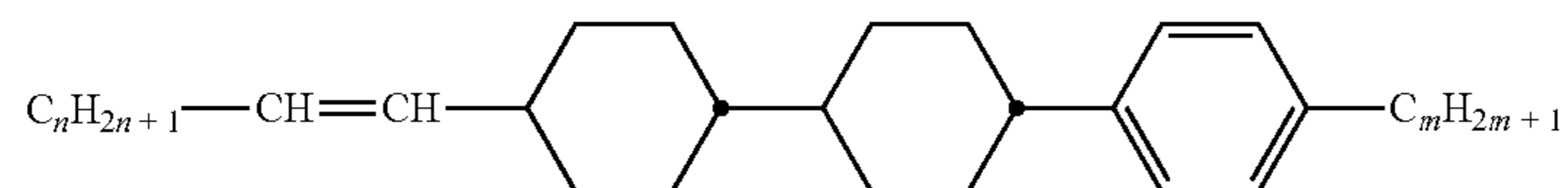
CCP-nV-m
