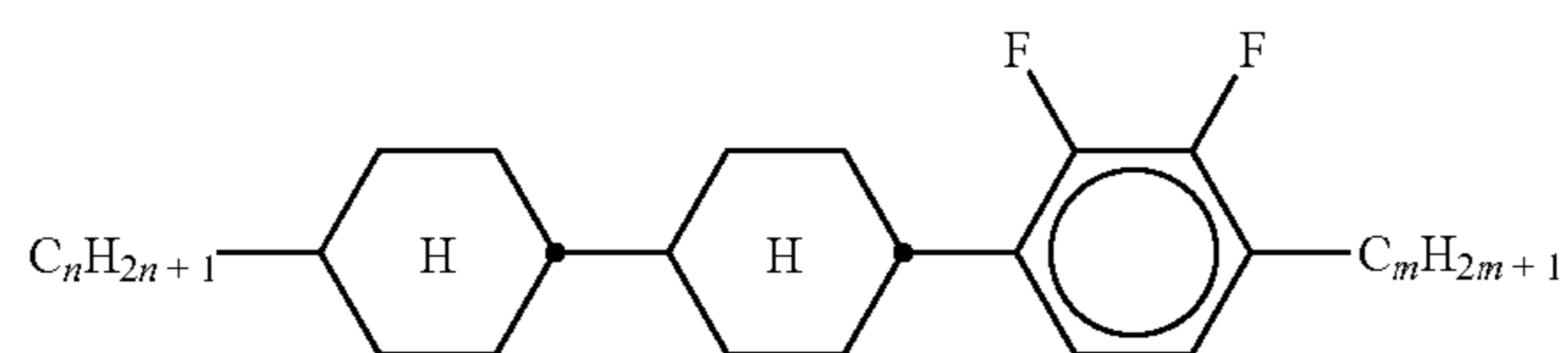
CCY-n-m
