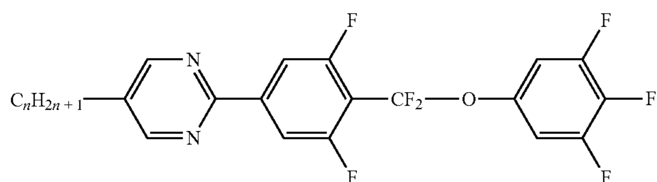
MUQU-n-F
