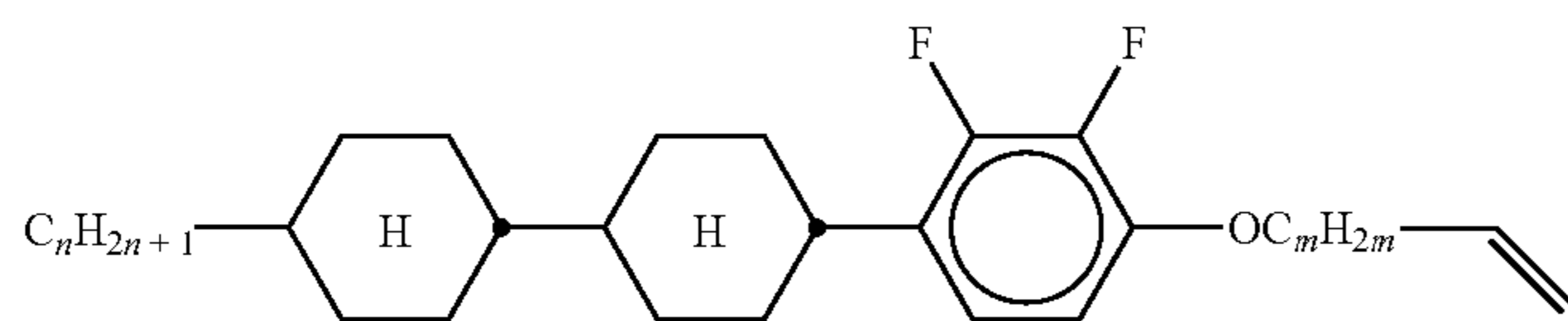
CCY-n-OmV
