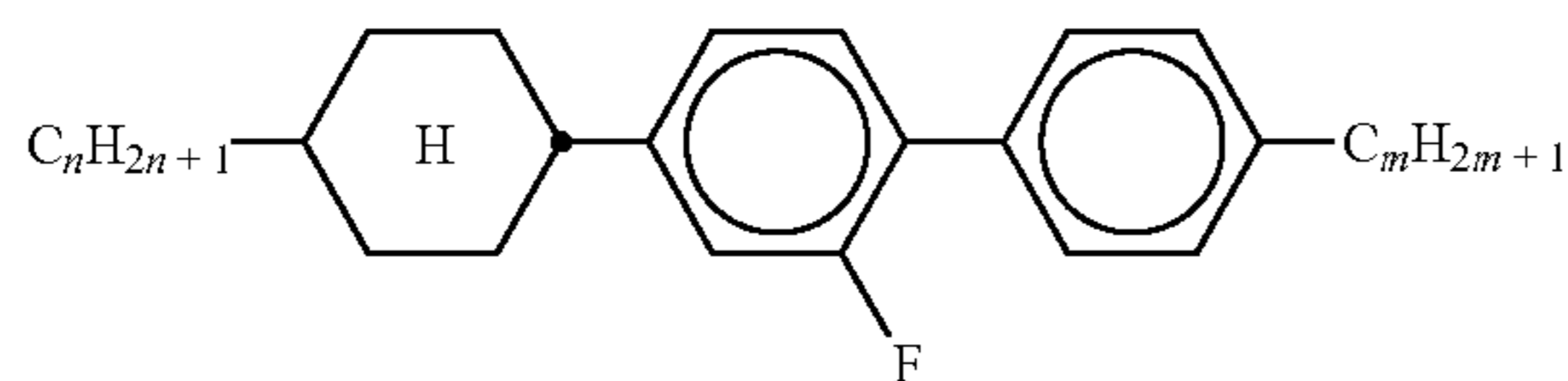
BCH-nmF
