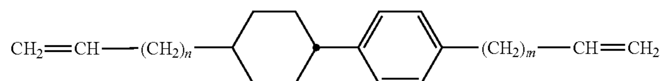
CP-Vn-mV
