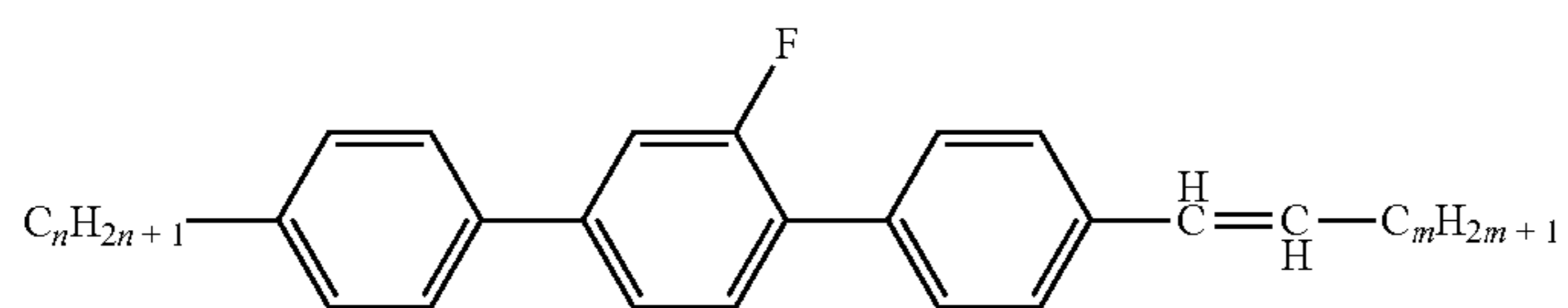
PGP-n-Vm
