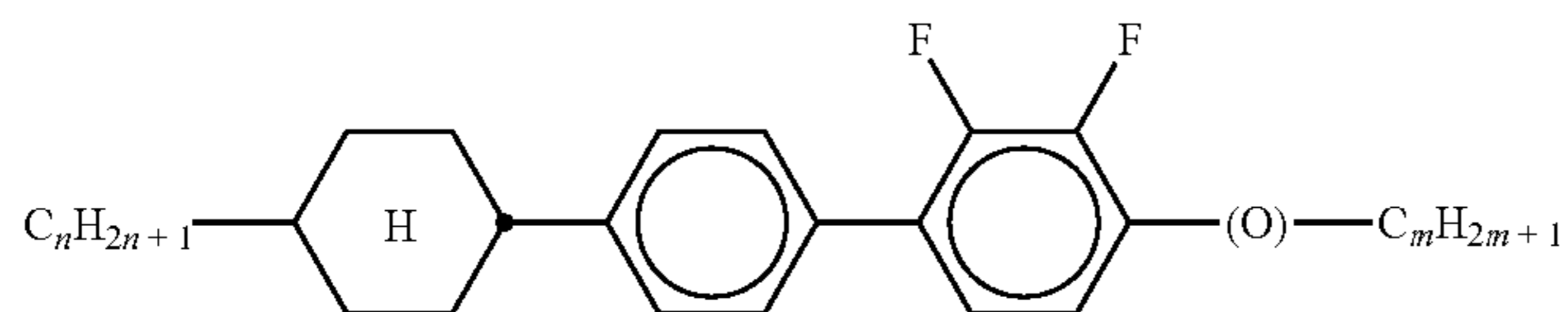
CPY-n-(O)m
