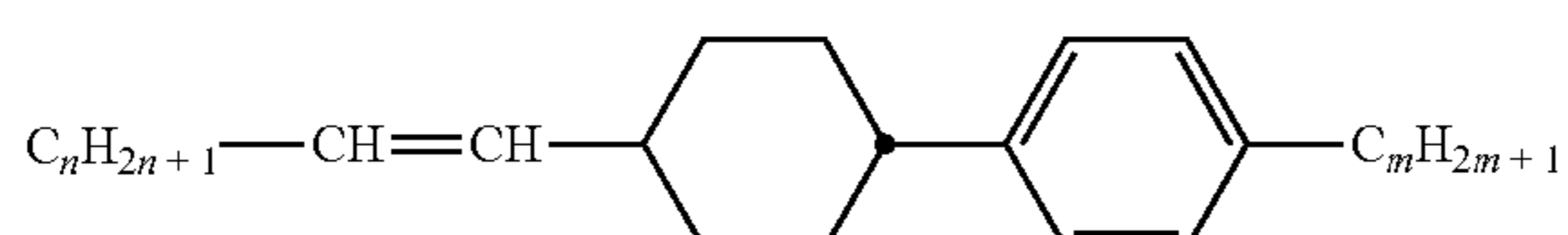
CP-nV-m
