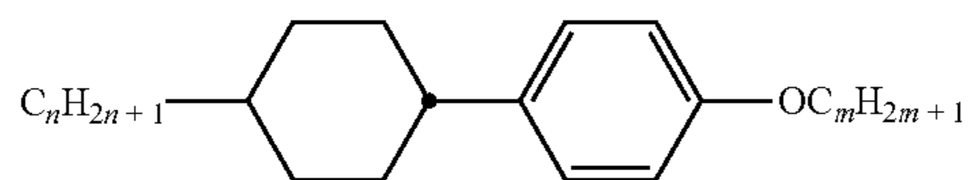
CP-n-Om
