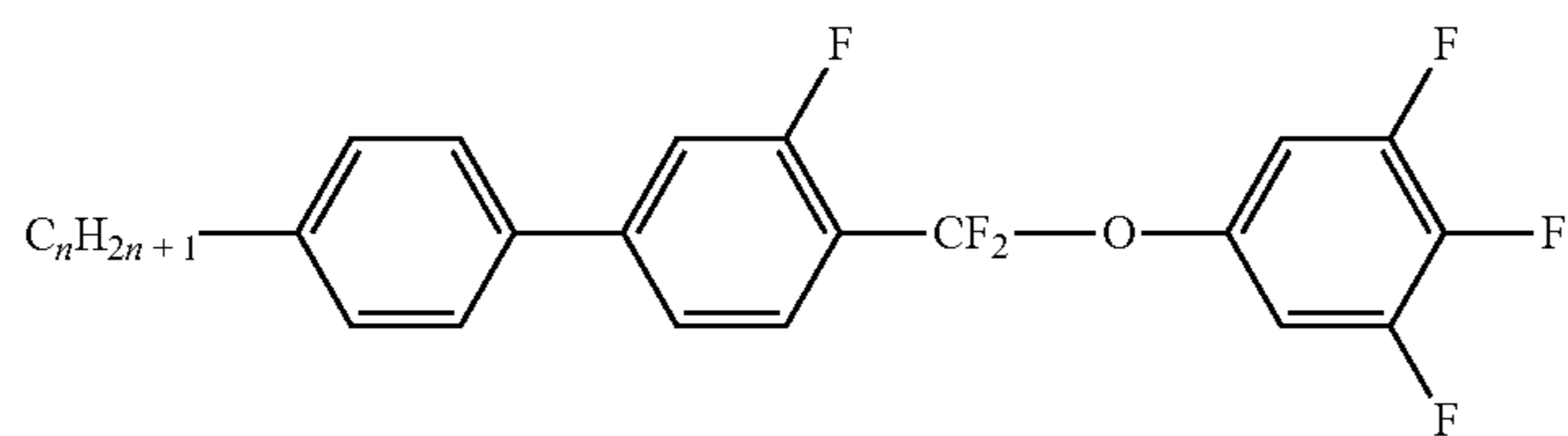
PGQU-n-F
