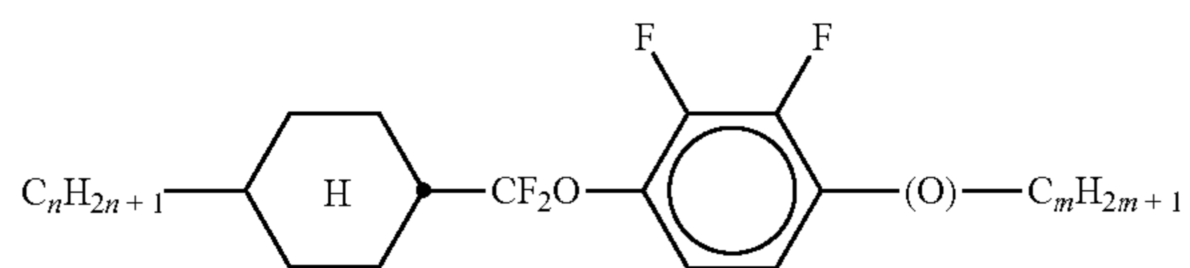
CQY-n-(O)m
