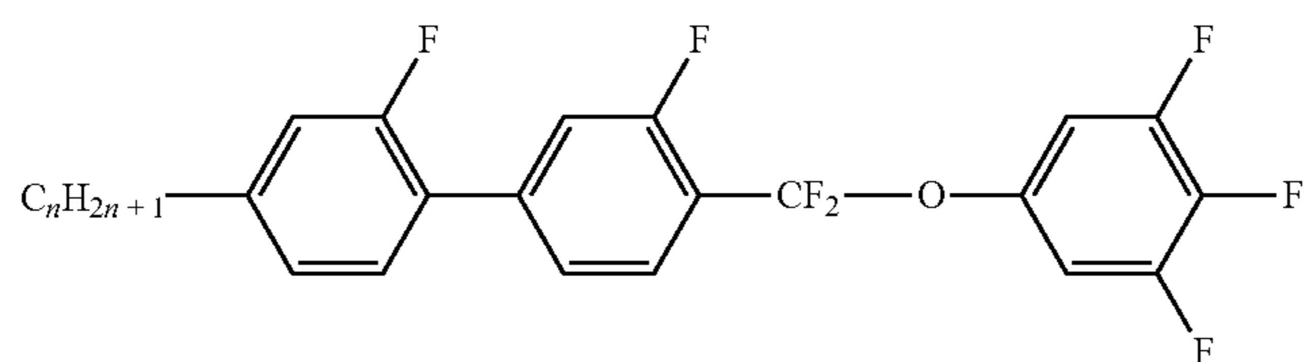
GGQU-n-F
