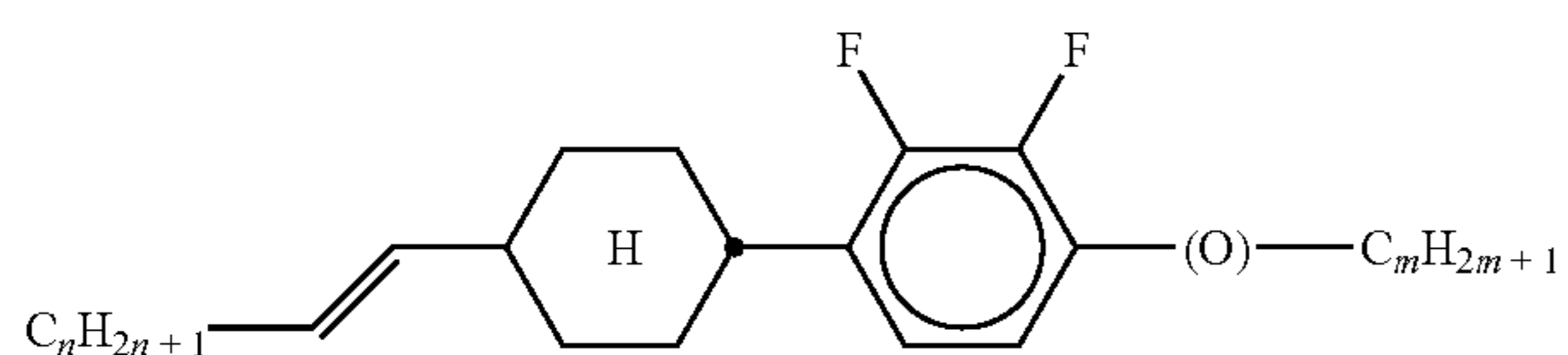
CY-nV-(O)m
