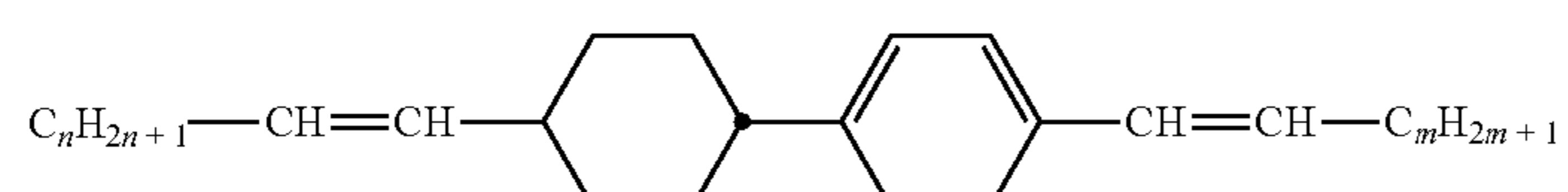
CP-nV-Vm
