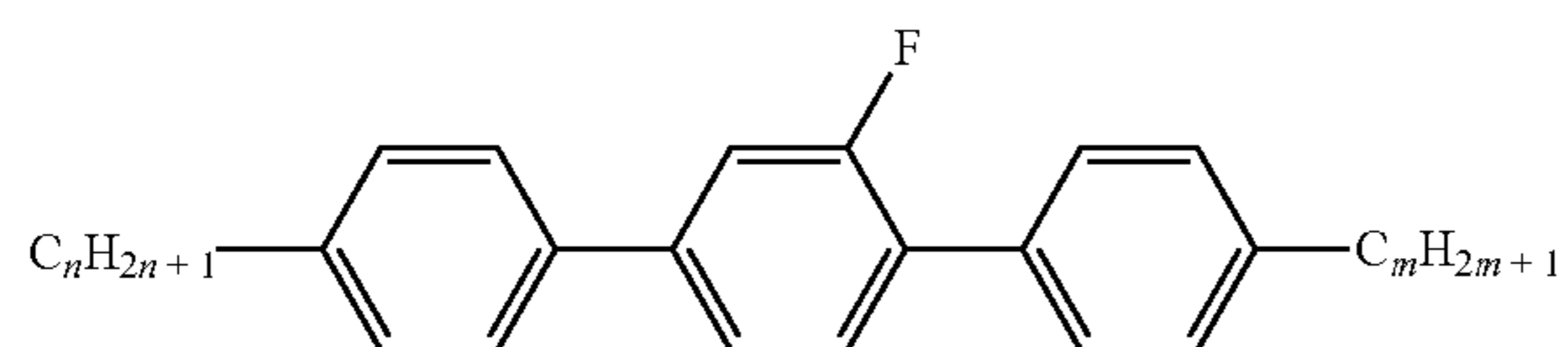
PGP-n-m
