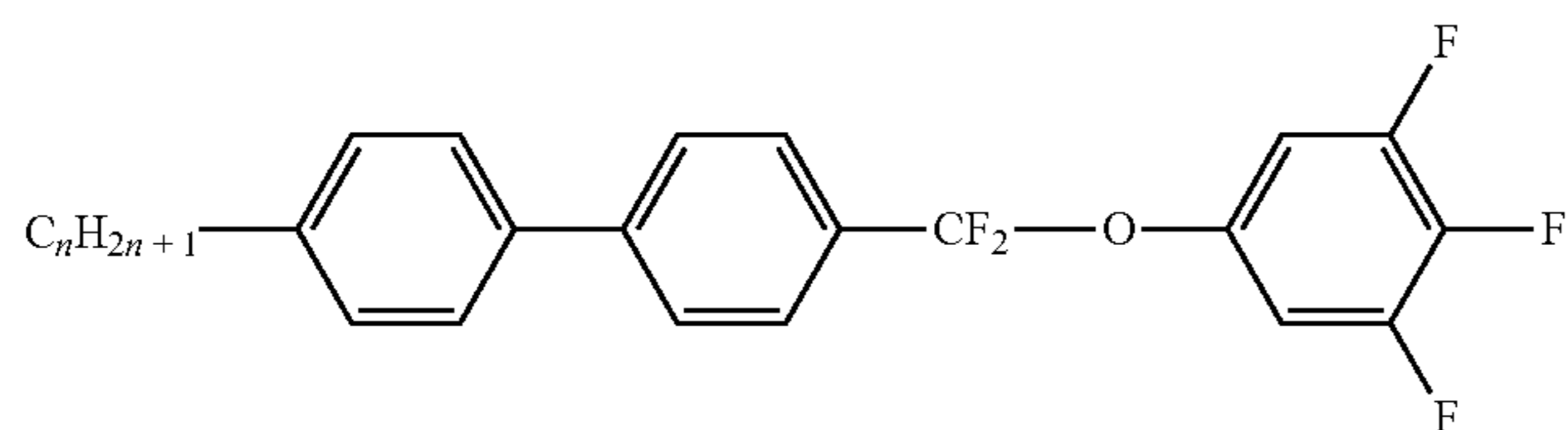
PPQU-n-F
