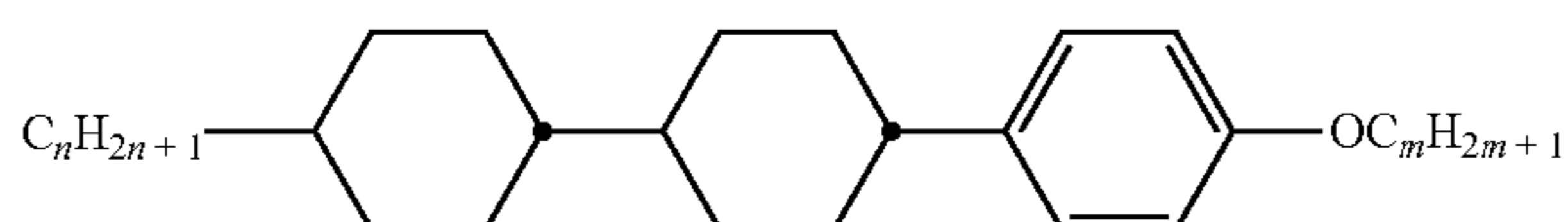
CCP-n-Om
