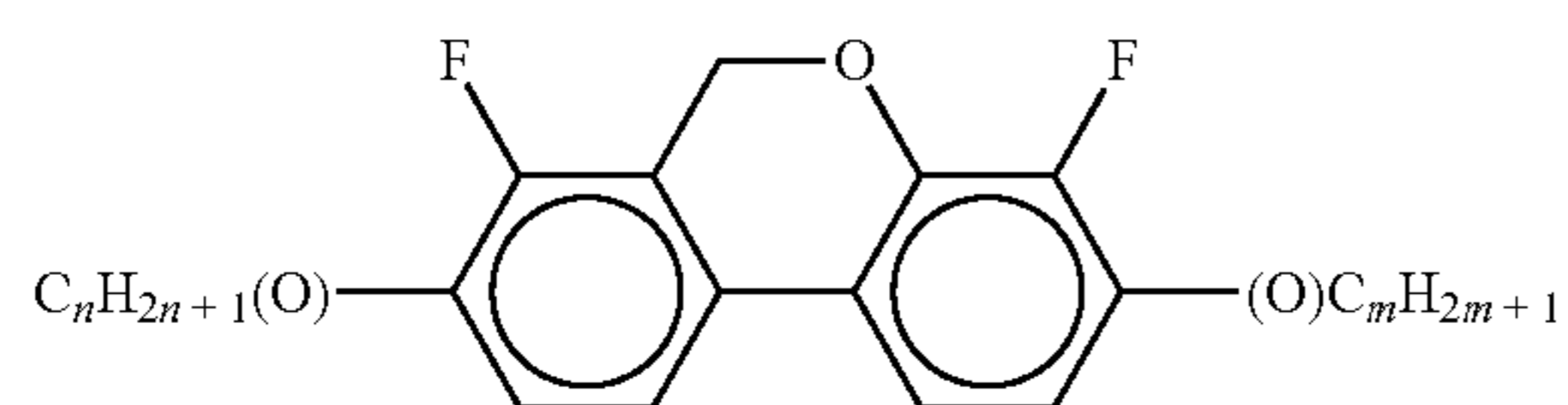
DFDBC-n(O)-(O)m
