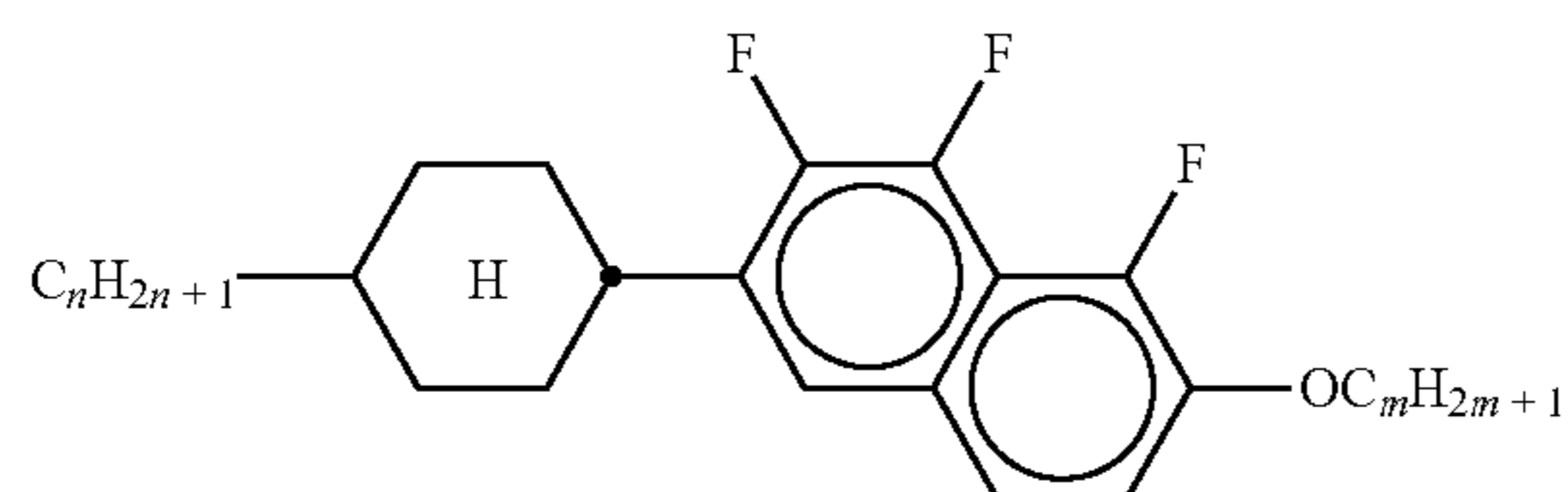
CNap-n-Om
