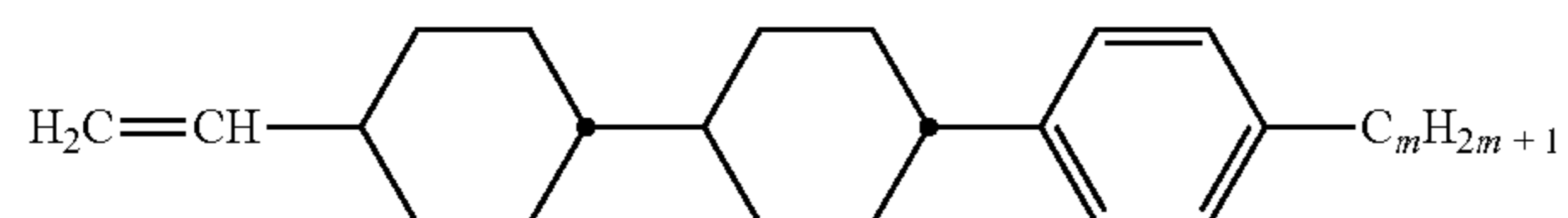
CCP-V-m
