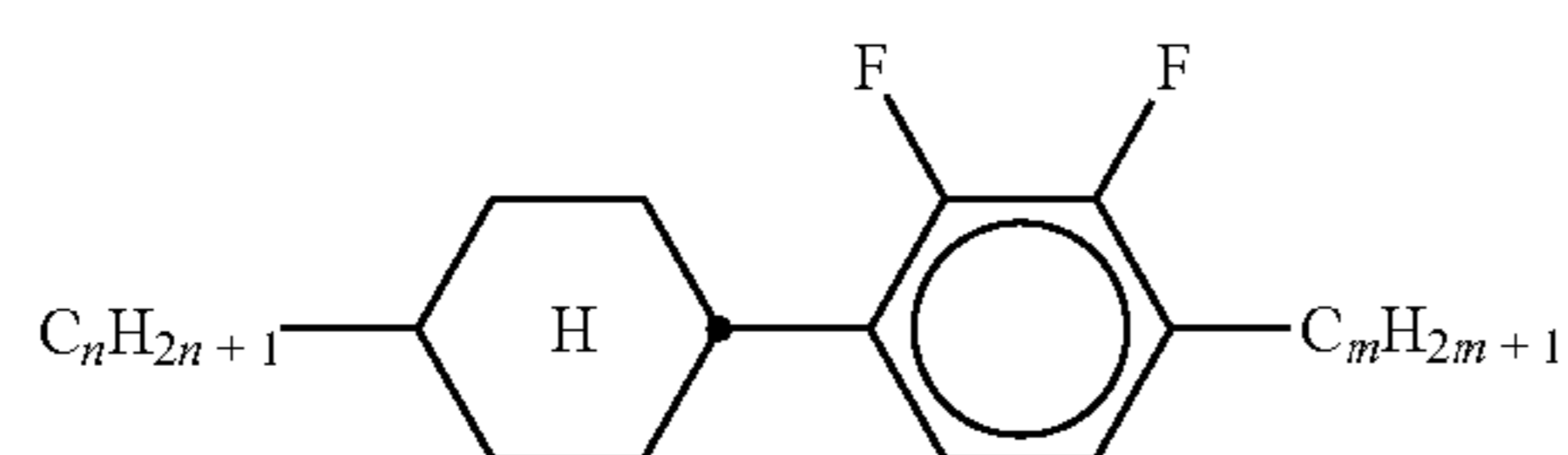
CY-n-m
