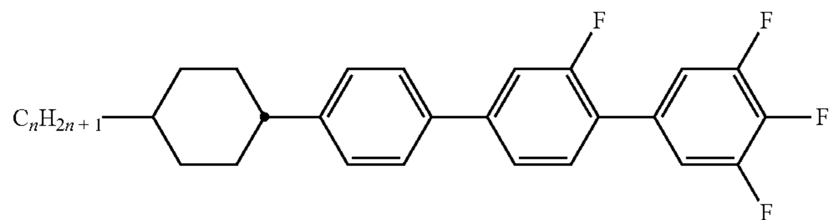
CPGU-n-F
