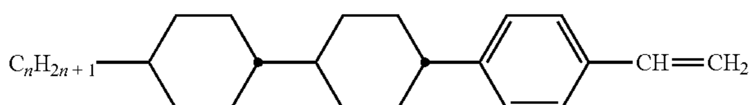
CCP-n-V
