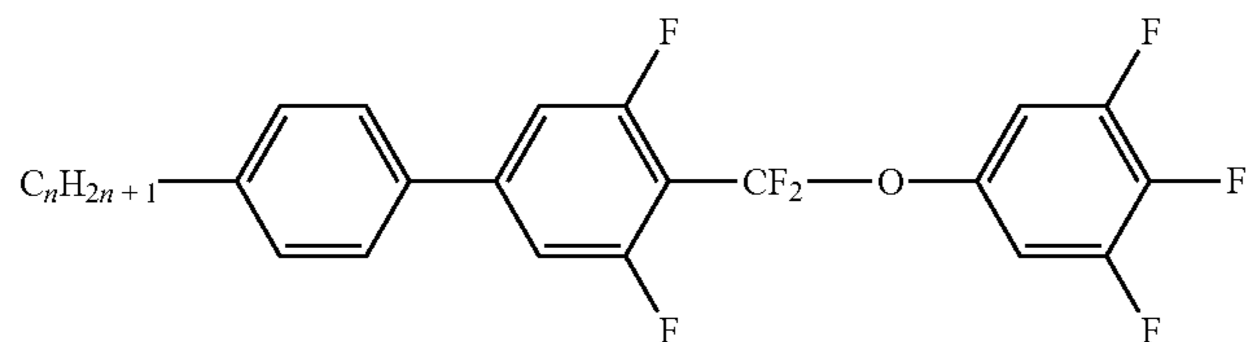
PUQU-n-F
