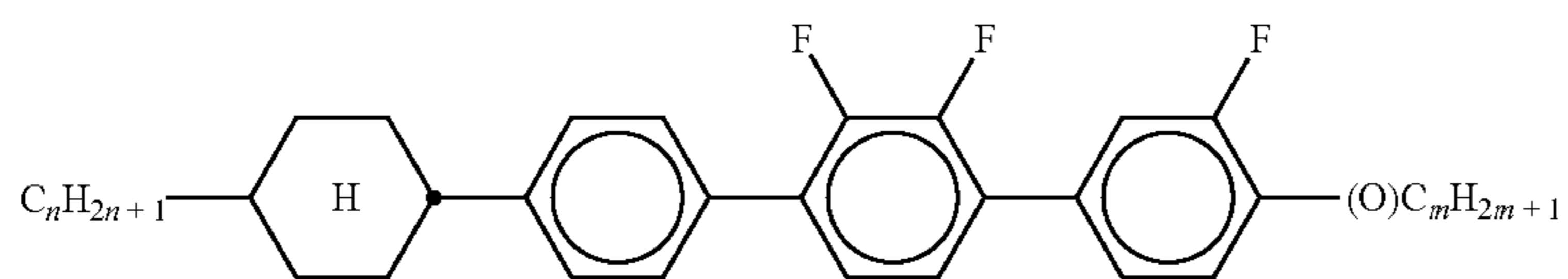
CPYP-n-(O)m
