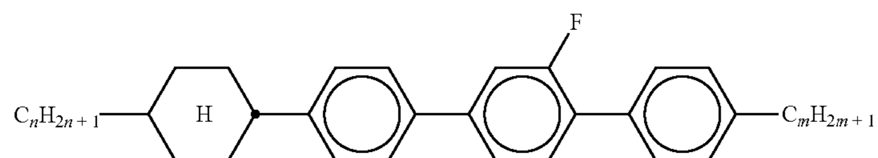
CPGP-n-m
