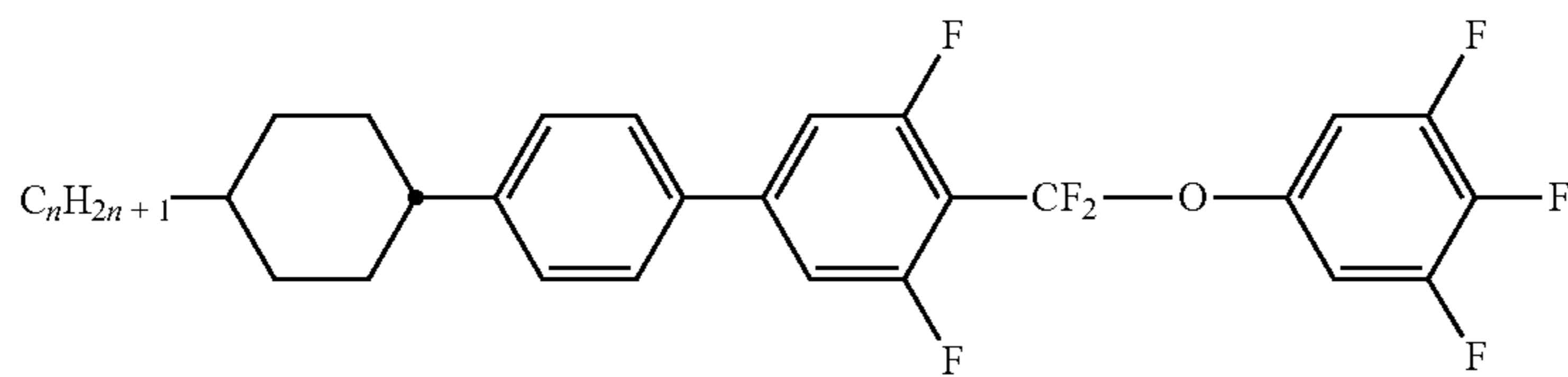
CPUQU-n-F
