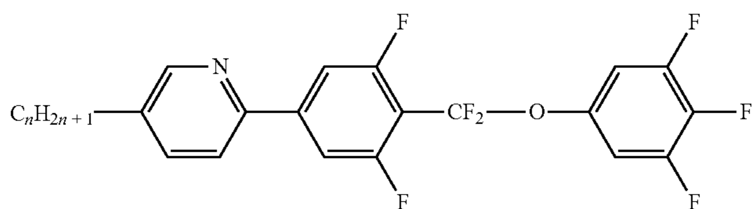
NUQU-n-F
