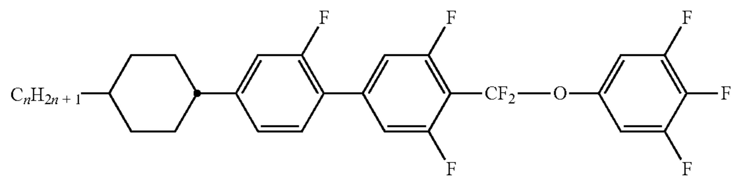
CGUQU-n-F
