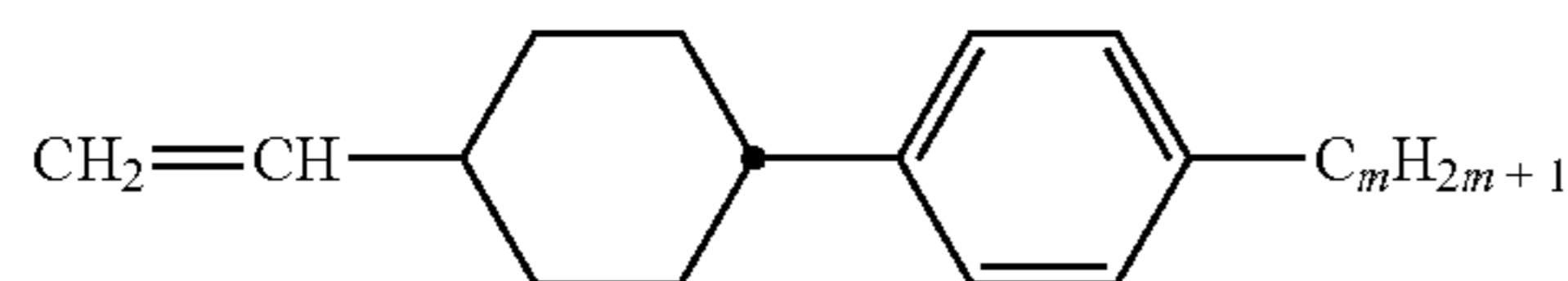
CP-V-m
