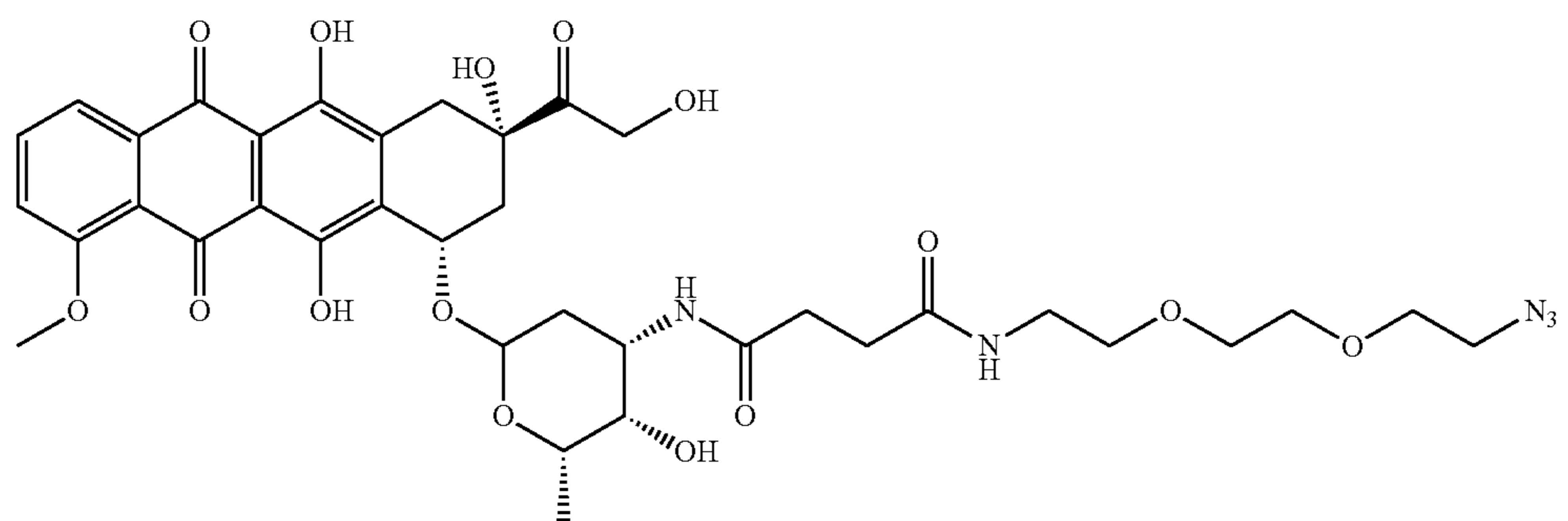
9-4 doxorubicin-PEG-azide
