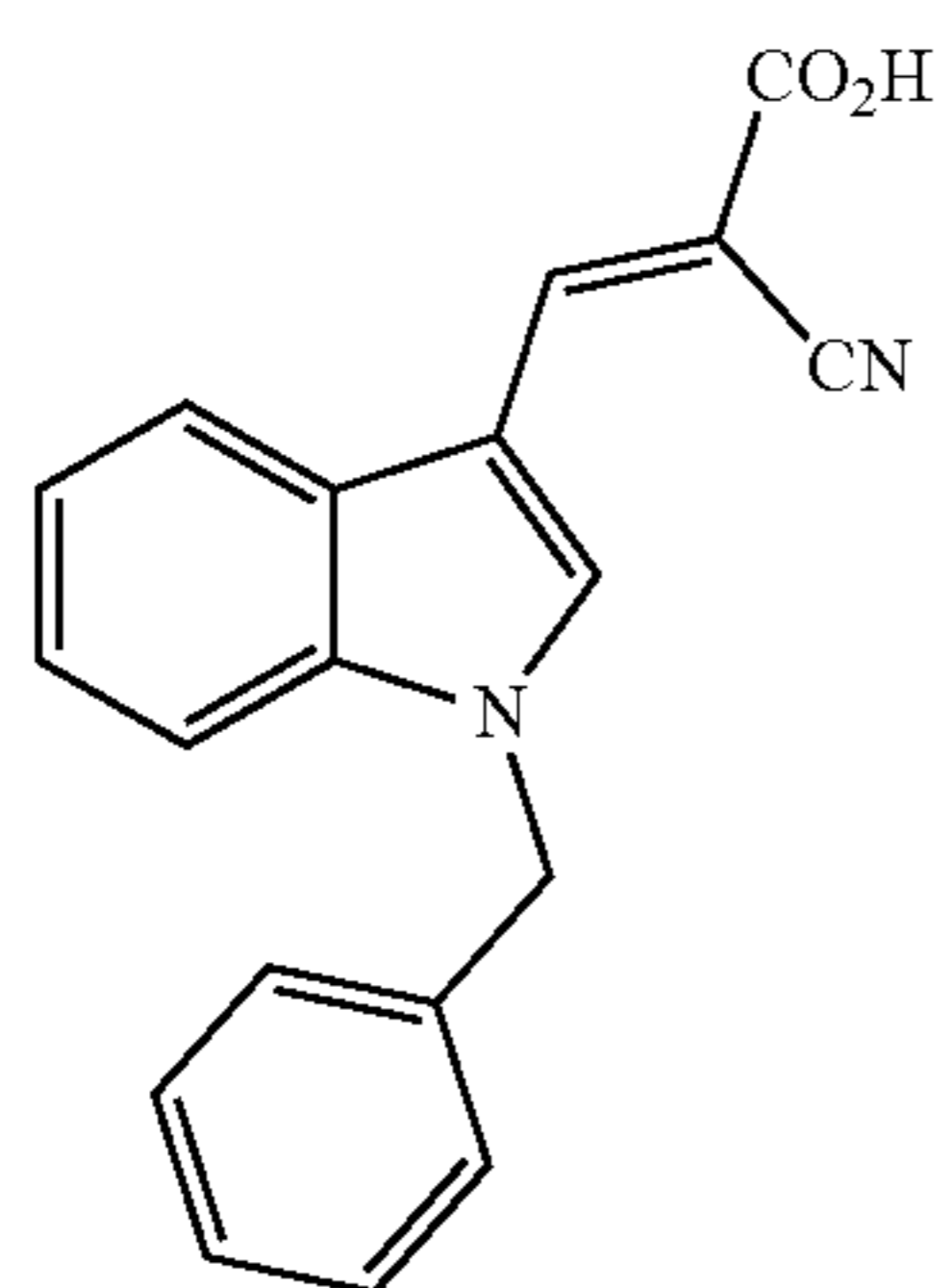
(E)-3-(1-Benzyl-1H-indol-3-yl)-2-cyanoacrylic Acid (JXL019)
