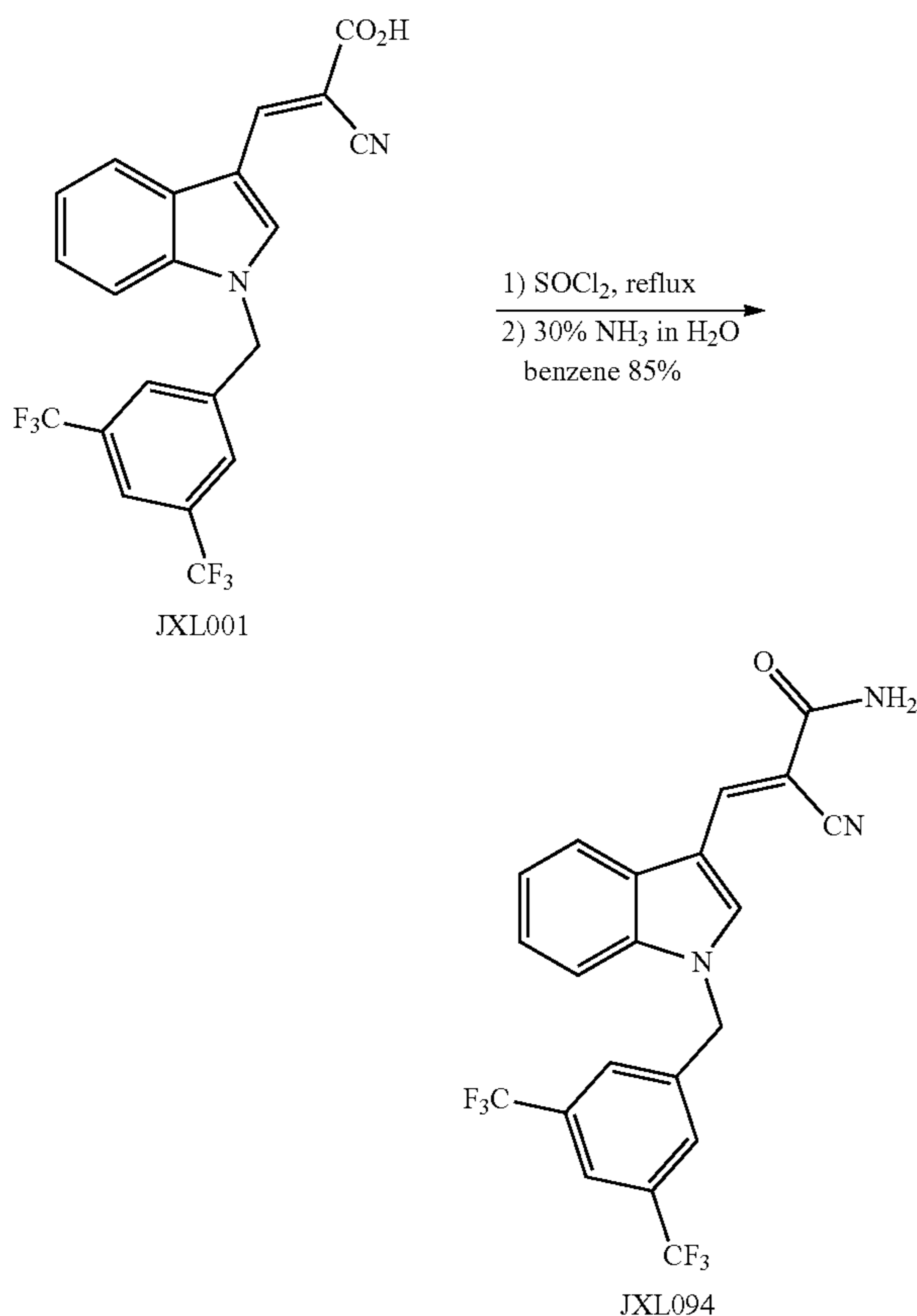
(E)-3-(1-(3,5-Bis(trifluoromethyl)benzyl)-1H-indol-3-yl)-2-cyanoacrylamide (JXL094)
