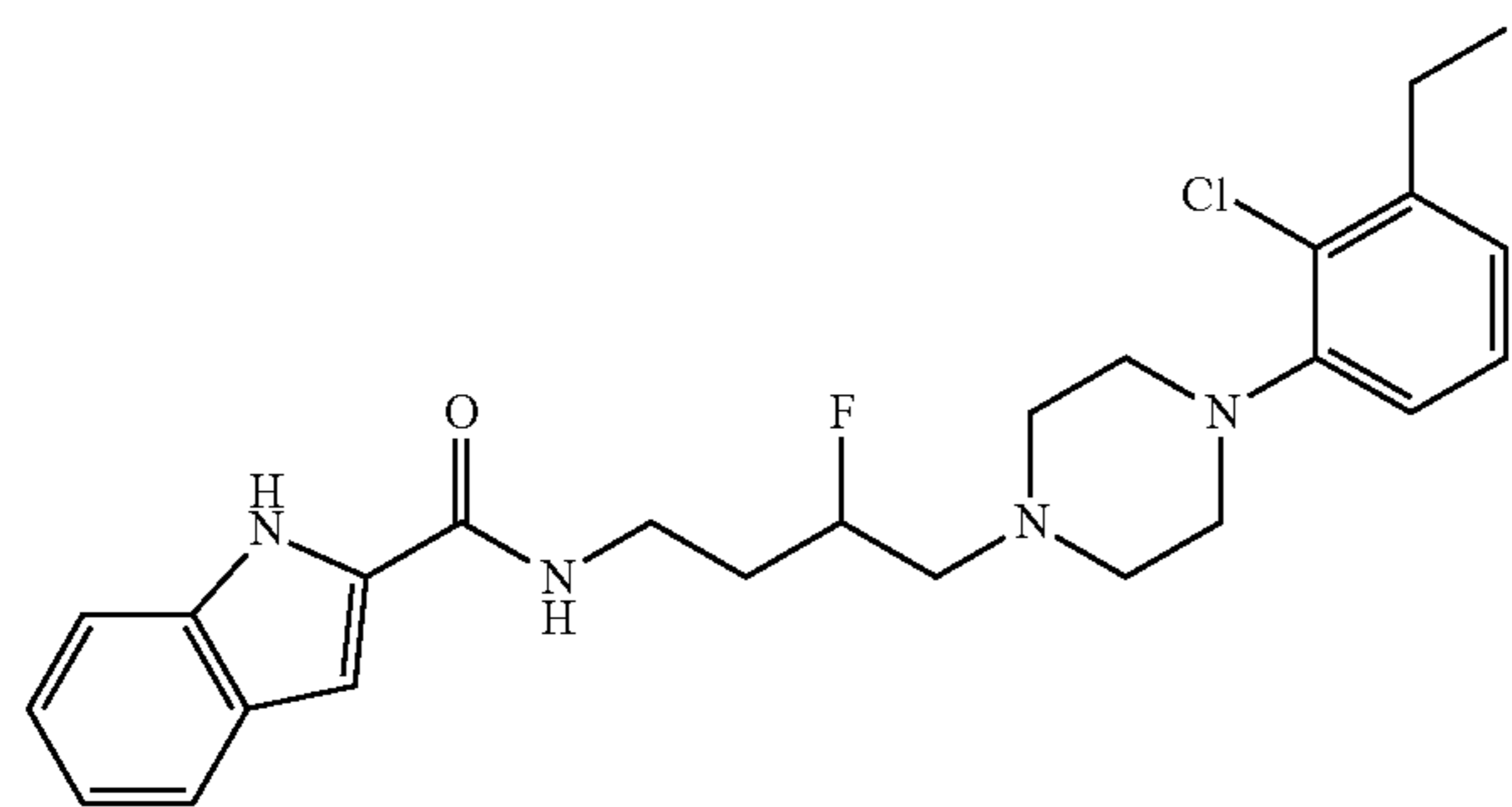
N-(4-(4-(2-chloro-3-ethylphenyl)piperazin-1-yl)-3-fluorobutyl)-1H-indole-2-carboxamide
