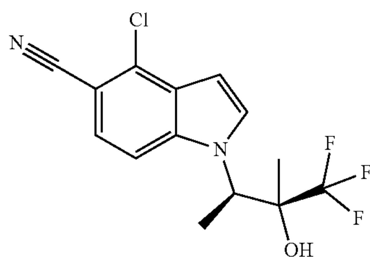
D. 4-Chloro-1-((2R,3S)-4,4,4-trifluoro-3-hydroxy-3-methylbutan-2-yl)-1H-indole-5-carbonitrile
