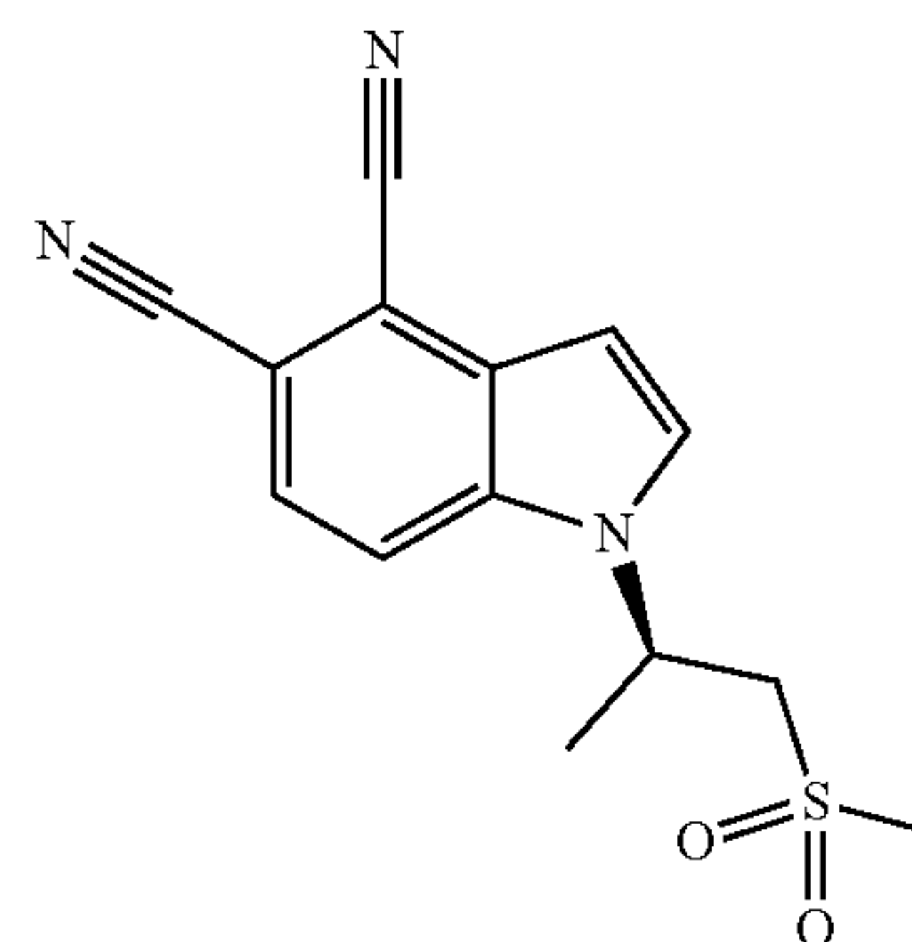
(R)-1-(1-(Methylsulfonyl)propan-2-yl)-1H-indole-4,5-dicarbonitrile
