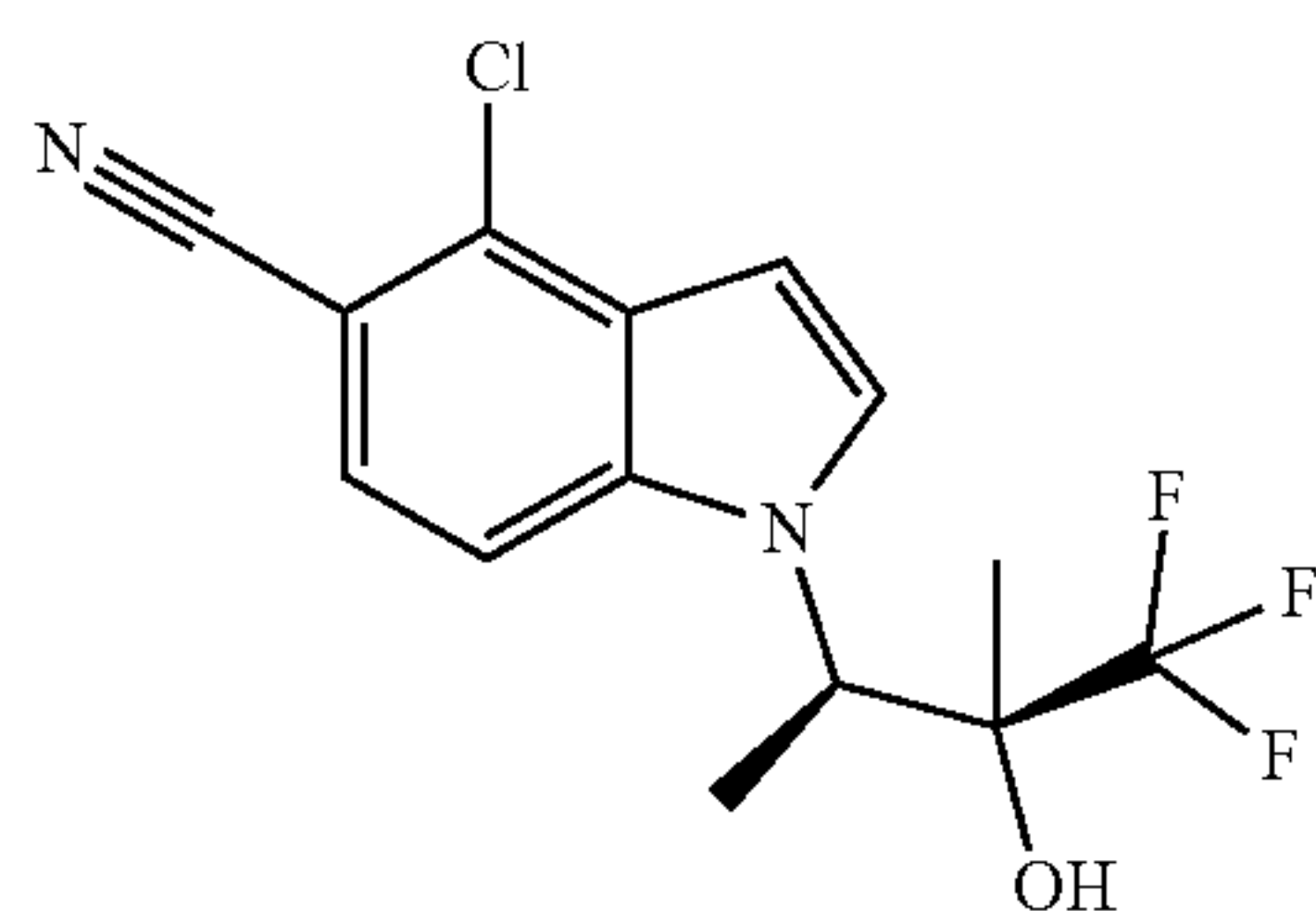
4-Chloro-1-((2R,3S)-4,4,4-trifluoro-3-hydroxy-3-methylbutan-2-yl)-1H-indole-5-carbonitrile
