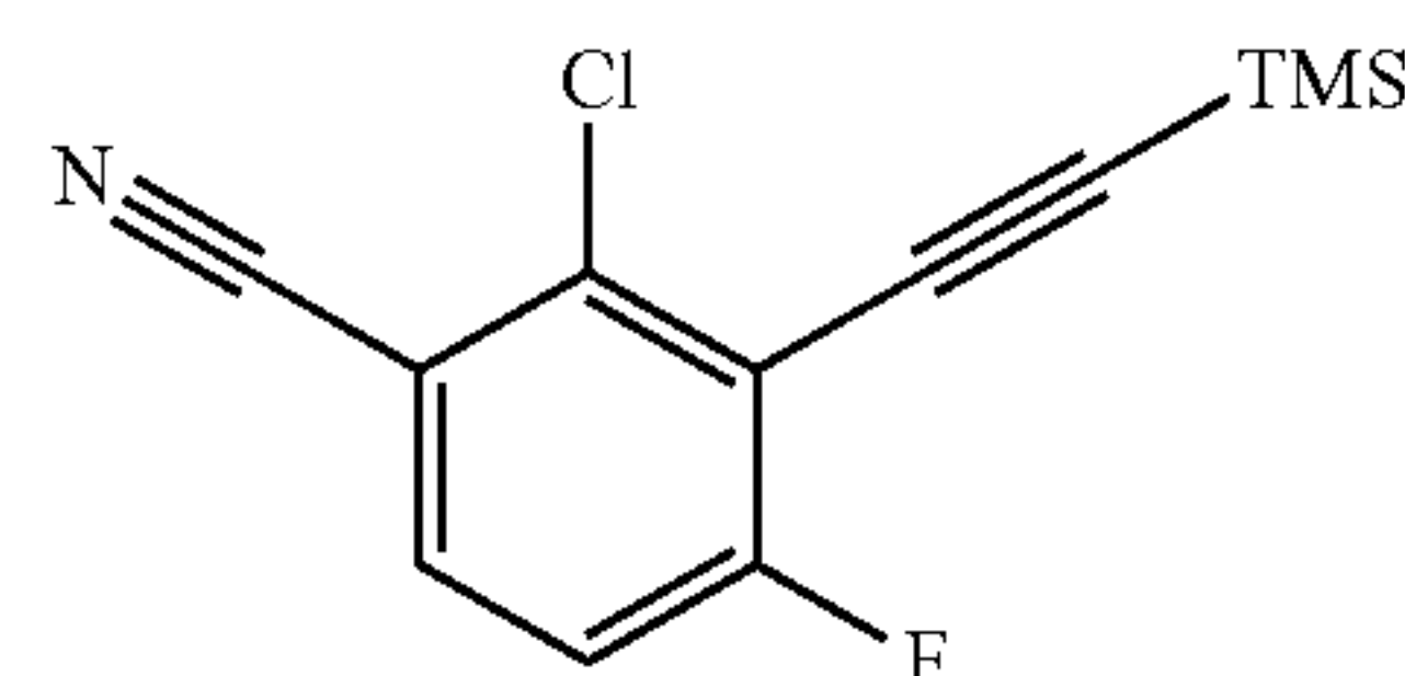
B. 2-Chloro-4-fluoro-3-((trimethylsilyl)ethynyl)benzonitrile
