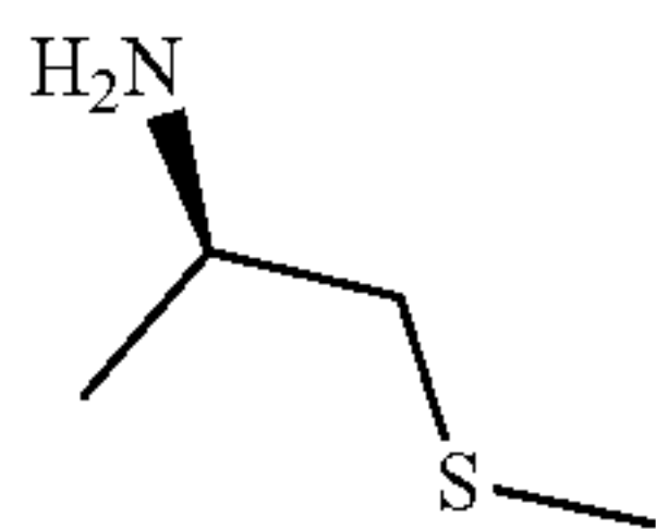
(R)-1-(Methylthio)propan-2-amine Hydrochloride
