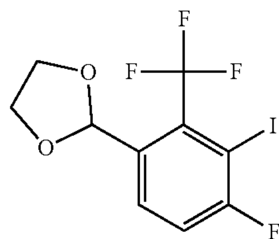
B. 2-(4-Fluoro-3-iodo-2-(trifluoromethyl)phenyl)-1,3-dioxolane
