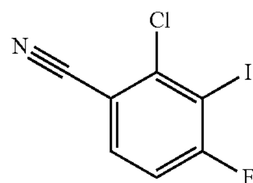
A. 2-Chloro-4-fluoro-3-iodobenzonitrile
