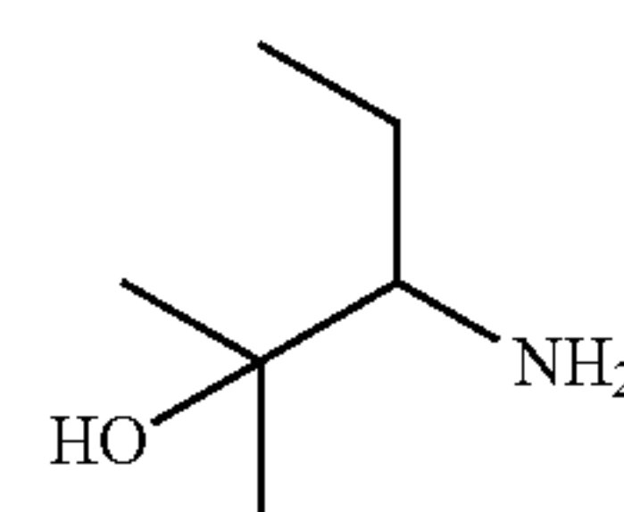
A. 3-Amino-2-methylpentan-2-ol
