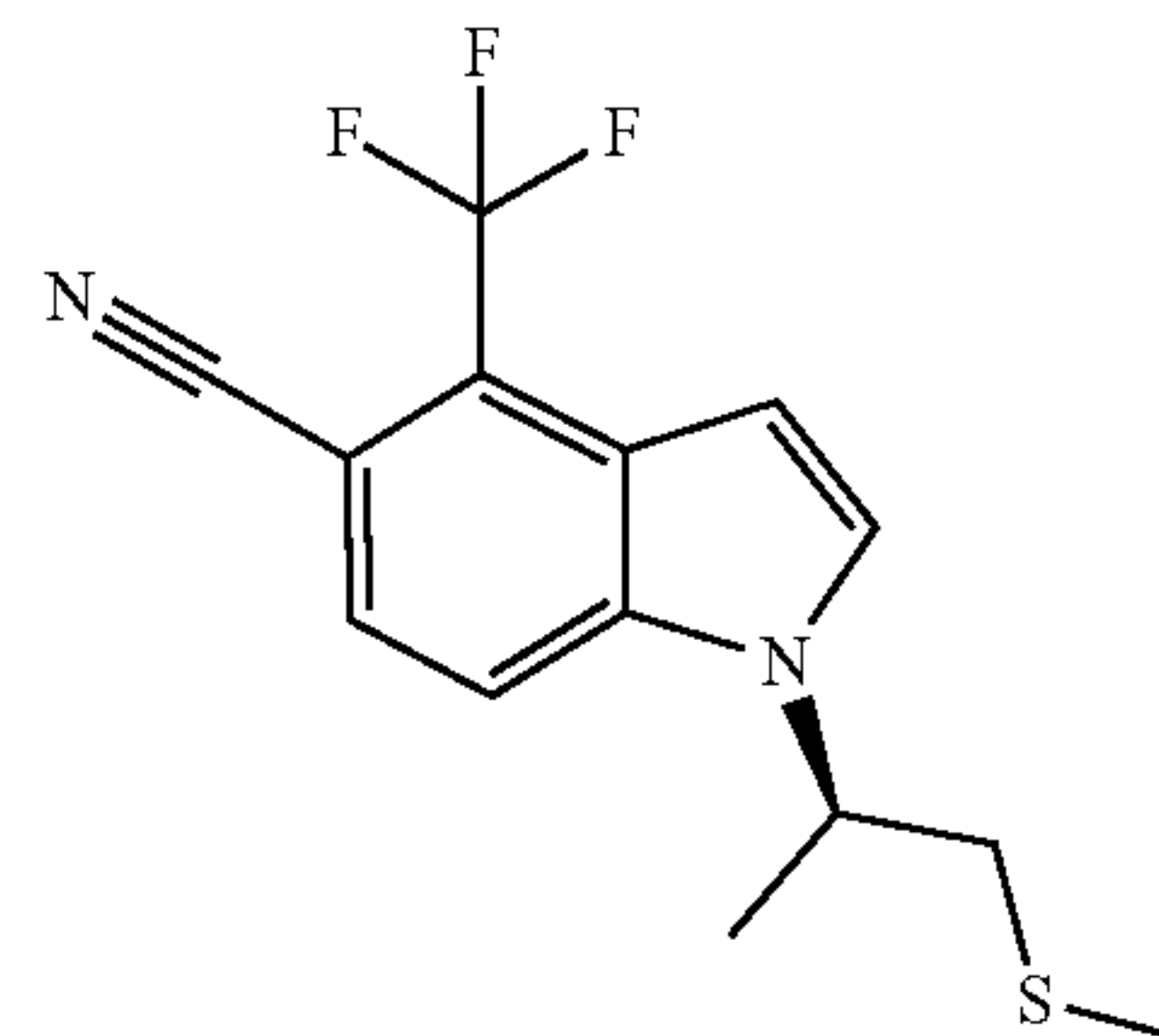
D. (R)-1-(1-(Methylthio)propan-2-yl)-4-(trifluoromethyl)-1H-indole-5-carbonitrile
