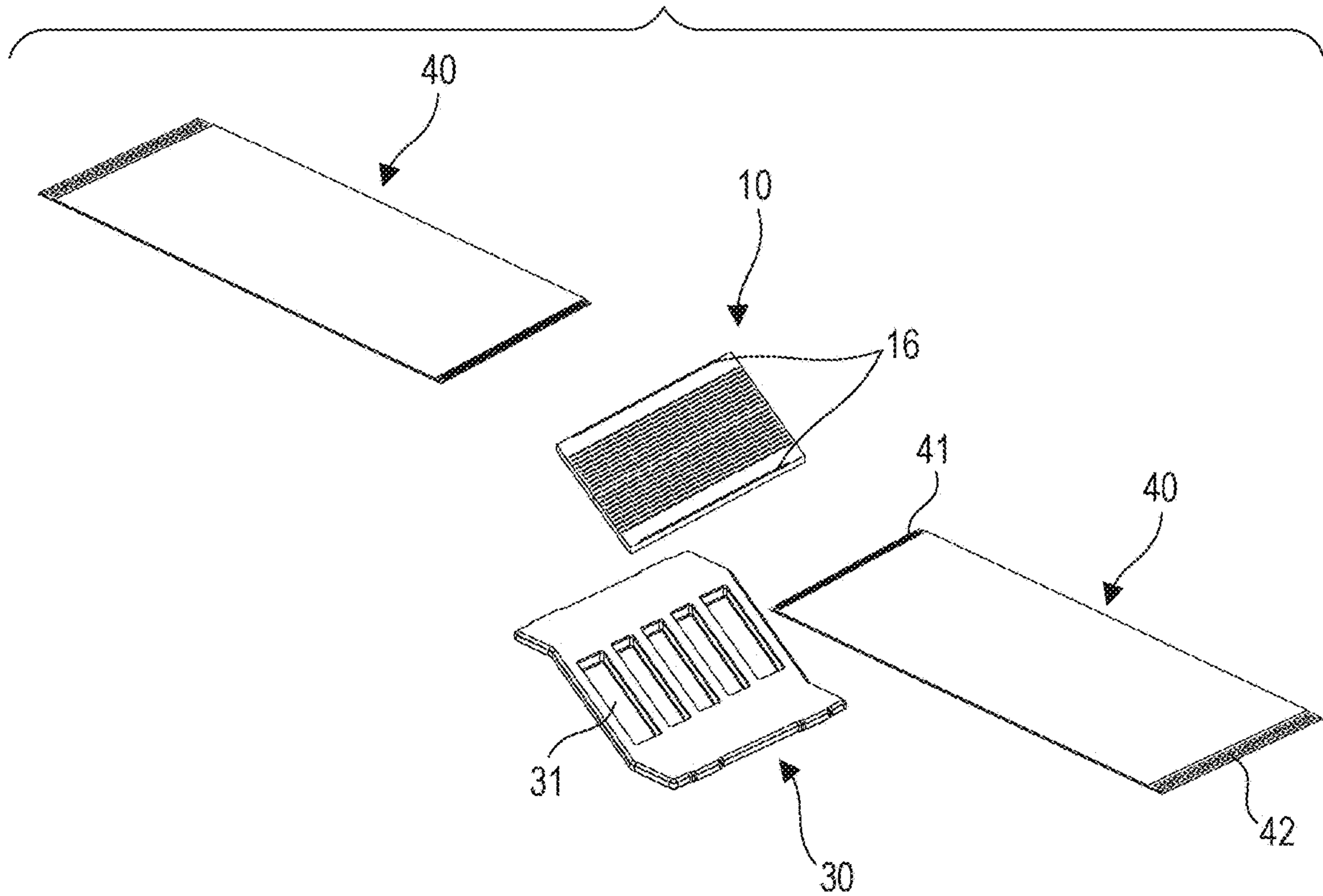
FIG. 19B
