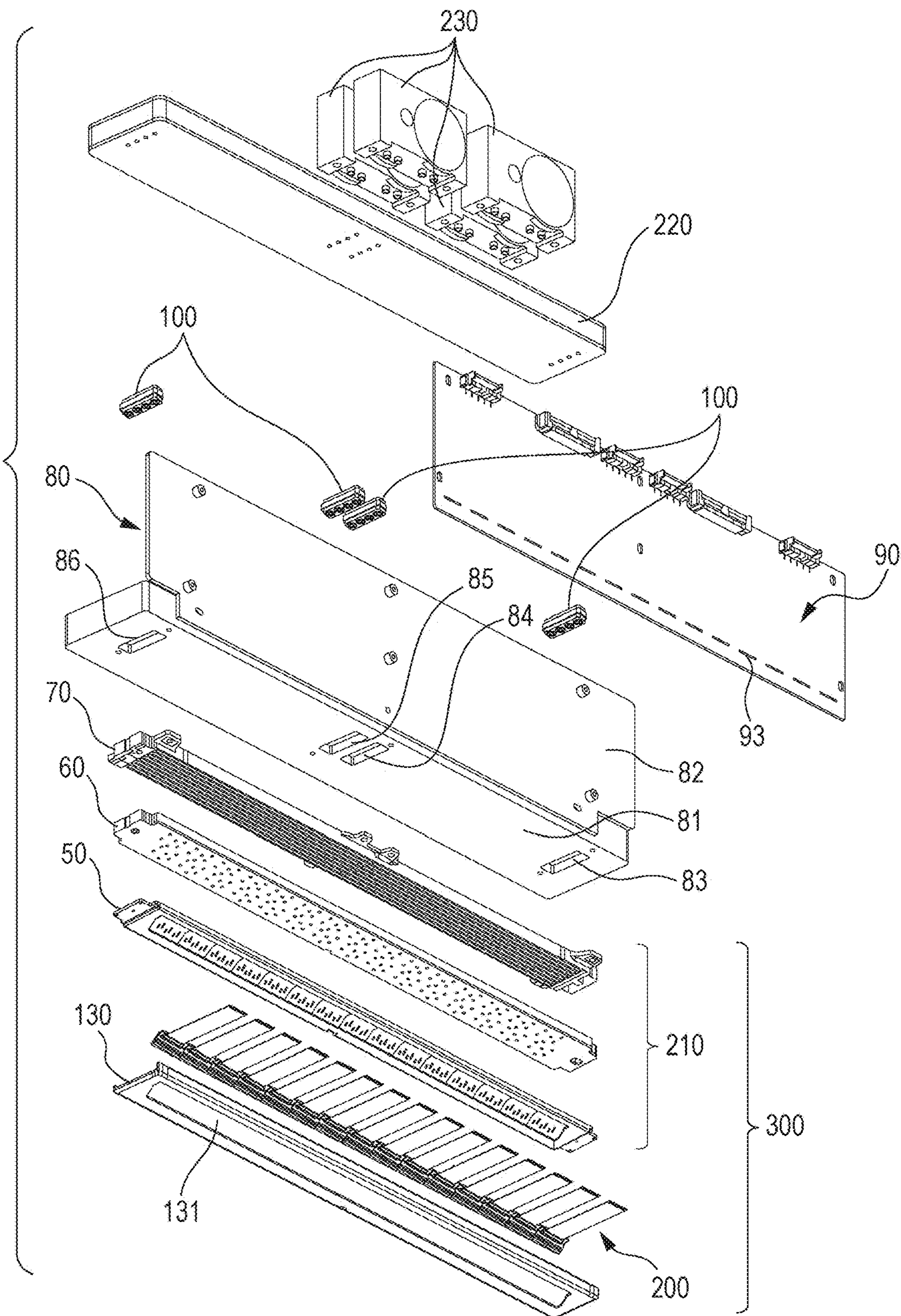
FIG. 30
