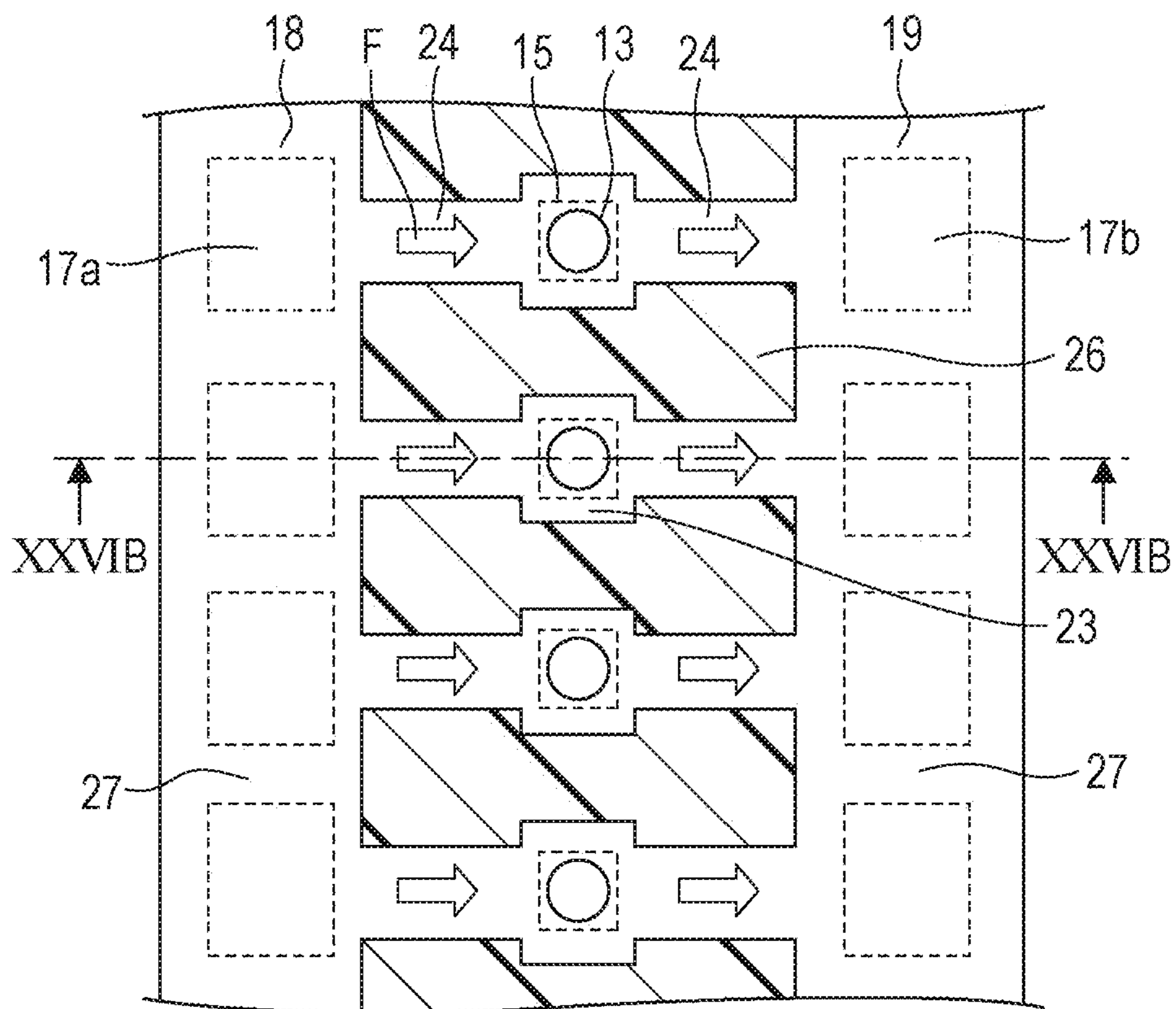
FIG. 26A
