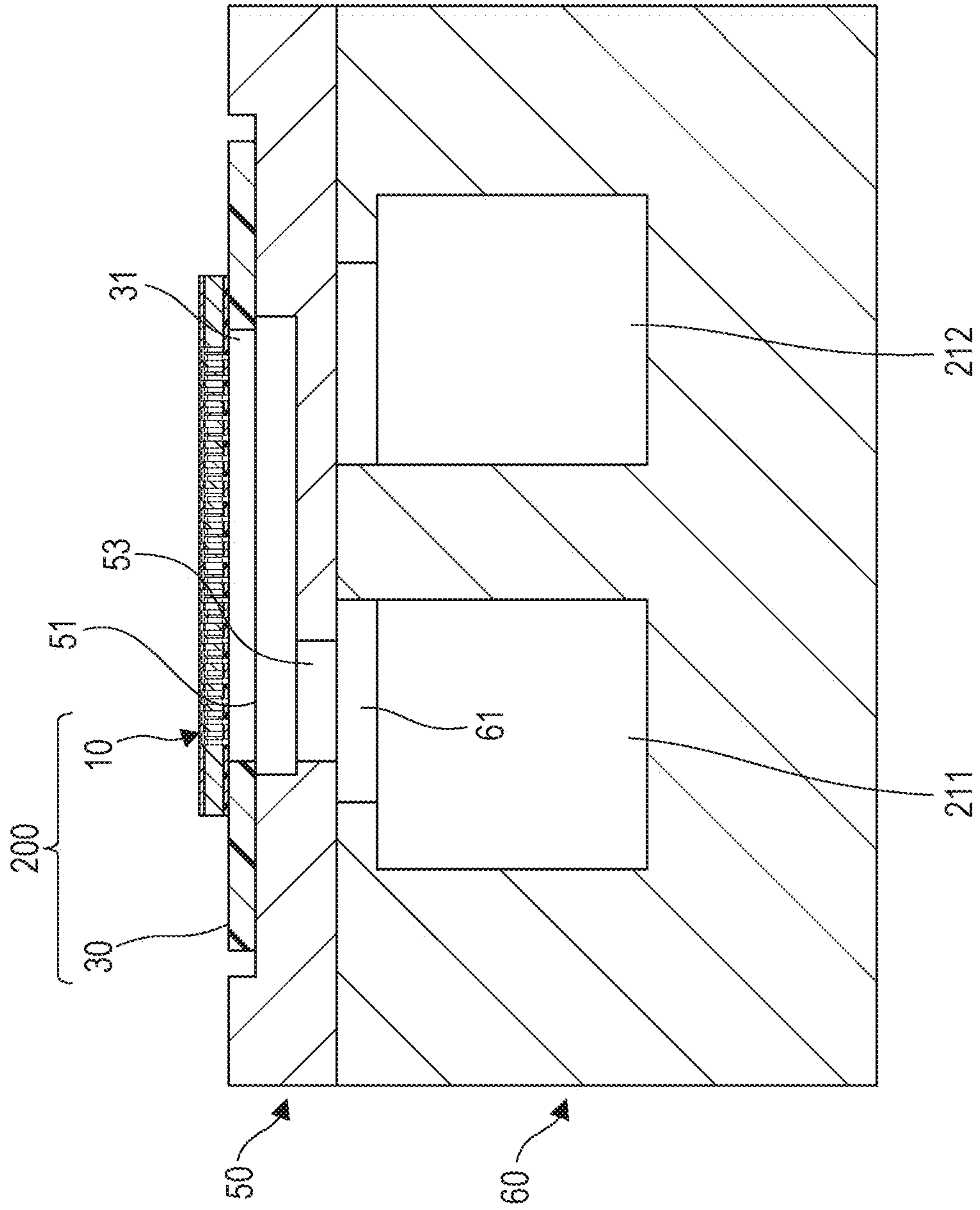
FIG. 18
