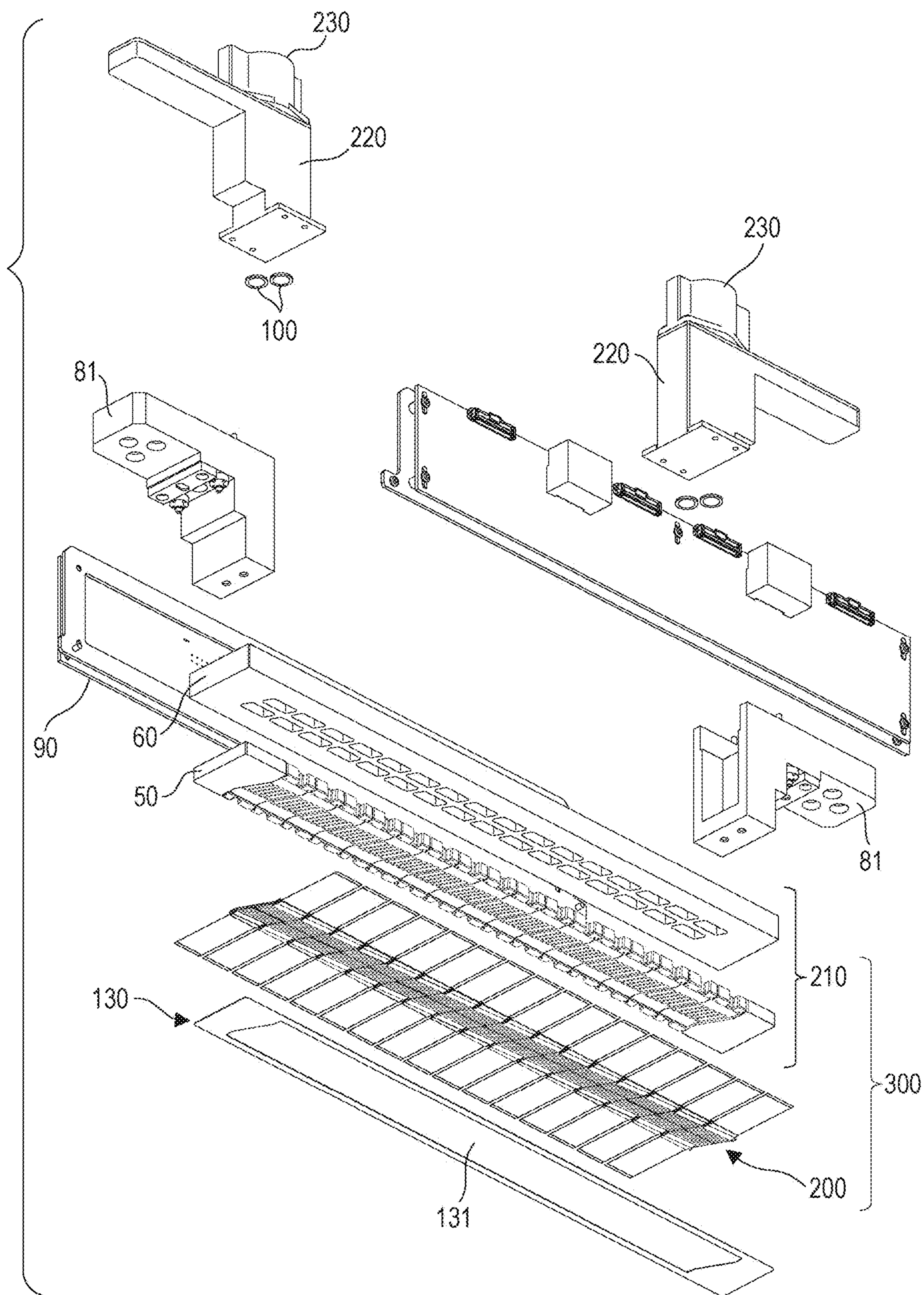
FIG. 15
