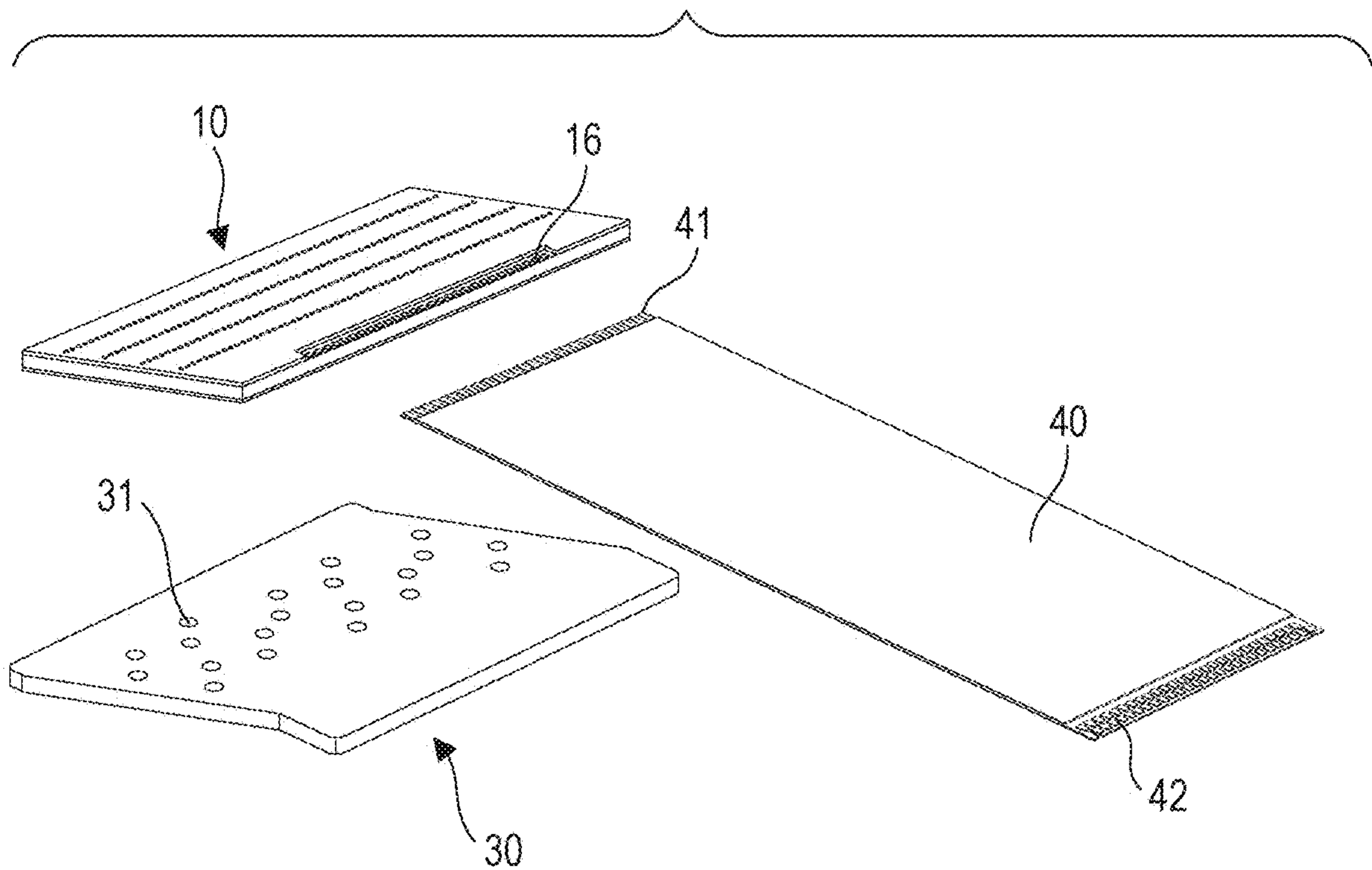
FIG. 9B
