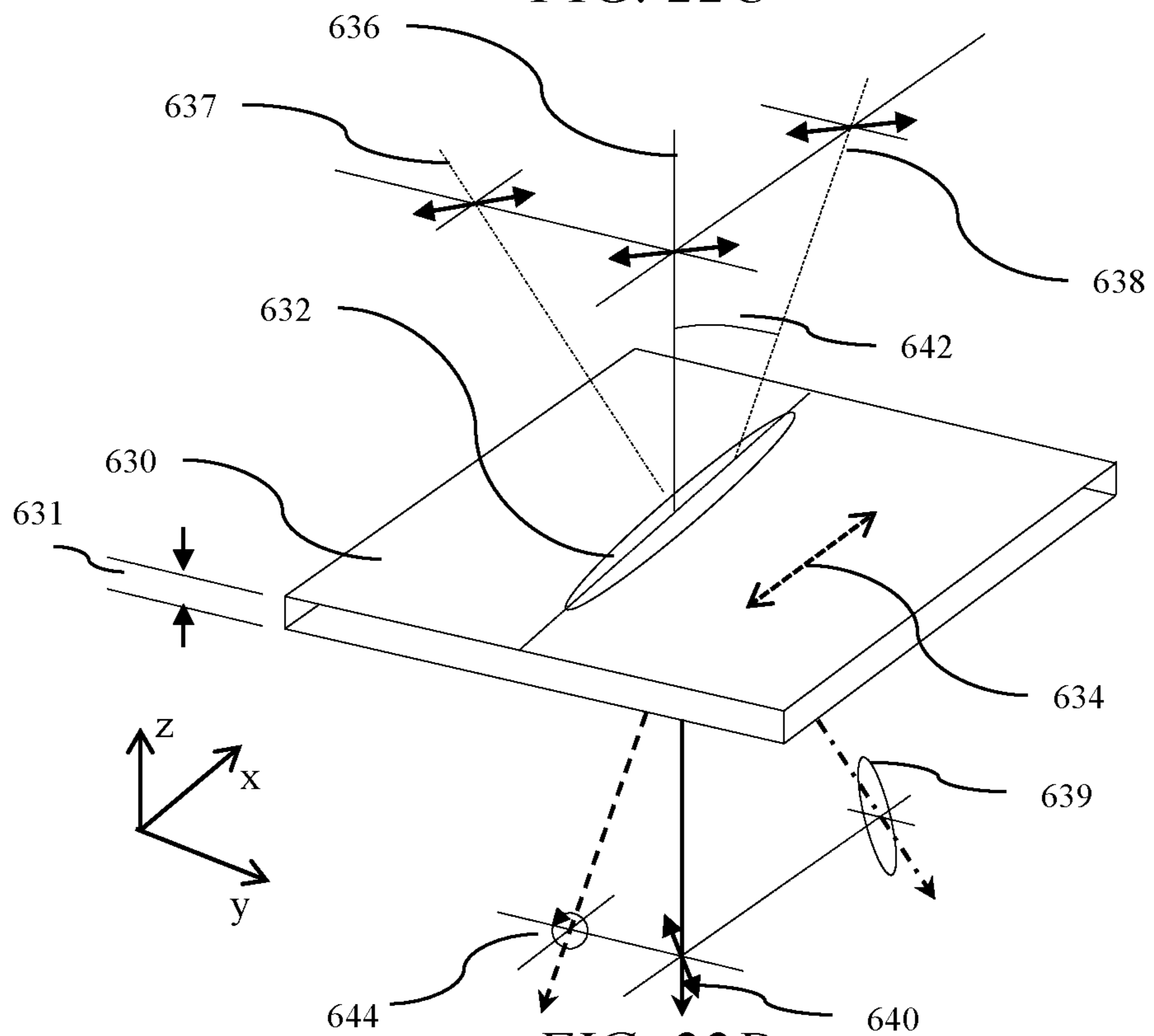
FIG. 22D
