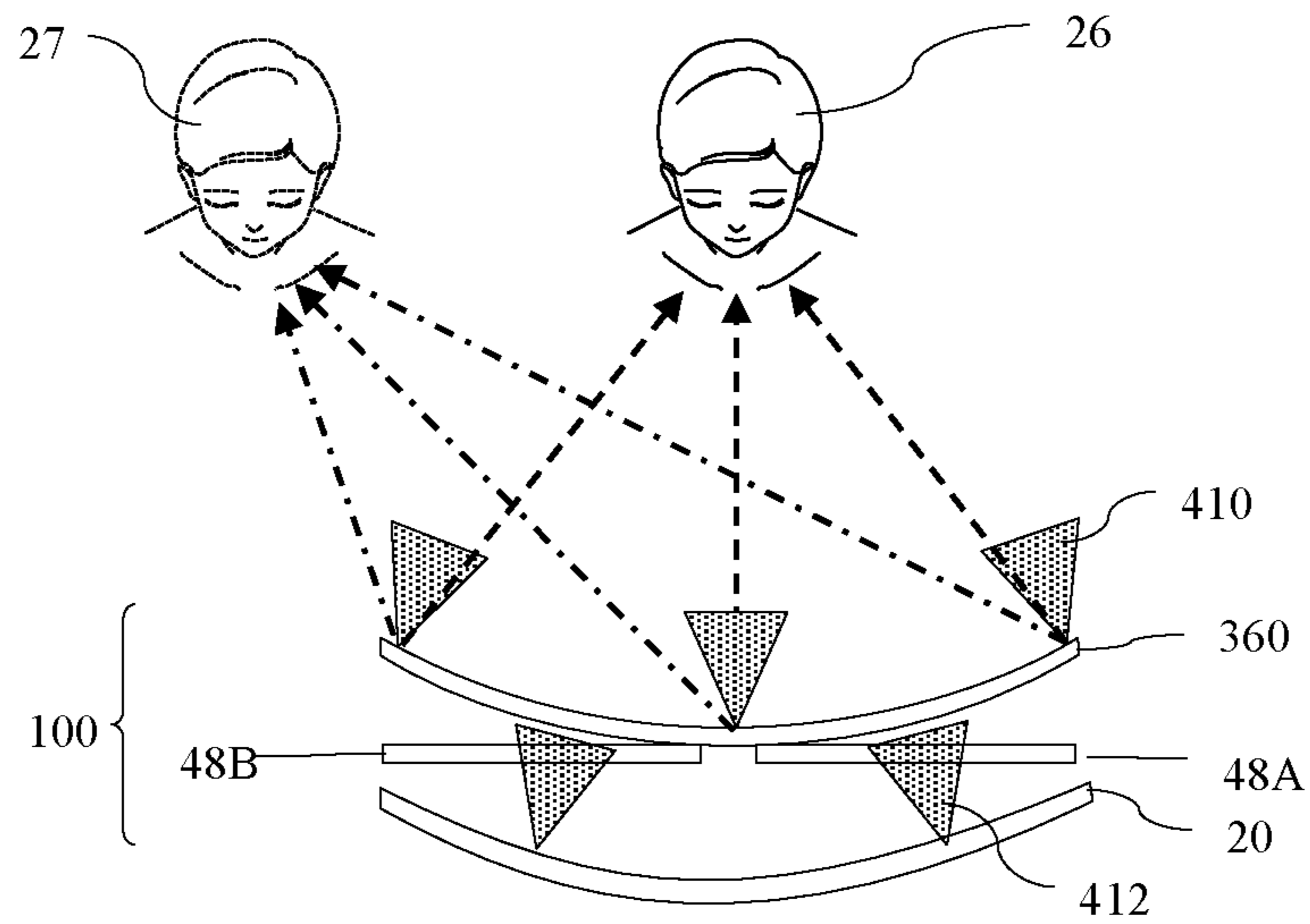
FIG. 10B
