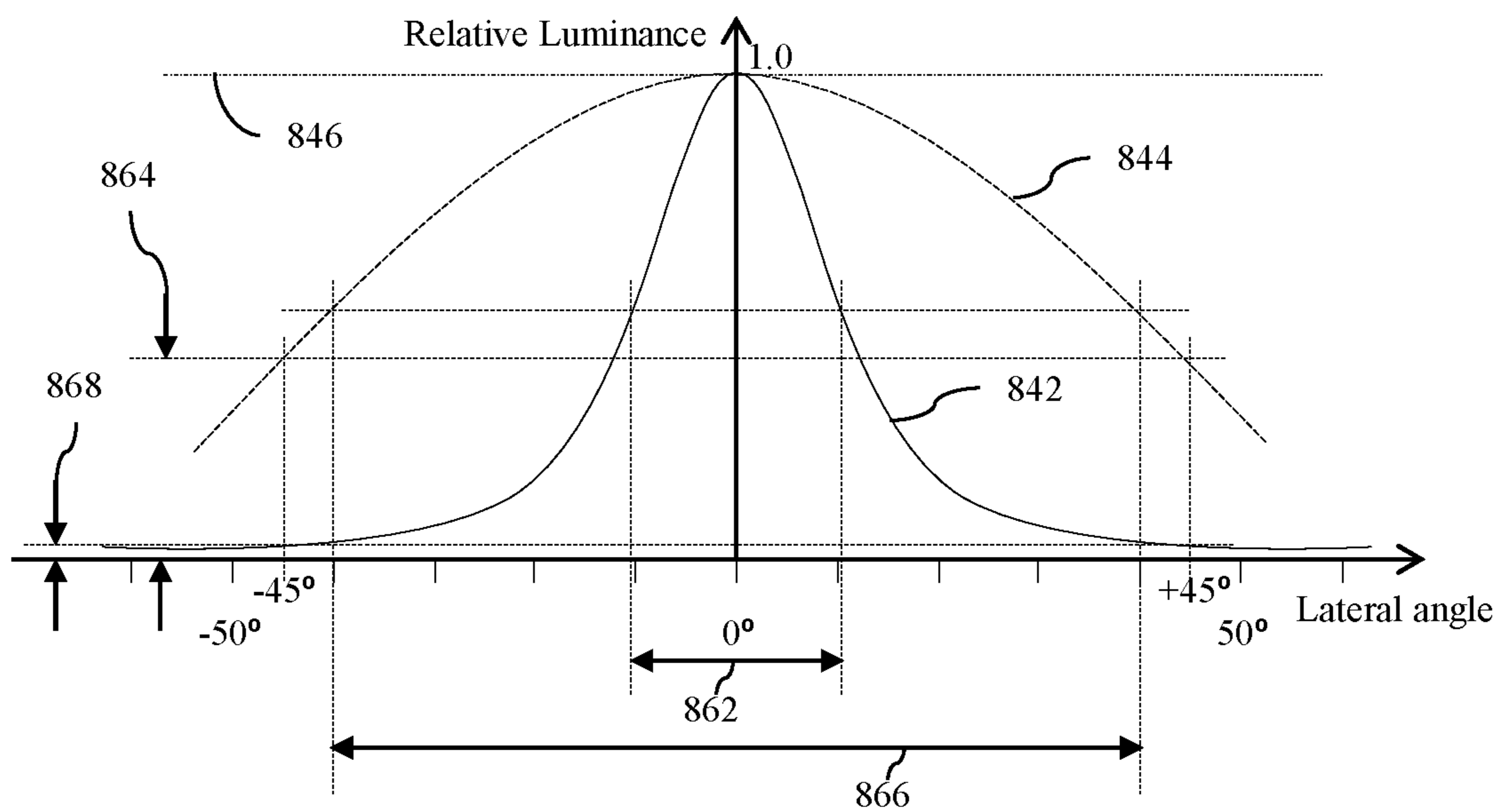
FIG. 19C
