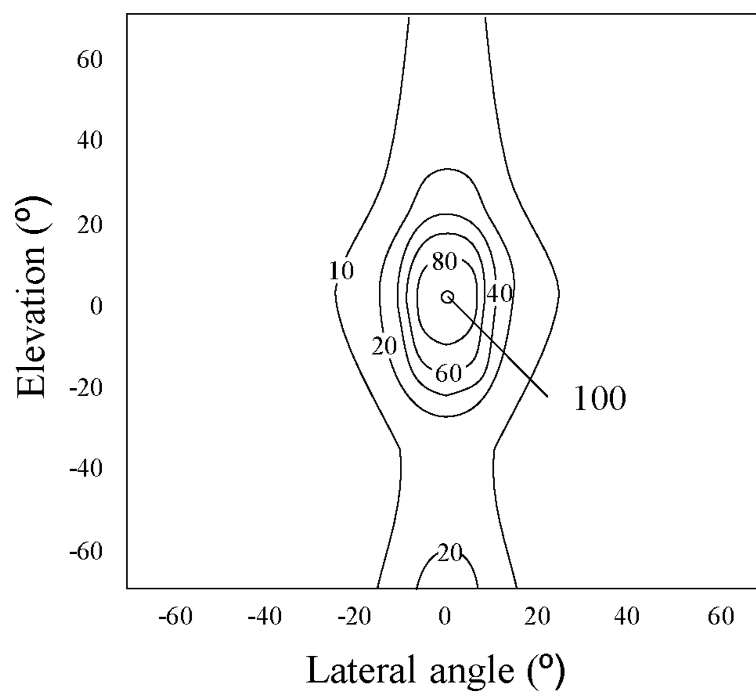
FIG. 19F
