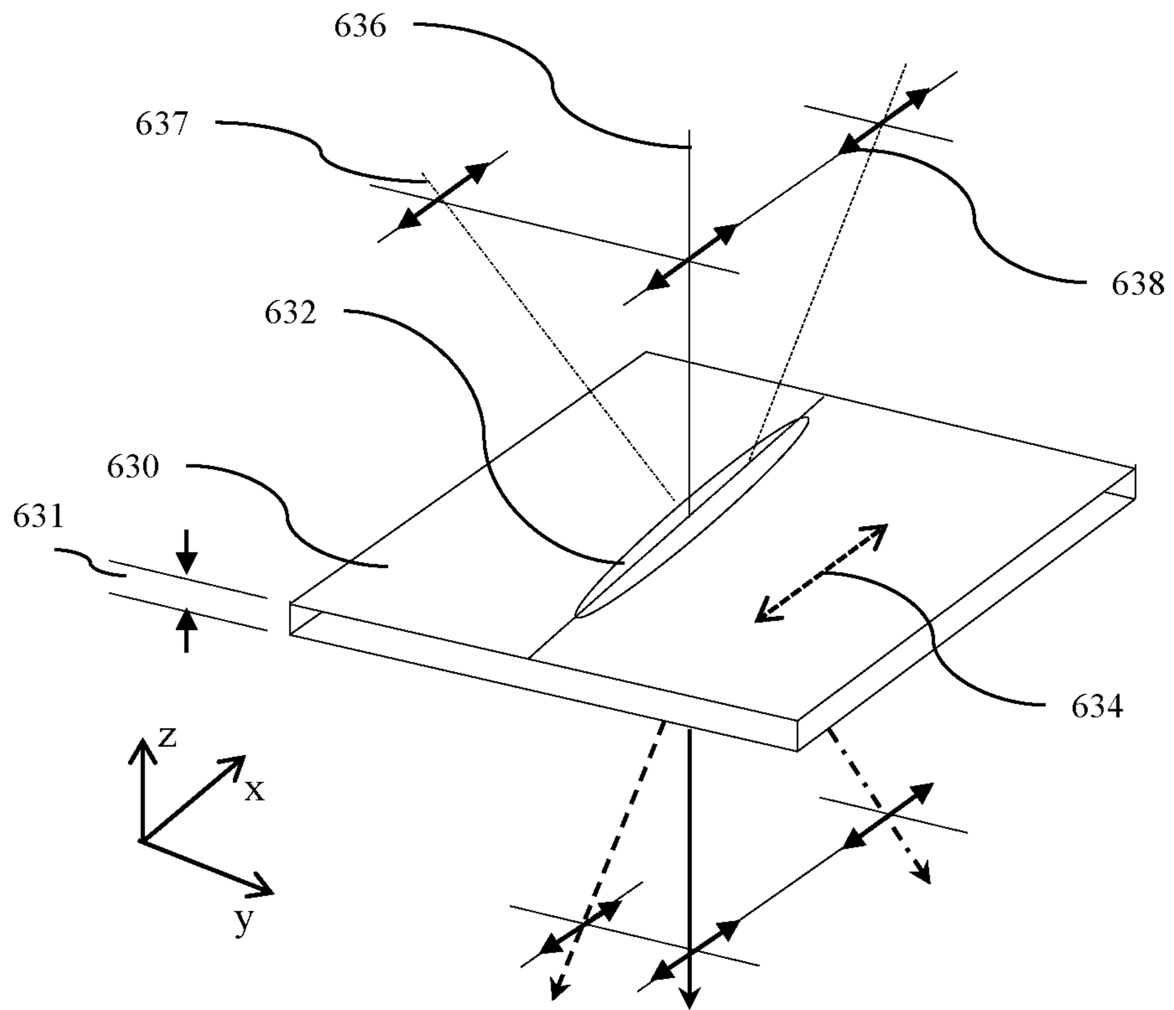
FIG. 22C
