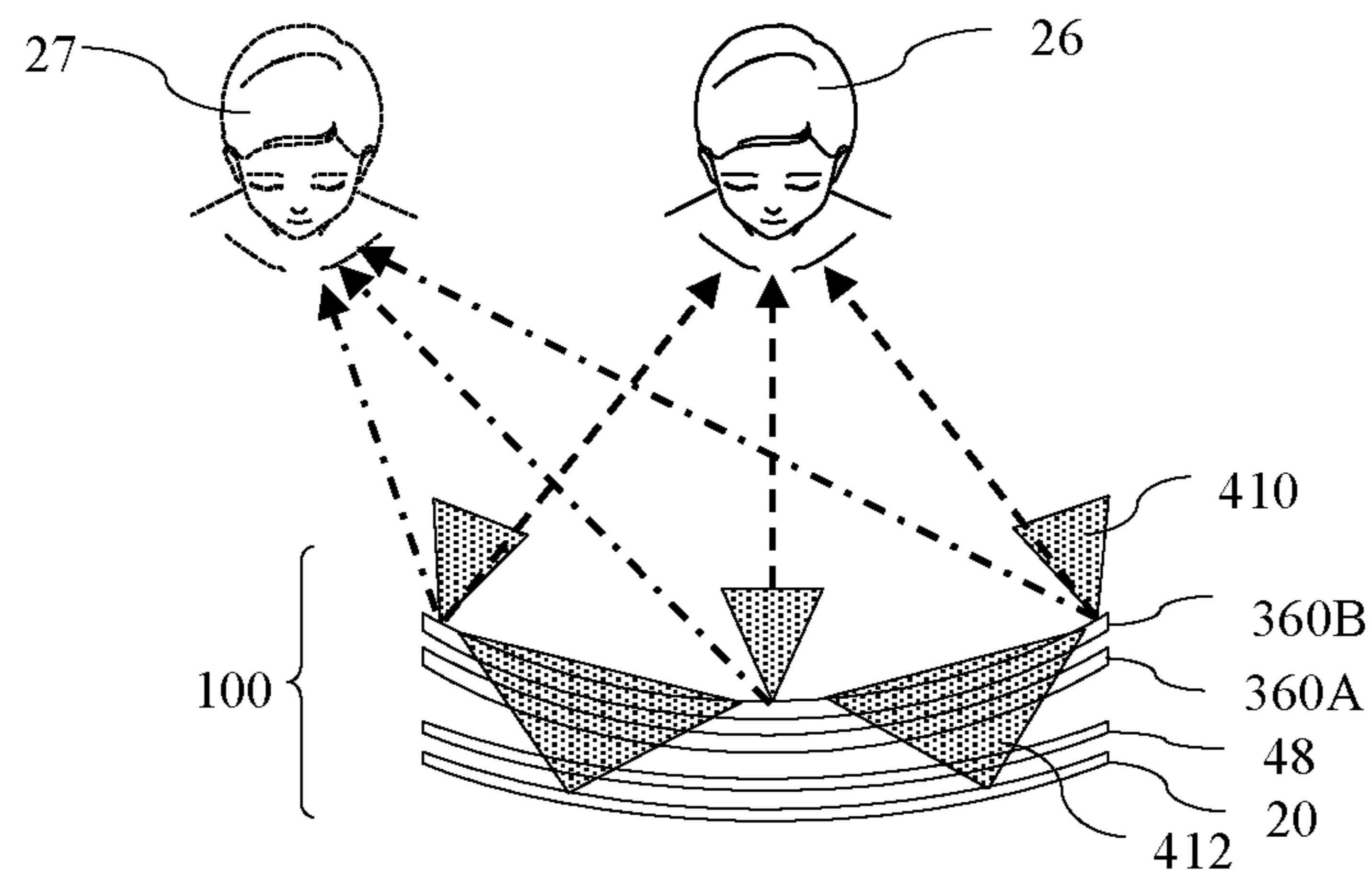
FIG. 11
