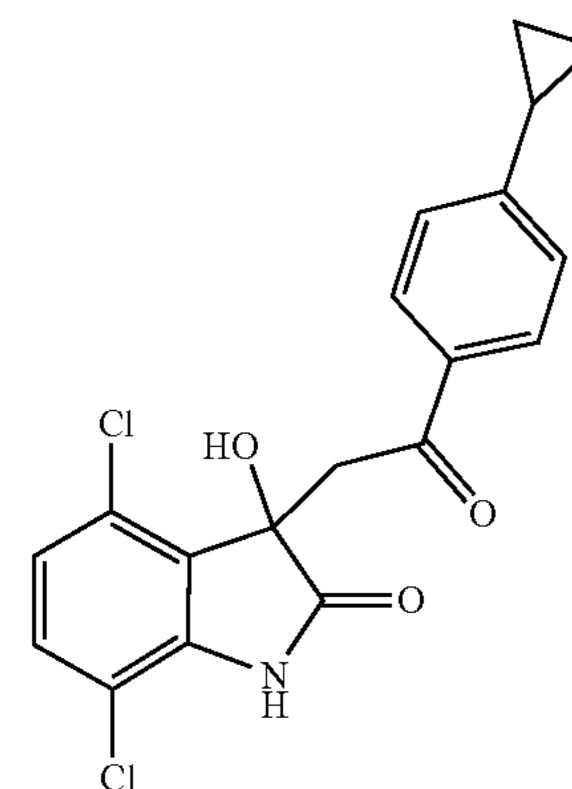
4,7-Dichloro-3-(2-(4-cyclopropylphenyl)-2-oxoethyl)-3-hydroxyindolin-2-one
