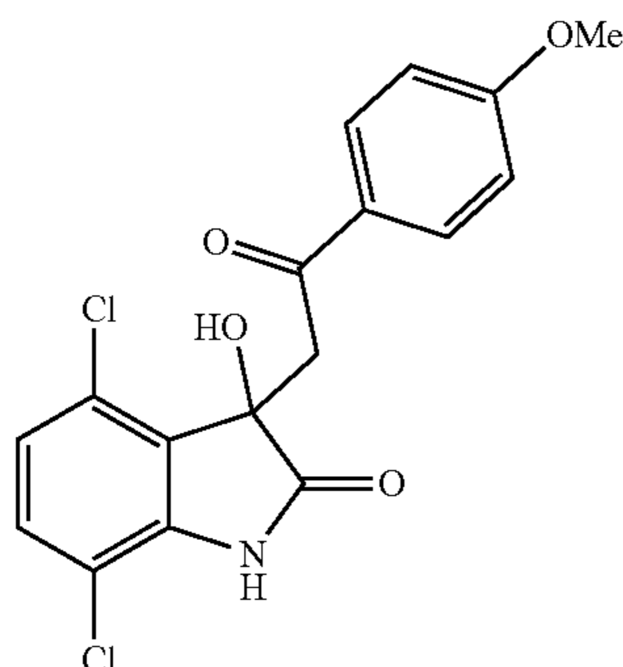
4,7-dichloro-3-hydroxy-3-(2-(4-methoxyphenyl)-2-oxoethyl)indolin-2-one
