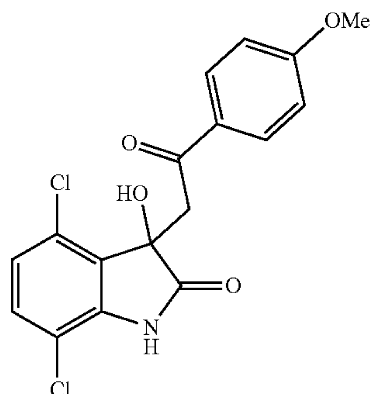
4,7-dichloro-3-hydroxy-3-(2-(4-methoxyphenyl)-2-oxoethyl)indolin-2-one
