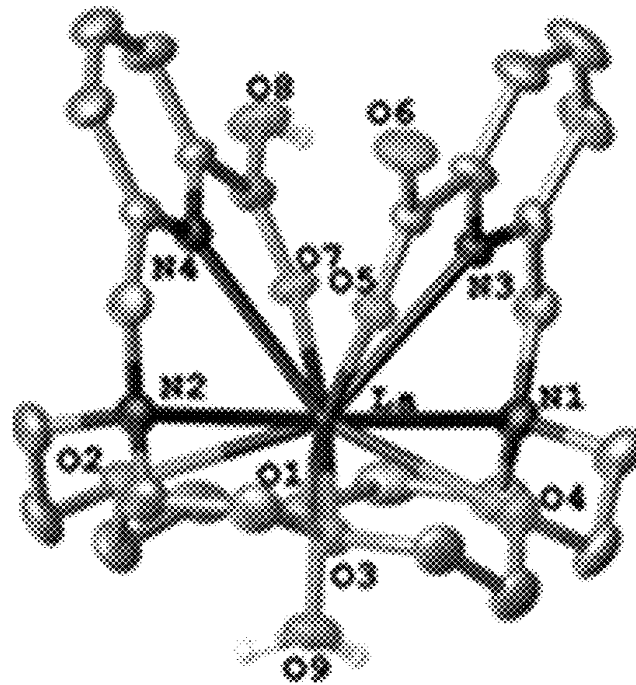
FIG. 1A
