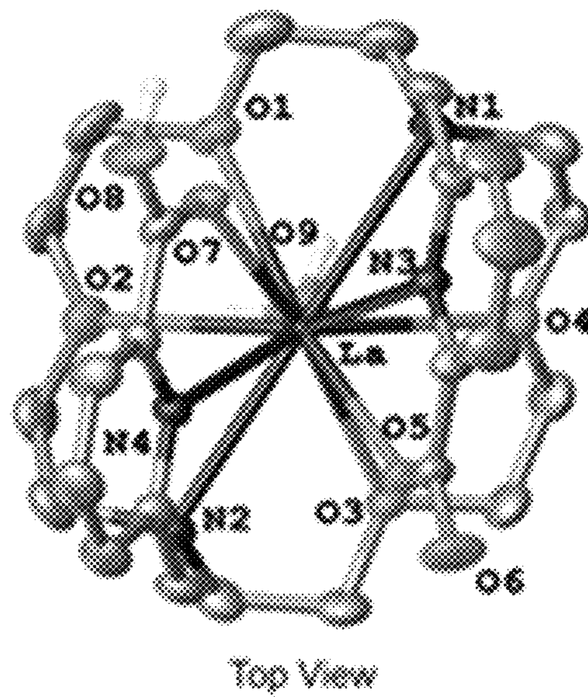
FIG. 1B
