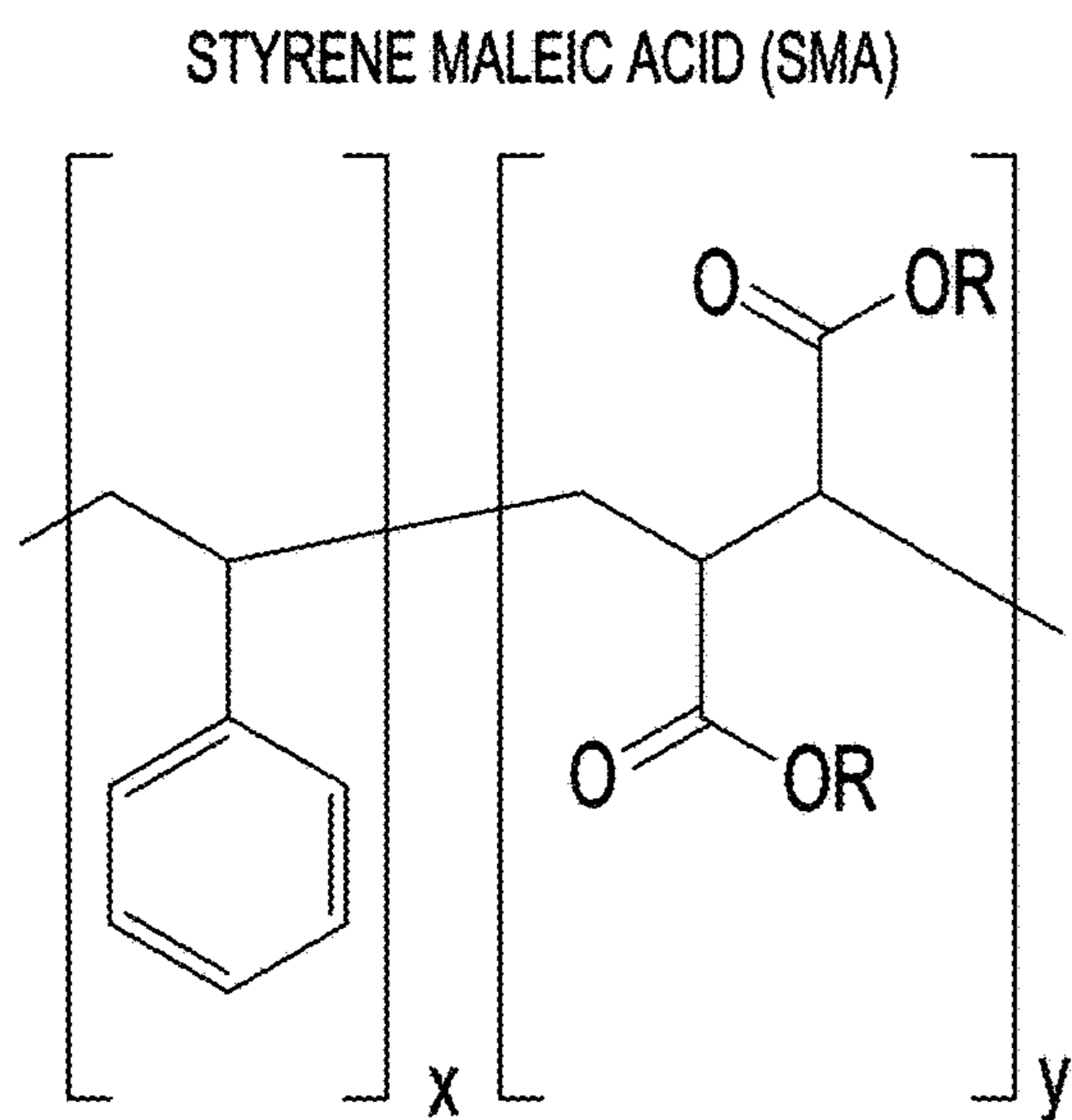
R = H or Na FIG. 15A
