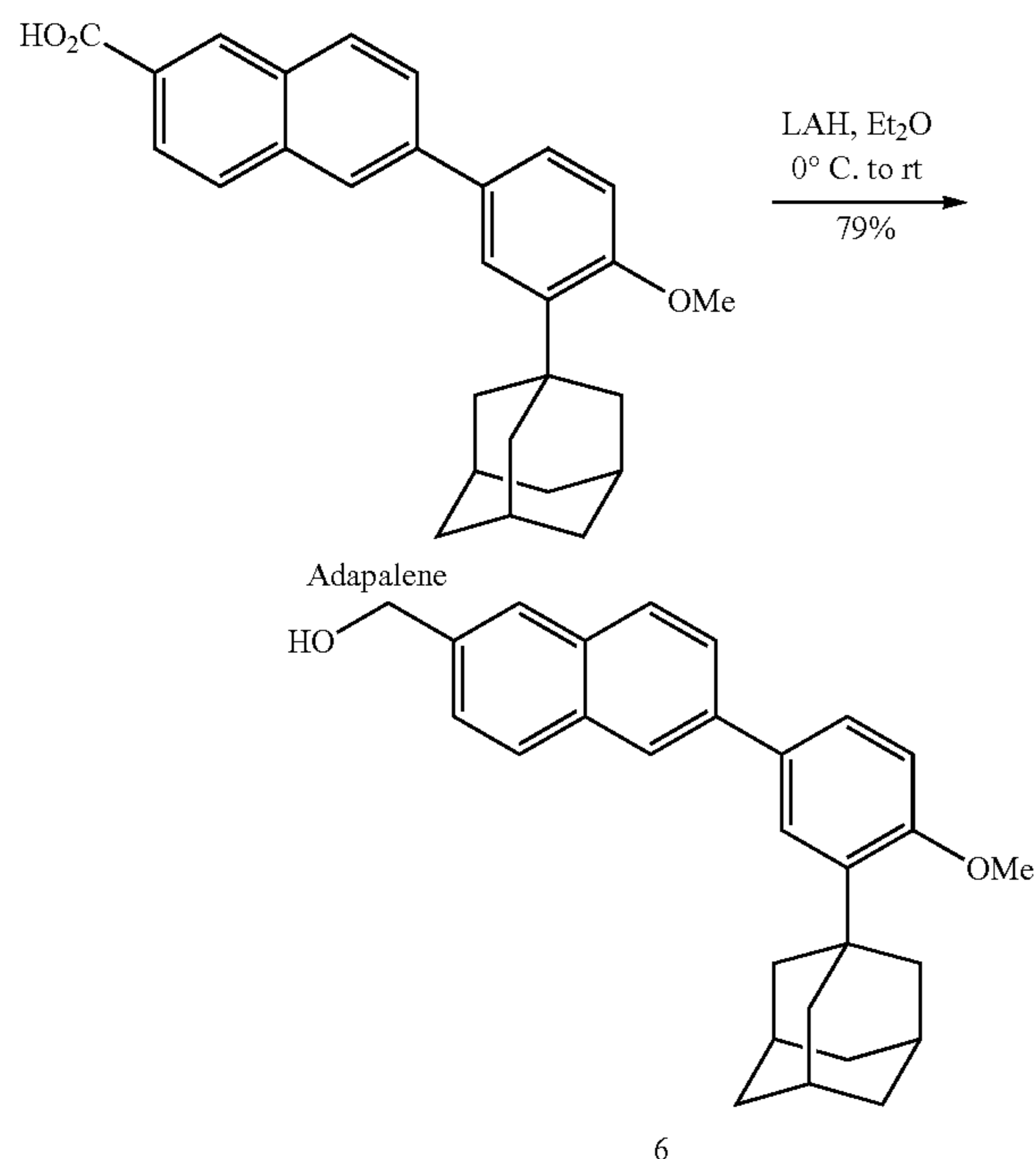
(6-(3-(adamantan-1-yl)-4-methoxyphenyl)naphthalen-2-yl)methanol (6)
